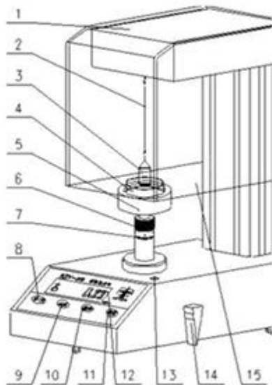
Рисунок 2. Описание устройства Тензиометр марки BZY-3B
