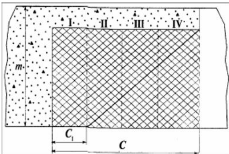
Рисунок 1. Построение защищенной зоны при опережающей обработке рудного тела. I-IV - номер блока, панели, полосы, ленты
