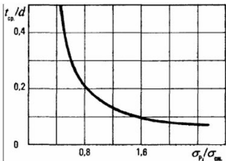
Рисунок 2. Номограмма для определения напряжений в максимуме зоны опорного давления по дискованию керна
