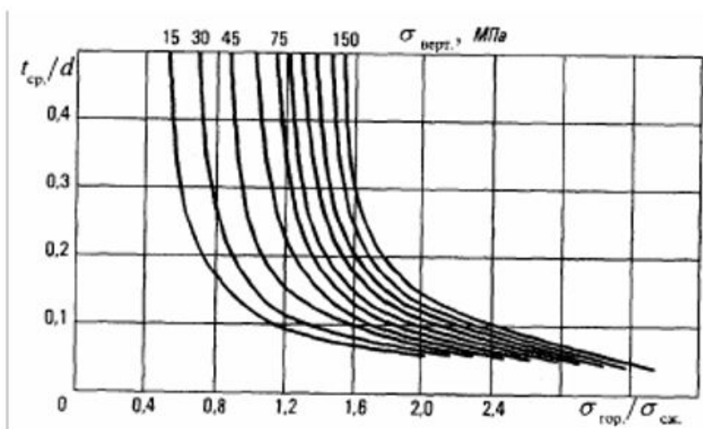
Рисунок 1. Номограмма для оценки напряженного состояния пород \sigma_{гор.}/\sigma_{сж.} по дискованию керна по данным бурения геологоразведочных скважин при различных вертикальных напряжениях, определяемых величиной \gamma H ; где \sigma_{гор.} — горизонтальные напряжения (в мегаПаскалях), t_{ср.} — средняя толщина дисков (в сантиметрах), d — диаметр дисков (в сантиметрах).
