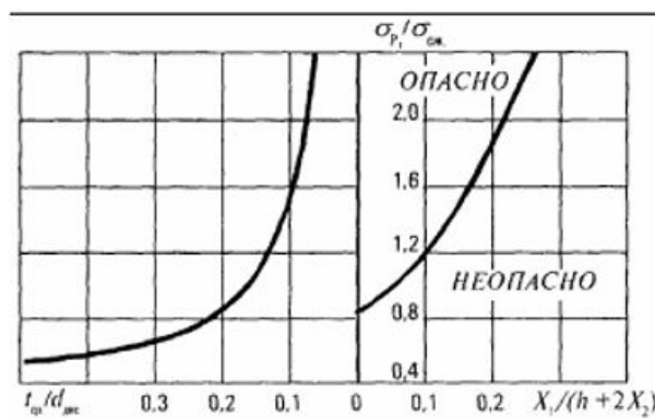
Рисунок 4. Номограмма для определения категории удароопасности участков массива по дискованию керна: h - высота выработки
