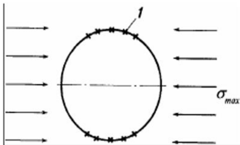
Рисунок 7. Ориентировка участков разрушения пород 1 в сечении выработки относительно наибольших сжимающих напряжений
