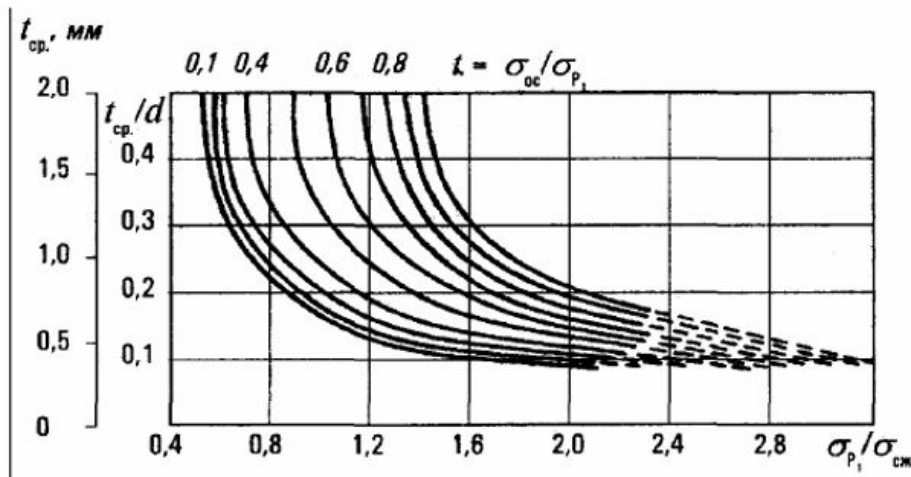
Рисунок 1. Зависимости параметров дискования керна t_{cp}/d_{disc} от уровня напряженности массива \sigma_{p1}/\sigma_{сж} при различных соотношениях между осевыми и радиальными напряжениями \sigma_{ос}/\sigma_{p1} : d_{disc} – диаметр дисков, t_{cp} – средняя толщина дисков
