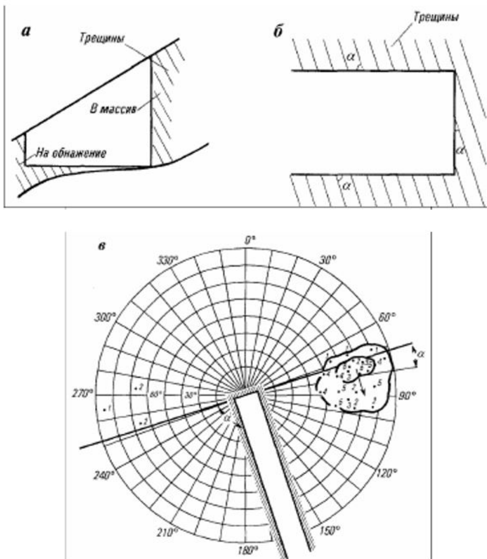
Рисунок 6. Ориентировка трещин относительно обнажения выработки: а - разрез, б - план, в - круговая диаграмма, \alpha - угол встречи трещины с обнажением
