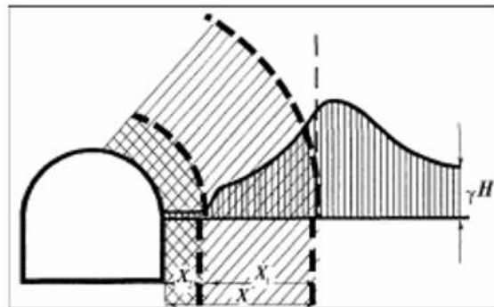
Рисунок 3. Схема, иллюстрирующая положение зоны дискования X_1 , X – расстояние от обнажения до зоны максимума опорного давления; X_1 = X - X_2 ; \gamma – удельный вес породы, H – глубина разработки
