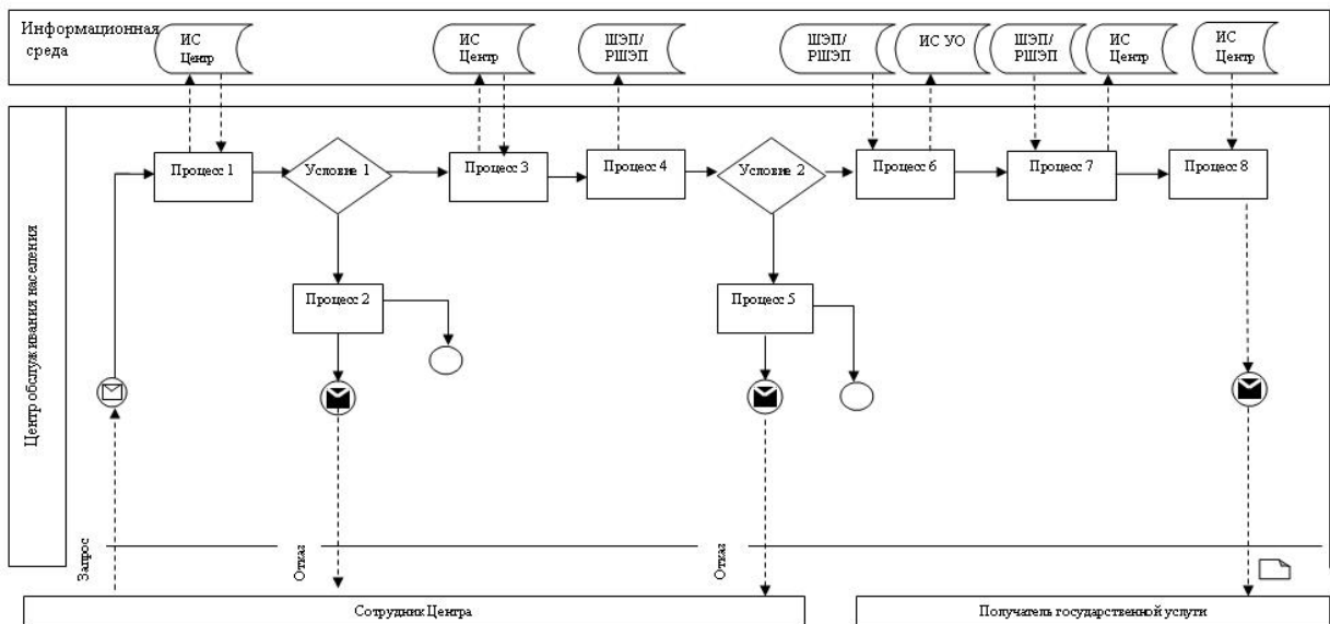
Рисунок 2. Диаграмма функционального взаимодействия при оказании "частично автоматизированной" электронной государственной услуги через ИС Центр
