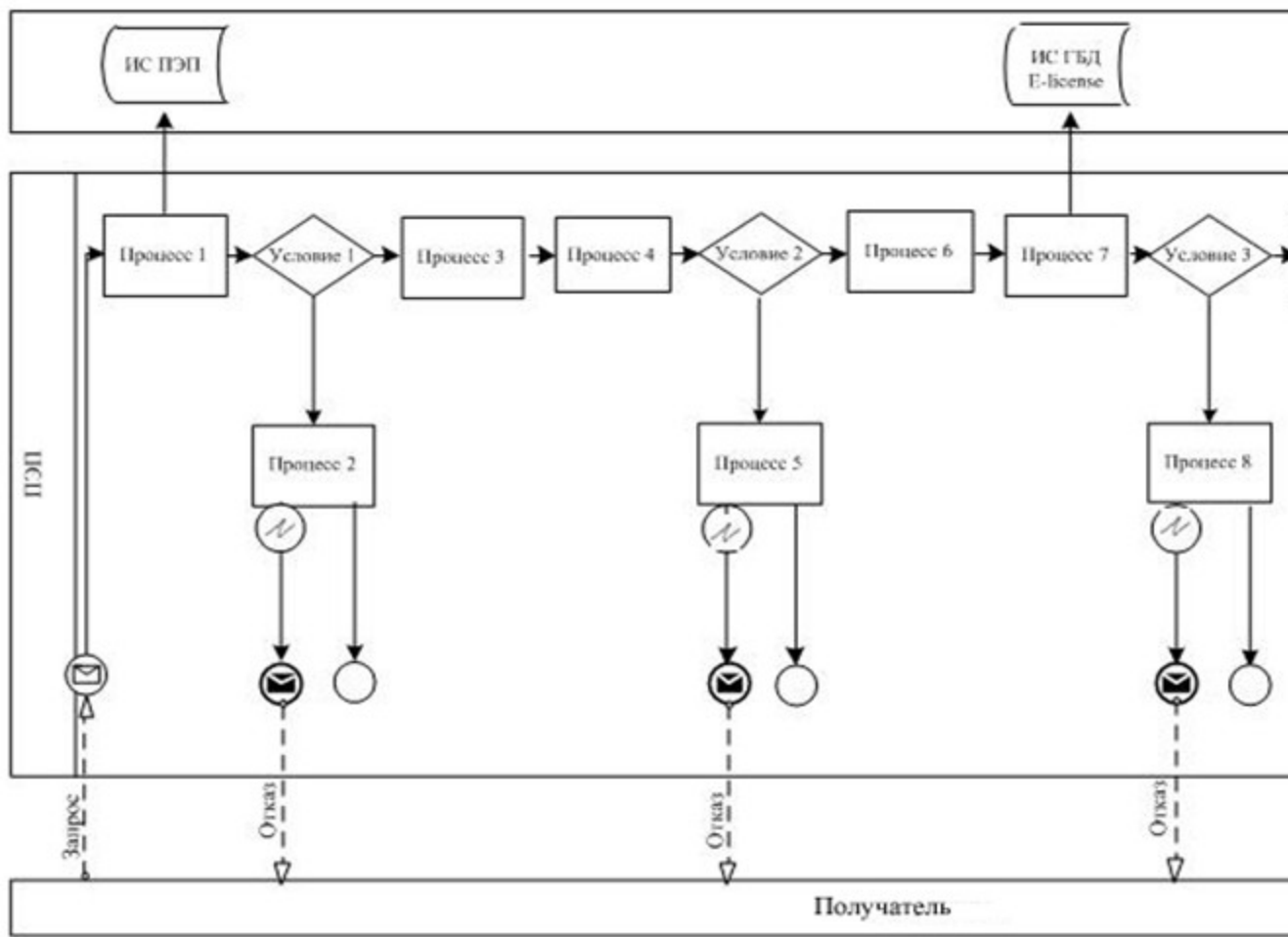
Диаграмма № 2 функционального взаимодействия при оказании электронной государственной услуги через Инспекцию
