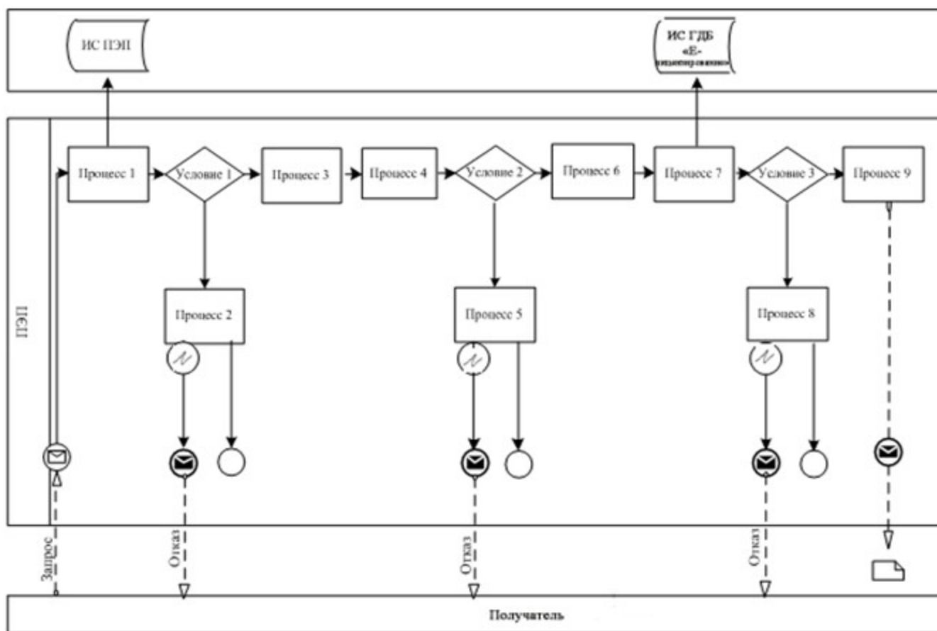
Диаграмма № 2 функционального взаимодействия при оказании электронной государственной услуги через Комитет
