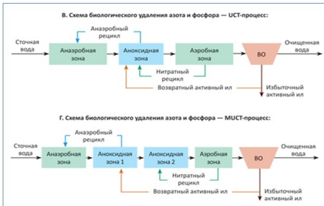
Рисунок 3.2. Примеры традиционных схем биологической очистки сточных вод
