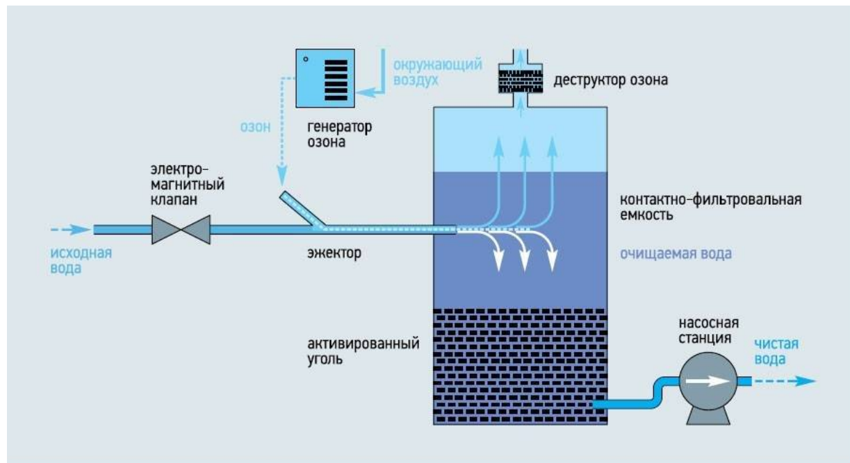
Принципиальная схема озонатора воды
