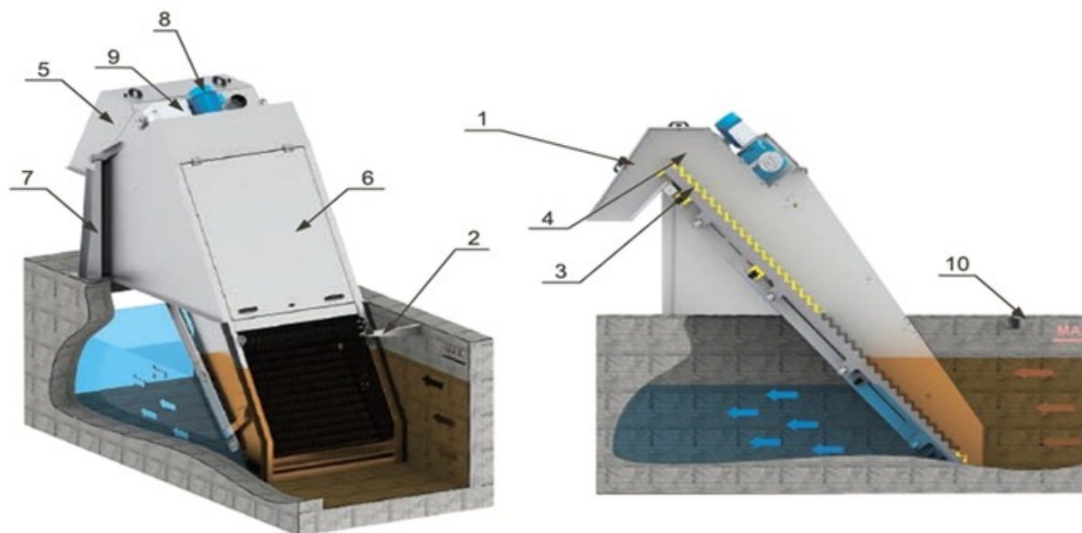
Рисунок 3.3. Решетка ступенчатая
