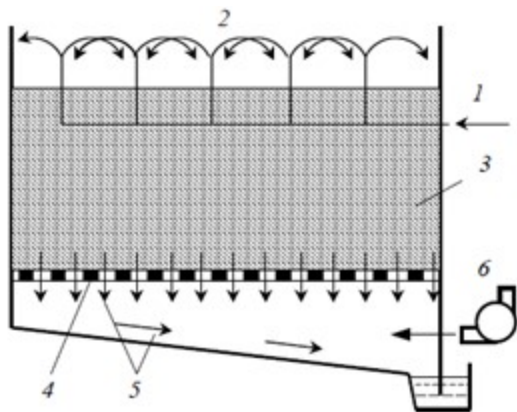
Рисунок 5.11. Схема биофильтра
