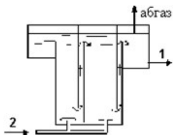
Рисунок 3.9. Схема реактора для озонирования
