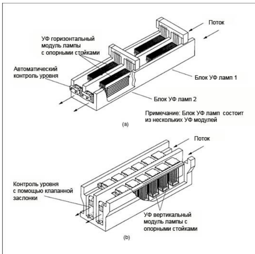
Рисунок 5.17. Схема горизонтально и вертикально расположенных ультрафиолетовых модулей в станциях обеззараживания
