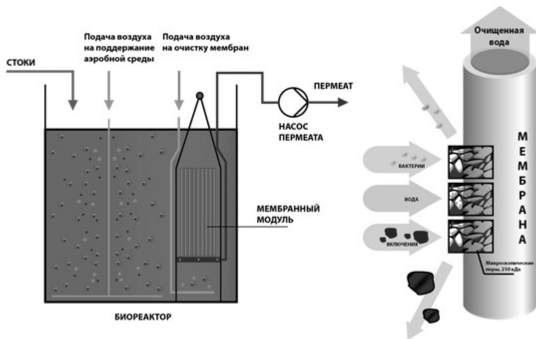
Рисунок 5.12. Принципиальная схема работы MBR
