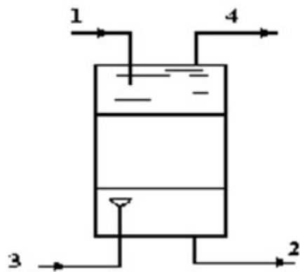
Рисунок 3.10. Экстрактор колонного типа
