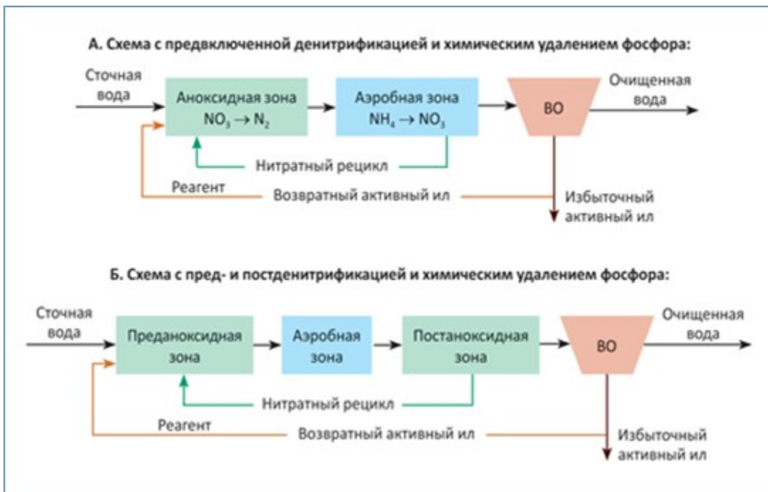
Рисунок 3.1. Типовая схема очистки сточных вод на городских КОС
