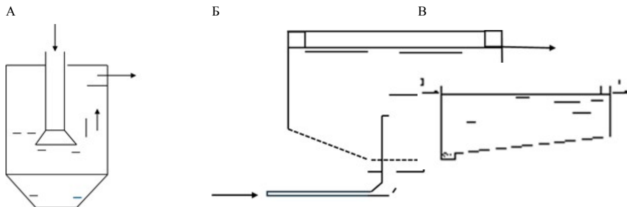
Рисунок 3.4. Отстойники: А – вертикальный, Б – радиальный, В – горизонтальный.
