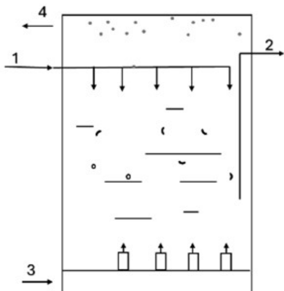
Рисунок 3.5. Напорный флотатор
