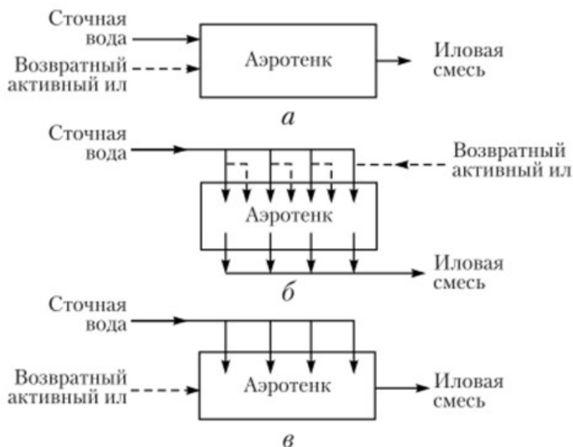
Рисунок 3.11. Схемы аэротенков (а – аэротенк-вытеснитель; б – аэротенк-смеситель ; в – аэротенк промежуточного типа).
