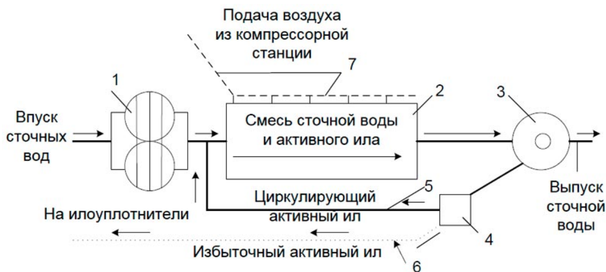
Рисунок 3.13. Схема работы аэротенка:
