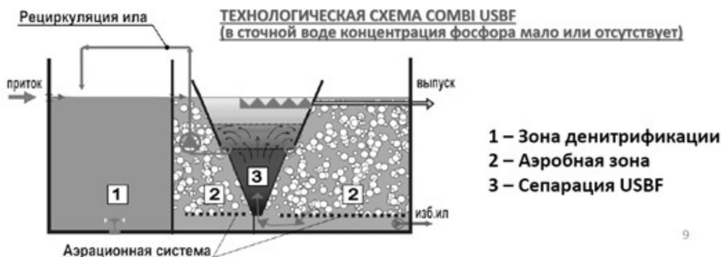
Рисунок 5.15. Технологическая схема USBF (при малых концентрациях фосфора или при его отсутствии)
