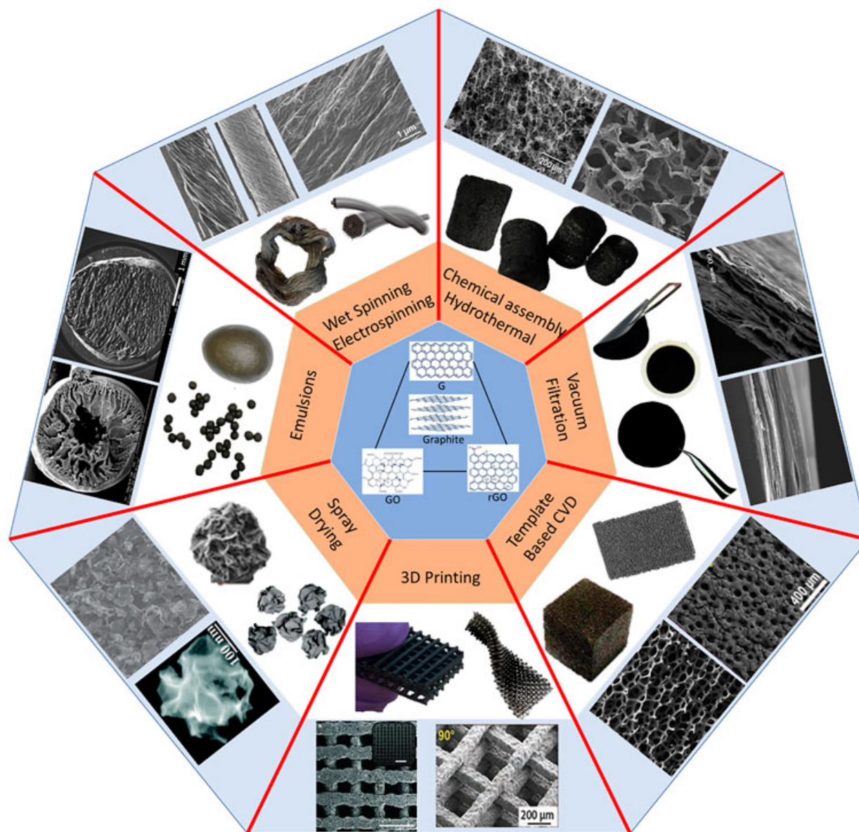
Рисунок 7.1. Самостоятельная сборка 2D-нанолистов на основе графена в 3D-макроструктуре
