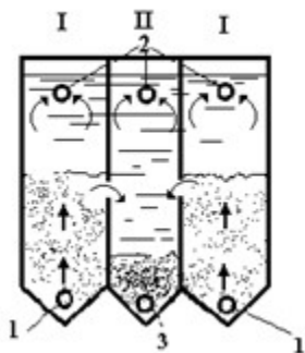
Рисунок 3.6. Осветлитель со взвешенным слоем осадка
