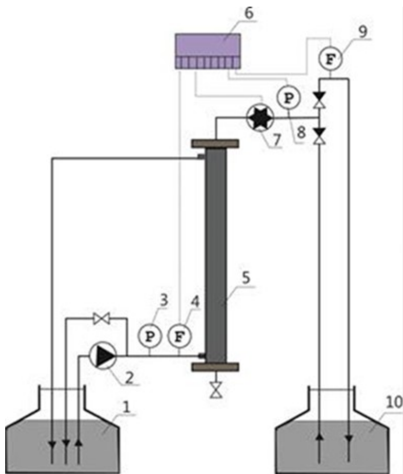
Рисунок 5.19.Схема установки доочистки
