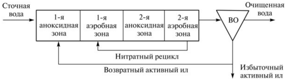
Рисунок 5.6. Технологическая схема Барденфо
