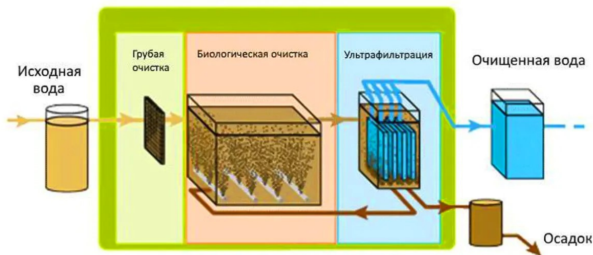
Рисунок 5.20. Технологическая схема очистки сточных вод с блоком ультрафильтрации
