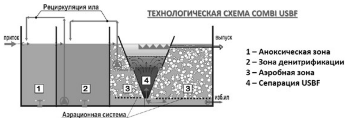
Рисунок 5.14. Технологическая схема USBF
