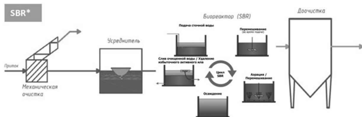
Рисунок 5.16. Технологическая схема реактора циклического действия (SBR)
