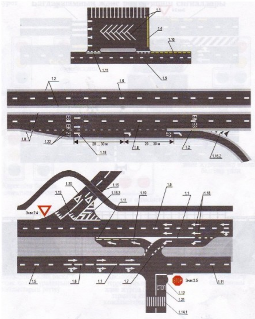
Рис. 3. ДОРОЖНАЯ РАЗМЕТКА ГОРИЗОНТАЛЬНАЯ РАЗМЕТКА
