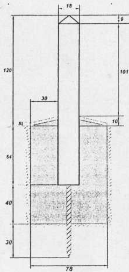
ВИД СБОКУ
