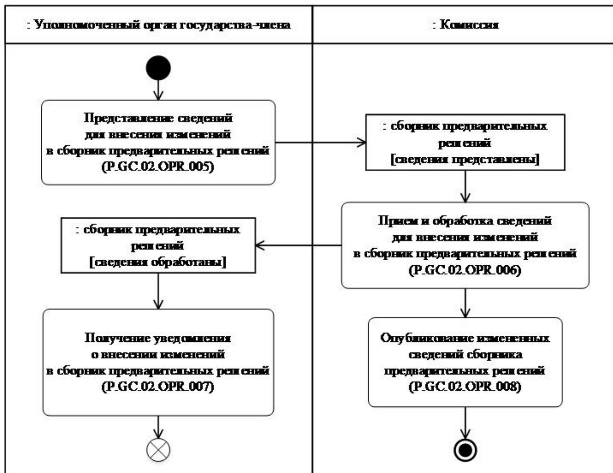
Рис. 5. Схема выполнения процедуры "Изменение сведений, содержащихся в сборнике предварительных решений" (P.GC.02.PRC.002)
