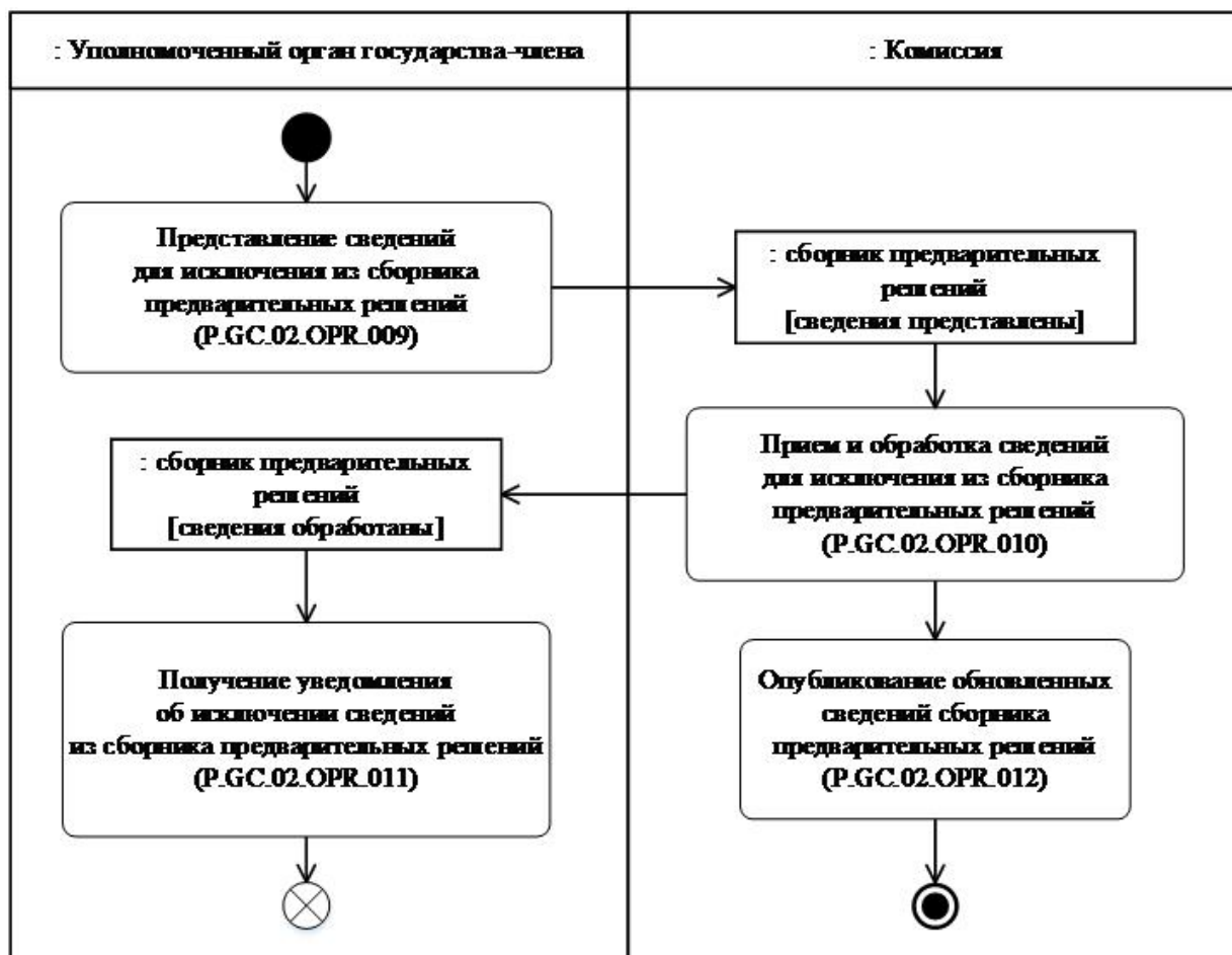
Рис. 6. Схема выполнения процедуры "Исключение сведений, содержащихся в сборнике предварительных решений" (P.GC.02.PRC.003)
