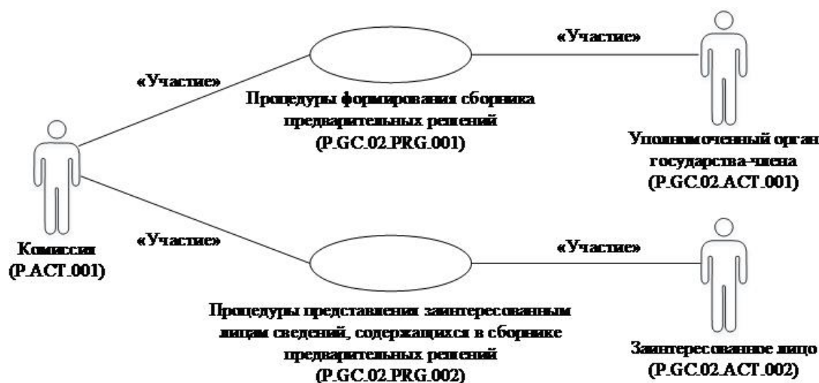
Рис. 1. Структура общего процесса
