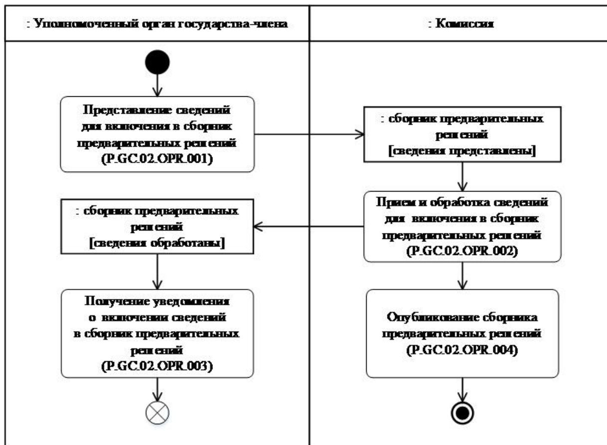
Рис. 4. Схема выполнения процедуры "Включение сведений в сборник предварительных решений" (P.GC.02.PRC.001)
