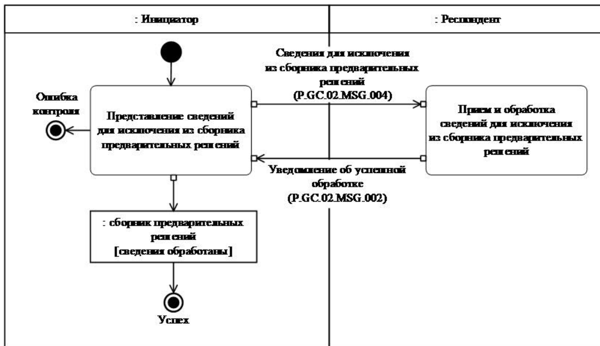
Рис. 5. Схема выполнения транзакции общего процесса "Представление сведений для исключения из сборника предварительных решений" (P.GC.02.TRN.003)
