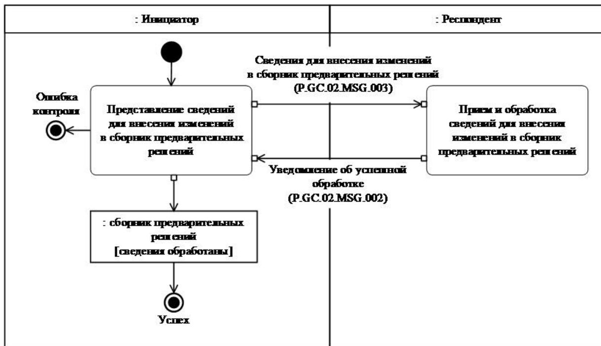
Рис. 4. Схема выполнения транзакции общего процесса "Представление сведений для внесения изменений в сборник предварительных решений" (P.GC.02.TRN.002)
