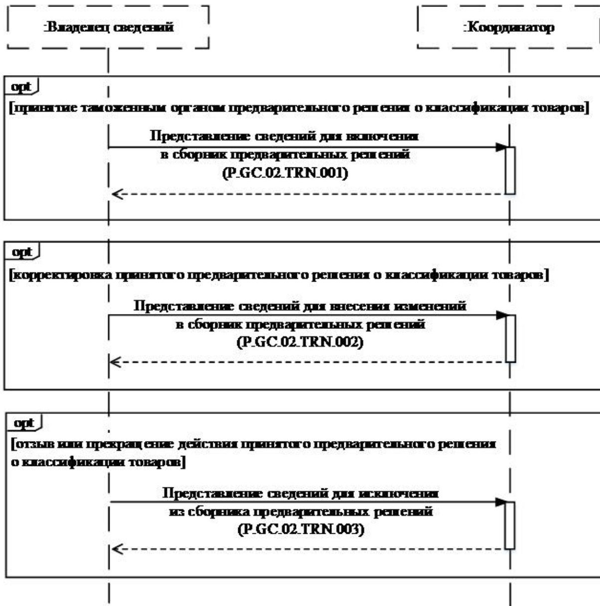
Рис. 2. Схема выполнения транзакций общего процесса при формировании сборника предварительных решений
