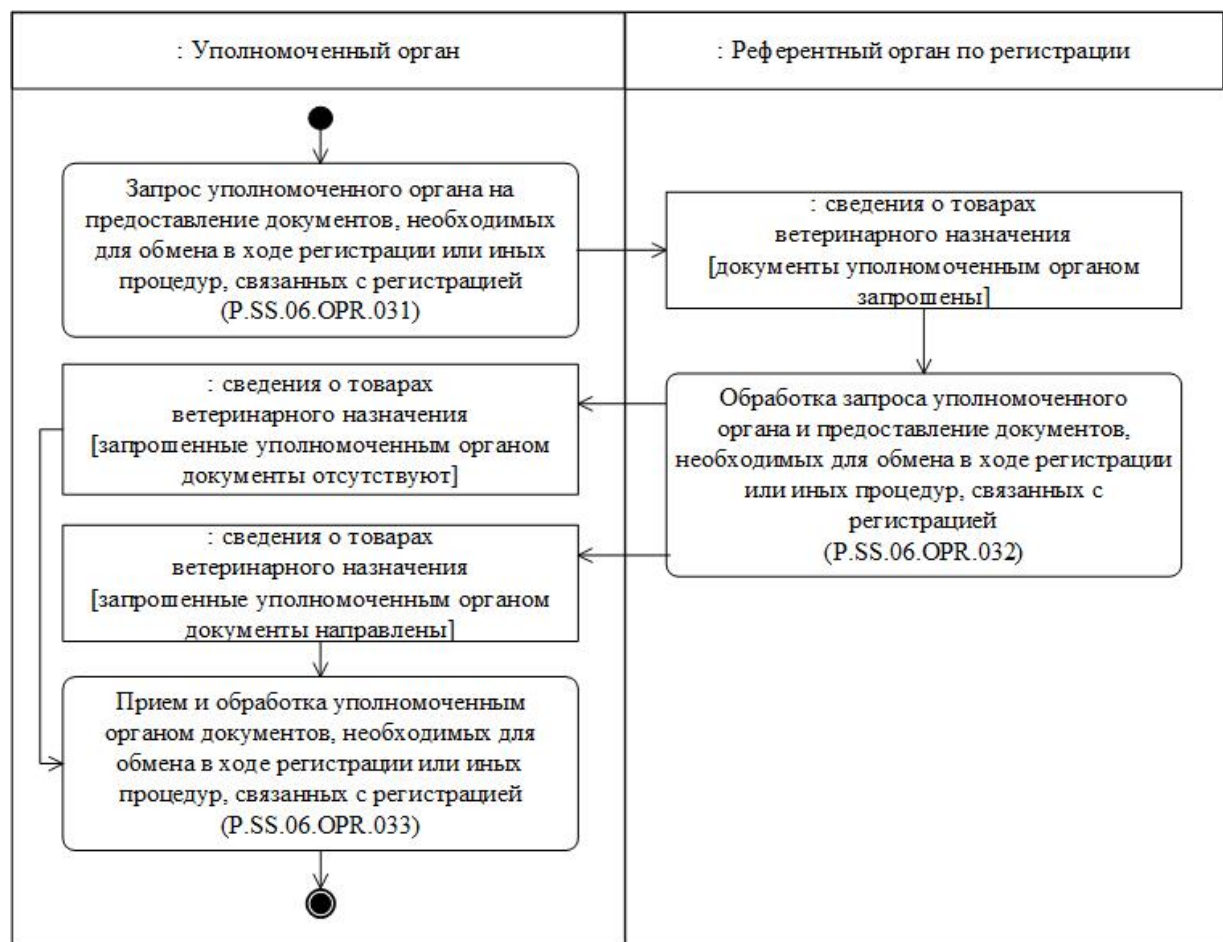
Рис. 18. Схема выполнения процедуры "Предоставление в уполномоченный орган документов, необходимых для обмена в ходе регистрации или иных процедур, связанных с регистрацией по запросу" (P.SS.06.PRC.012)
