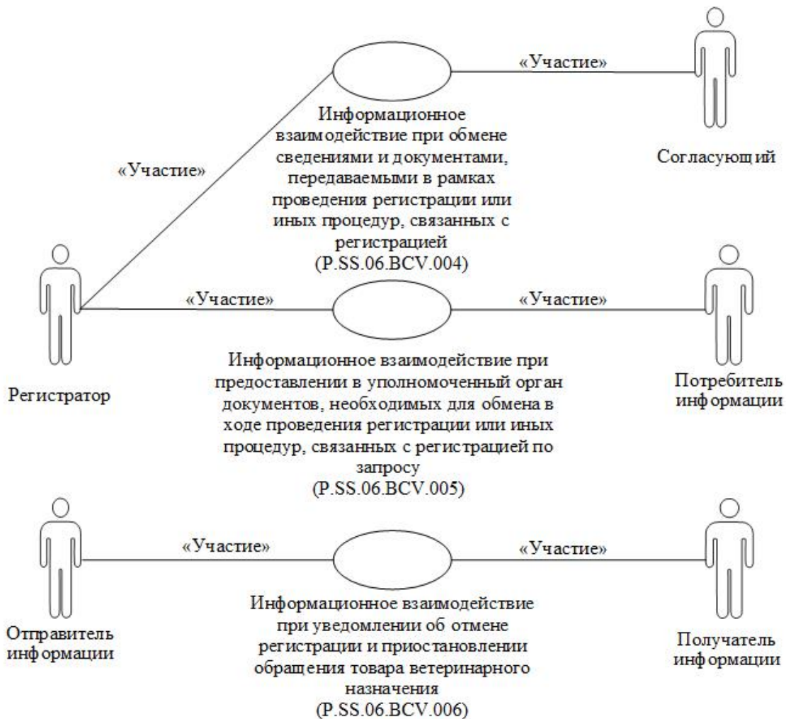
Рис. 1. Структура информационного взаимодействия между уполномоченными органами государств – членами Евразийского экономического союза
