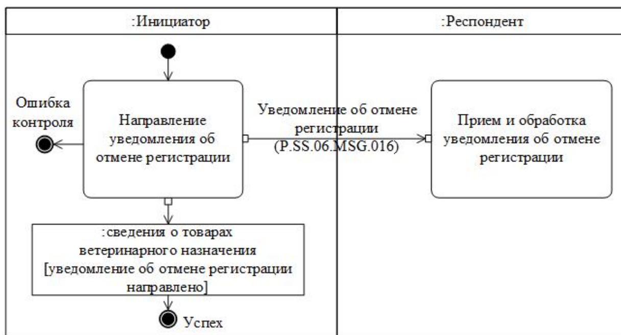
Рис. 10. Схема выполнения транзакции общего процесса "Уведомление об отмене регистрации" (P.SS.06.TRN.011)
