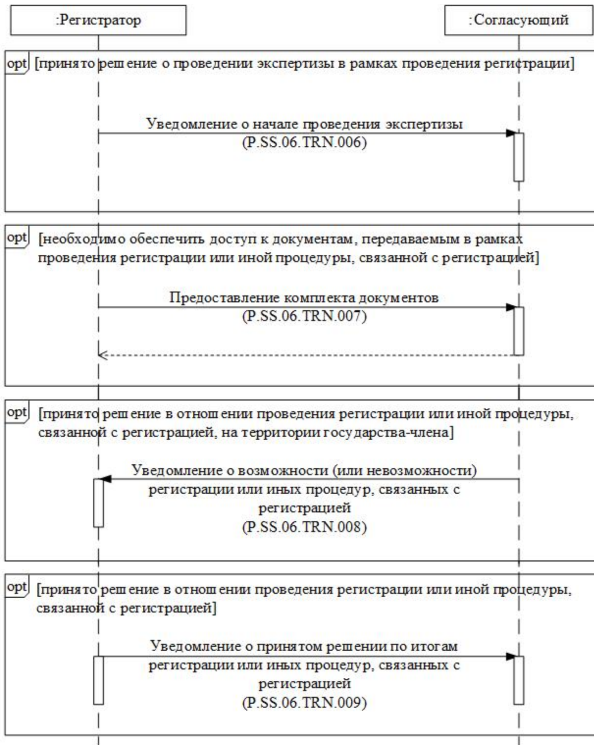
Рис. 2. Схема выполнения транзакций общего процесса при обмене сведениями и документами, передаваемыми в рамках проведения регистрации или иных процедур, связанных с регистрацией
