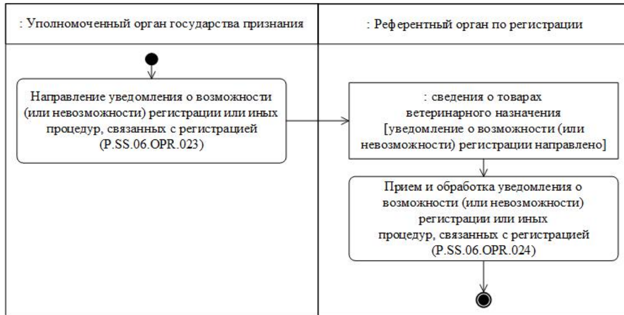
Рис. 14. Схема выполнения процедуры "Уведомление о возможности (или невозможности) регистрации или иных процедур, связанных с регистрацией" (P.SS.06.PRC.008)
