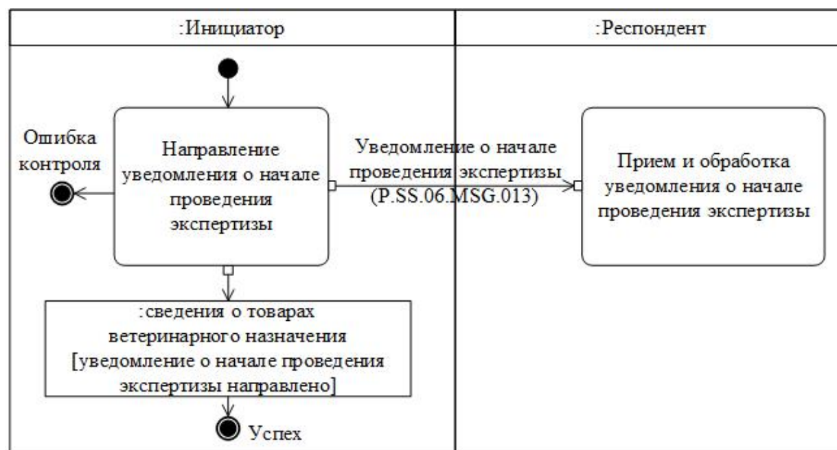
Рис. 5. Схема выполнения транзакции общего процесса "Уведомление о начале проведения экспертизы" (P.SS.06.TRN.006)
