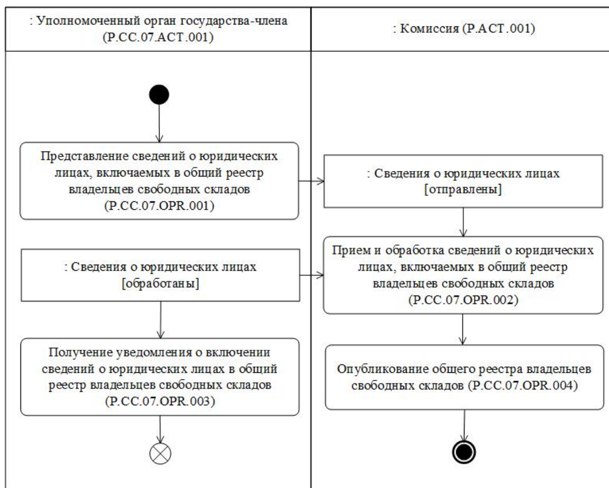
Рис. 5. Схема выполнения процедуры "Включение сведений о юридических лицах в общий реестр владельцев свободных складов" (P.CC.07.PRC.001)
