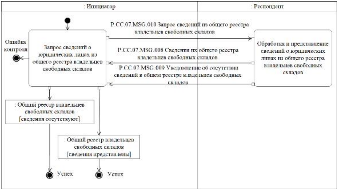
Рис. 8. Схема выполнения транзакции общего процесса "Получение сведений о юридических лицах из общего реестра владельцев свободных складов" (P. CC.07.TRN.005)
