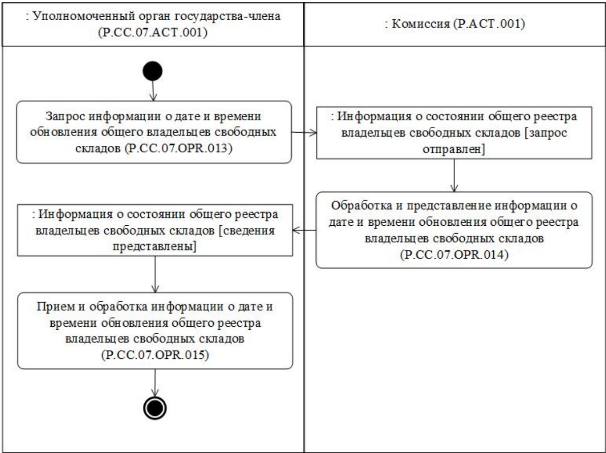
Рис. 9. Схема выполнения процедуры "Получение информации о дате и времени обновления общего реестра владельцев свободных складов" (P.CC.07.PRC.004)
