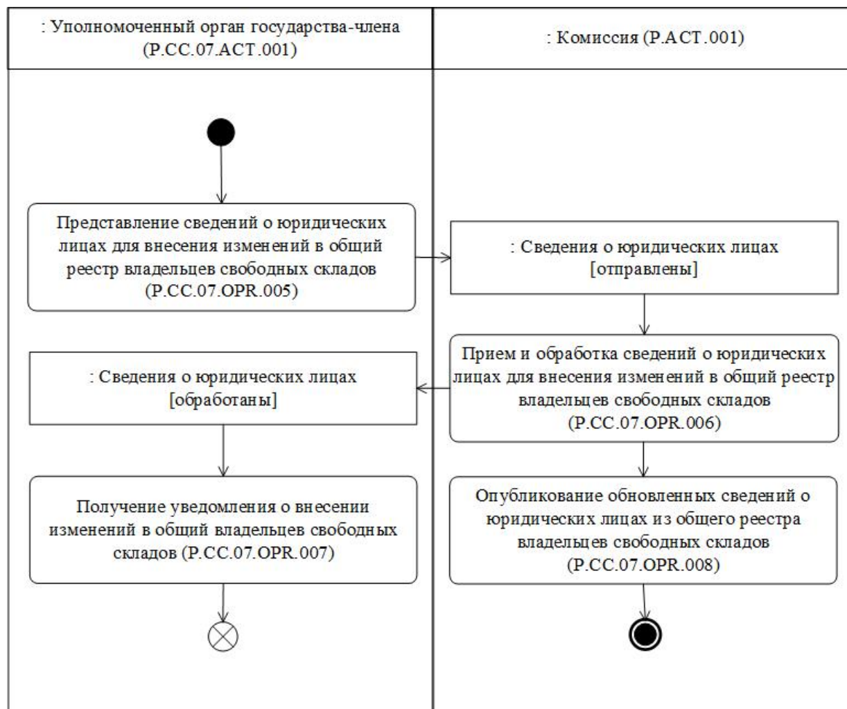
Рис. 6. Схема выполнения процедуры "Изменение сведений о юридических лицах, содержащихся в общем реестре владельцев свободных складов" (Р.СС.07.ПРС.002)
