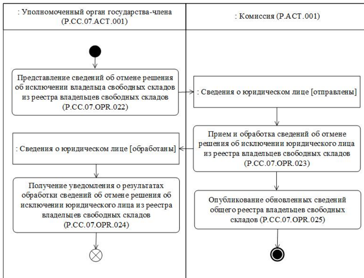
Рис. 8. Схема выполнения процедуры "Отмена решения об исключении юридического лица из общего реестра владельцев свободных складов" (P.CC.07.PRC.008)
