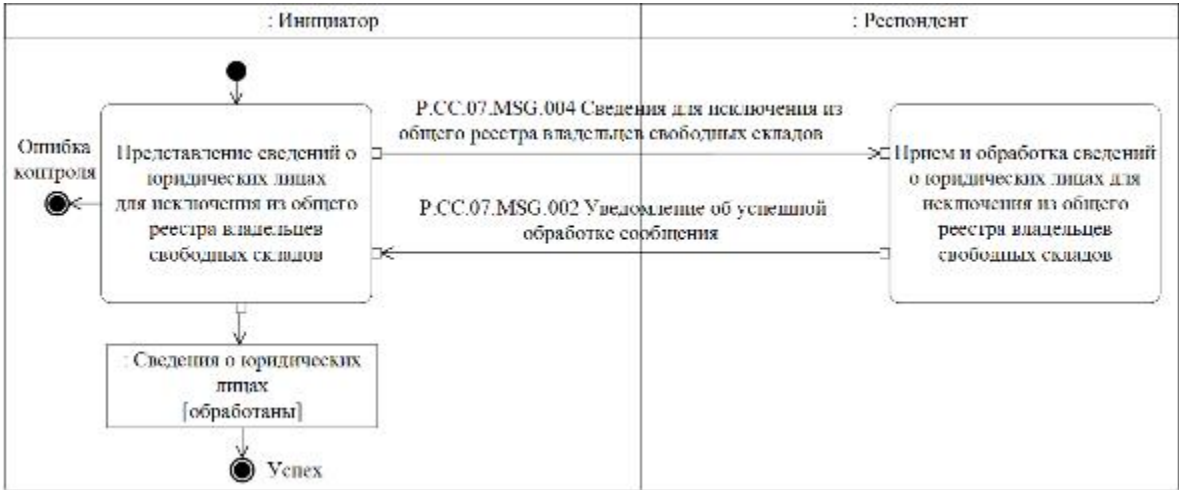
Рис. 6. Схема выполнения транзакции общего процесса "Исключение сведений о юридических лицах из общего реестра владельцев свободных складов" (P.CC.07.TRN.003)
