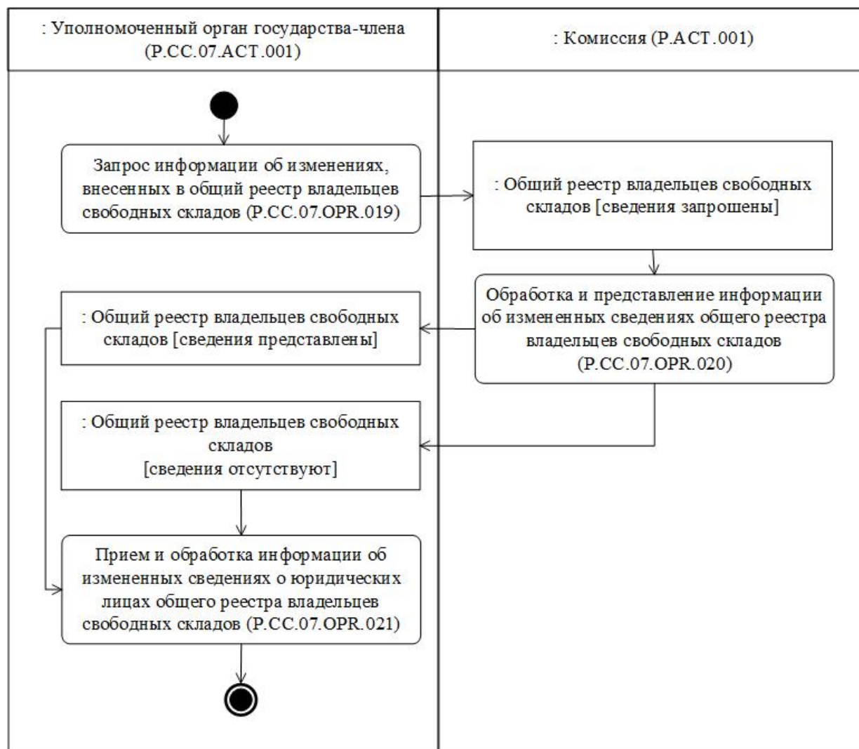
Рис. 11. Схема выполнения процедуры "Получение информации об изменениях, внесенных в общий реестр владельцев свободных складов" (P.CC.07.PRC.006)
