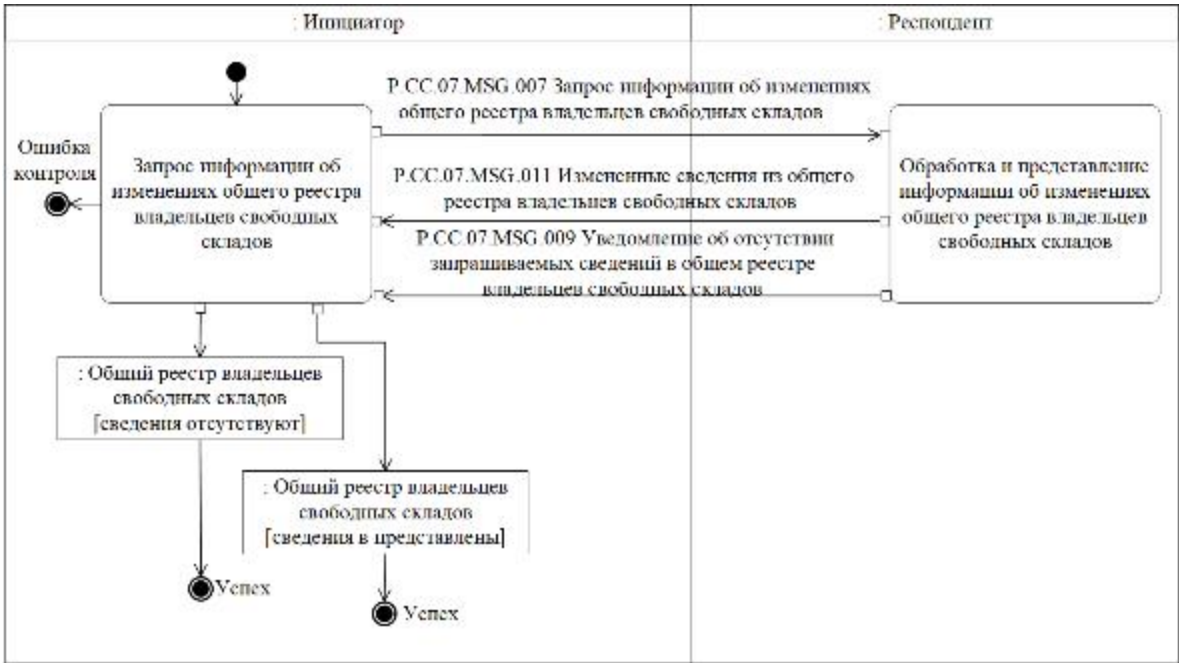
Рис. 9. Схема выполнения транзакции общего процесса "Получение информации об изменениях, внесенных в общий реестр владельцев свободных складов" (P.07.TRN.006)
