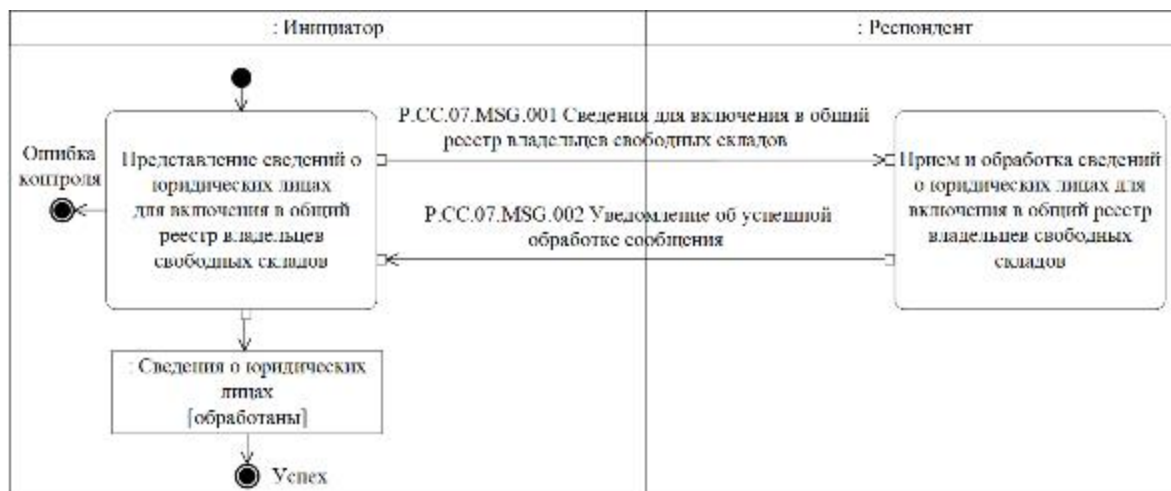
Рис. 4. Схема выполнения транзакции общего процесса "Включение сведений о юридических лицах в общий реестр владельцев свободных складов" (P.CC.07.TRN.001)
