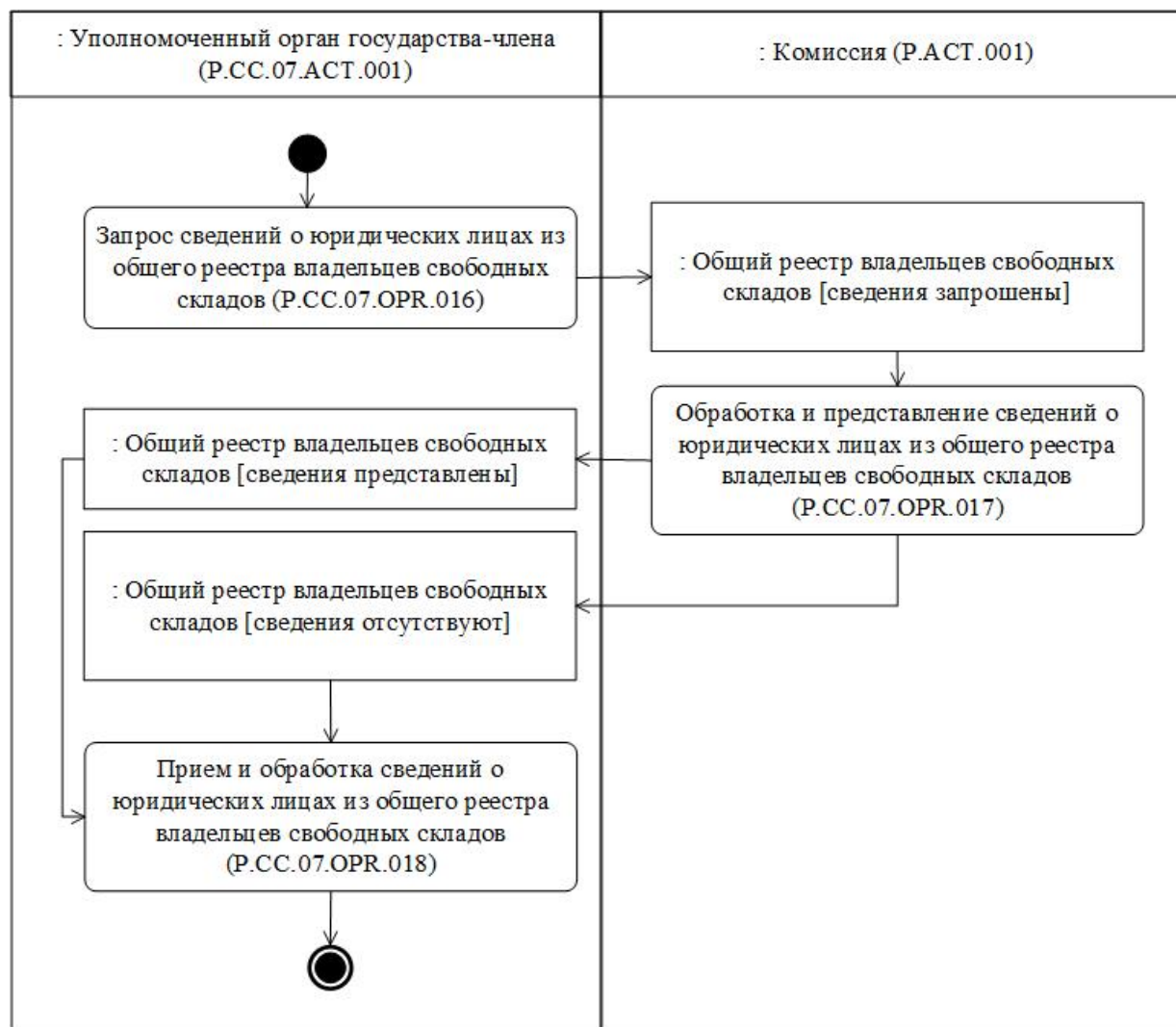
Рис. 10. Схема выполнения процедуры "Получение сведений о юридических лицах из общего реестра владельцев свободных складов" (P.CC.07.PRC.005)
