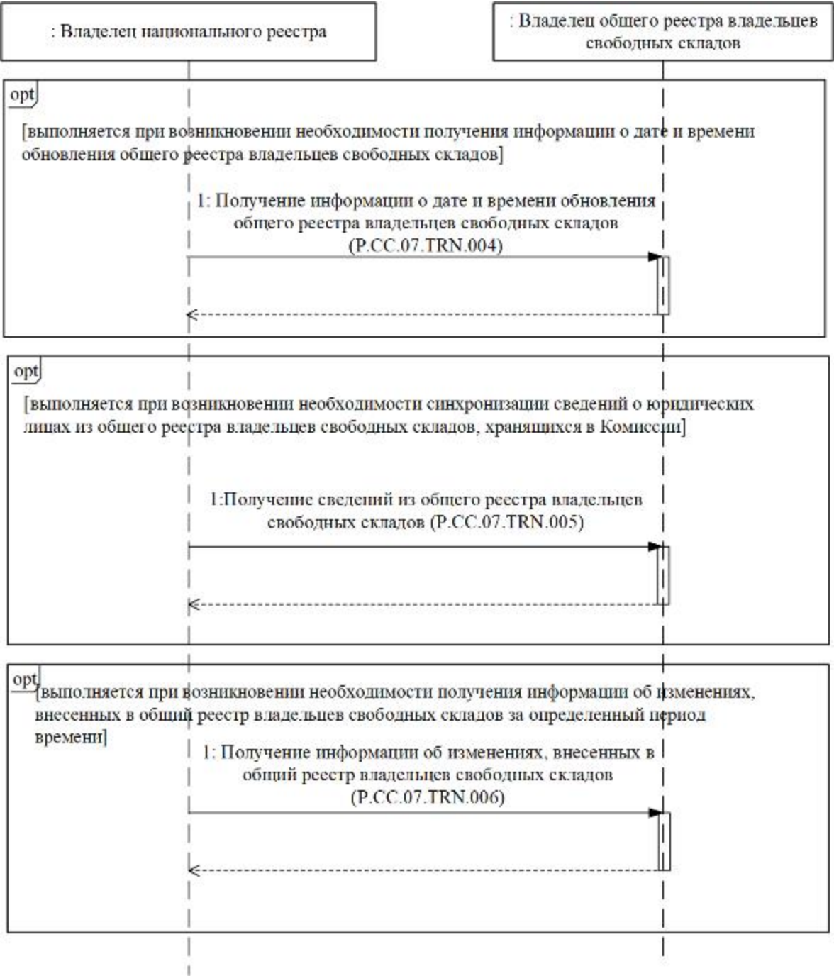
Рис. 3. Схема выполнения транзакций общего процесса при представлении уполномоченным органам государств-членов сведений о юридических лицах, содержащихся в общем реестре владельцев свободных складов
