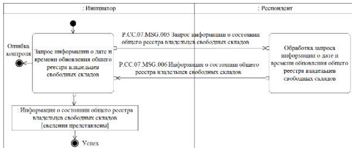
Рис. 7. Схема выполнения транзакции общего процесса "Получение информации о дате и времени обновления общего реестра владельцев свободных складов" (P.CC.07.TRN.004)
