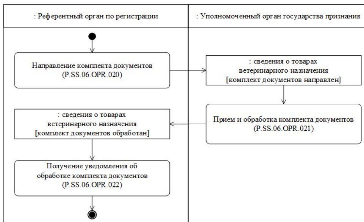
Рис. 13. Схема выполнения процедуры "Предоставление комплекта документов" (P.SS.06.PRC.007)
