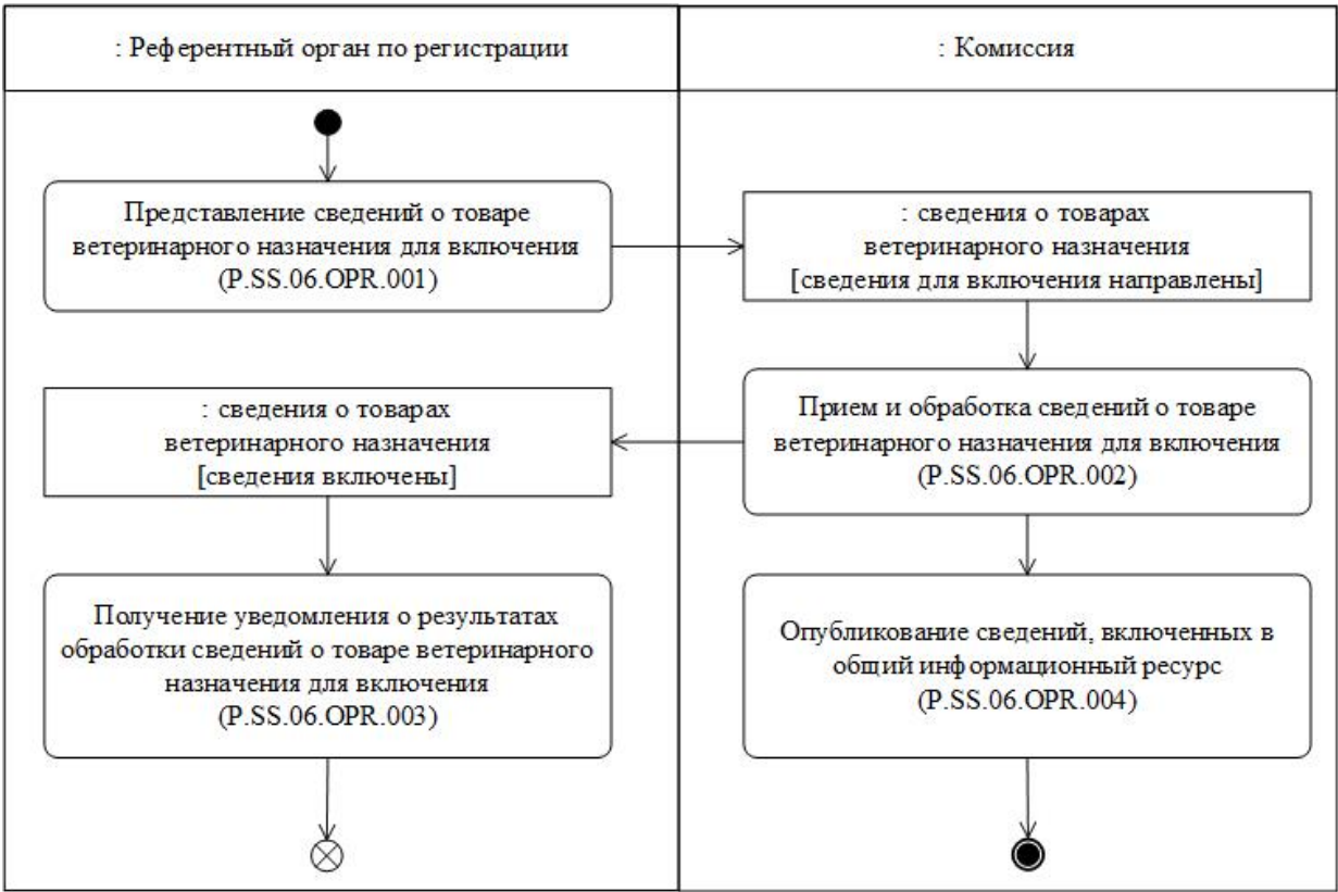
Рис. 7. Схема выполнения процедуры "Включение сведений в общий информационный ресурс" (P.SS.06.PRC.001)
