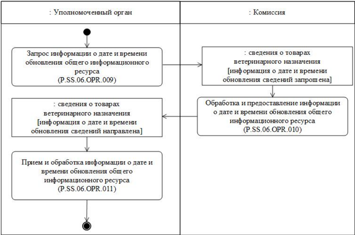
Рис. 9. Схема выполнения процедуры "Получение информации о дате и времени обновления общего информационного ресурса" (P.SS.06.PRC.003)
