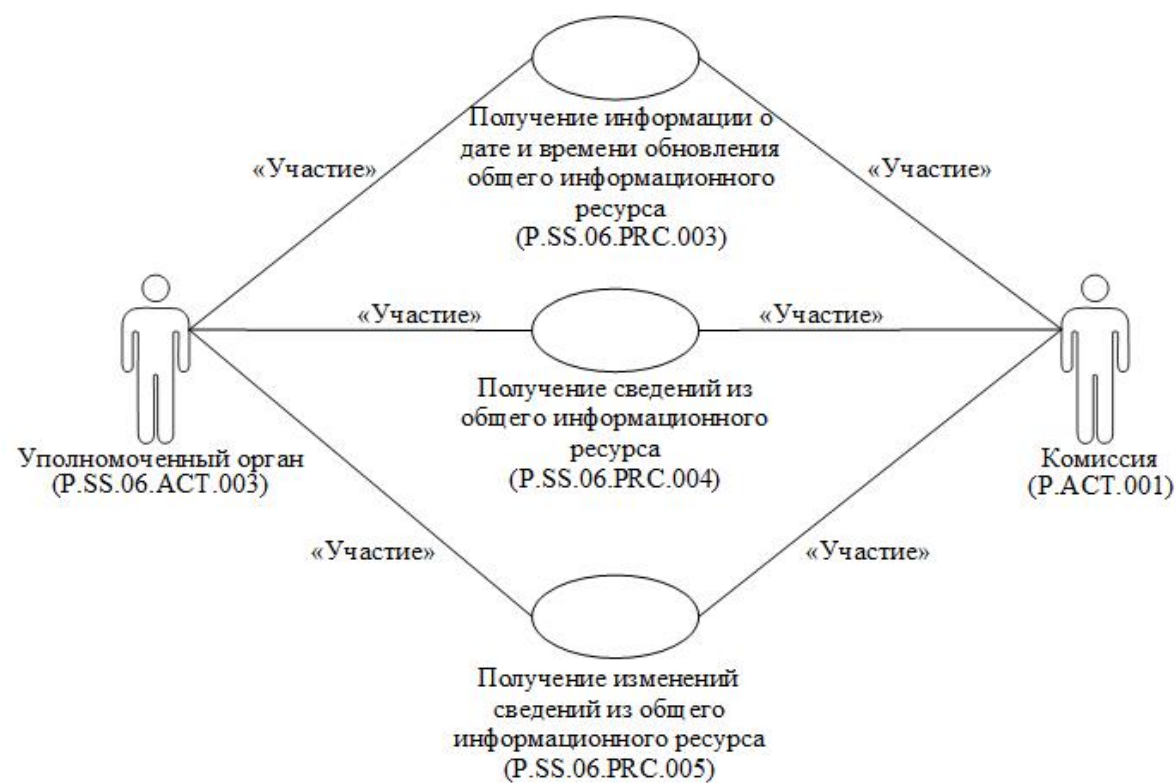
Рис. 3. Общая схема группы процедур получения сведений из общего информационного ресурса
