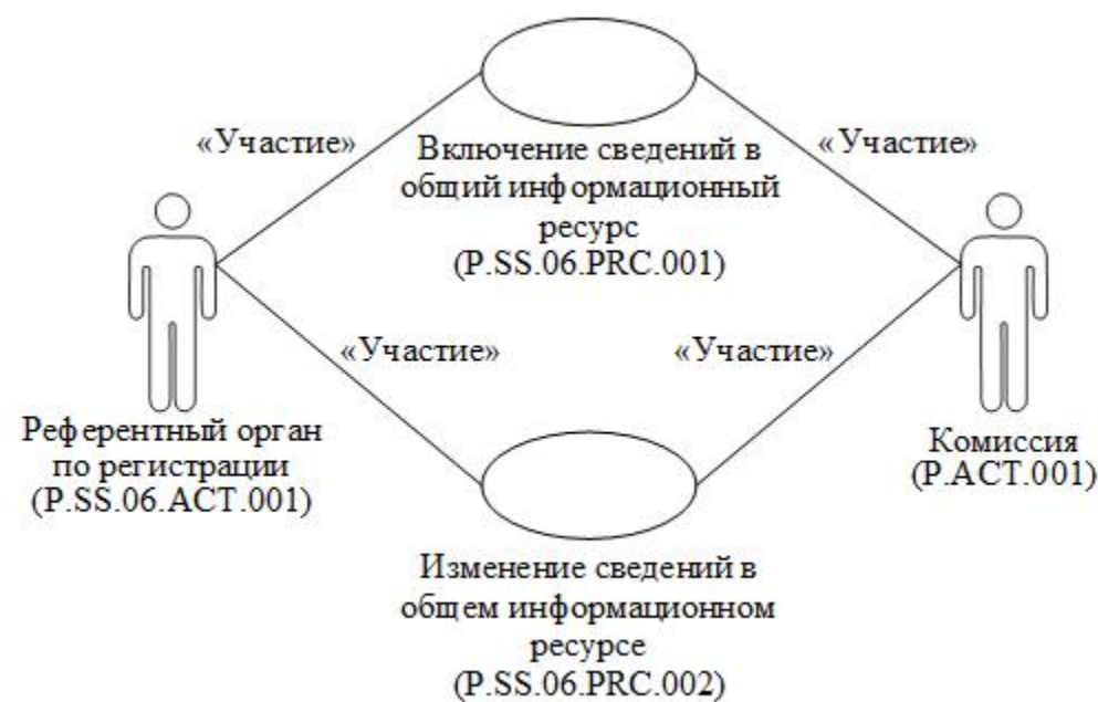
Рис. 2. Общая схема группы процедур формирования и ведения общего информационного ресурса
