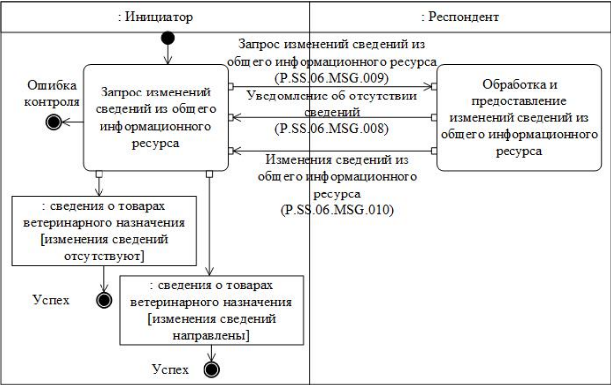
Рис. 8. Схема выполнения транзакции общего процесса "Получение изменений сведений из общего информационного ресурса" (P.SS.06.TRN.005)
