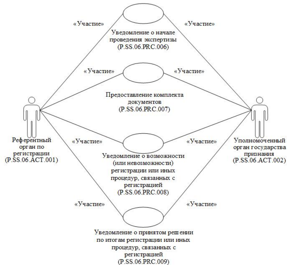
Рис. 4. Общая схема группы процедур обмена сведениями и документами, необходимыми для обмена в ходе регистрации или иных процедур, связанных с регистрацией
