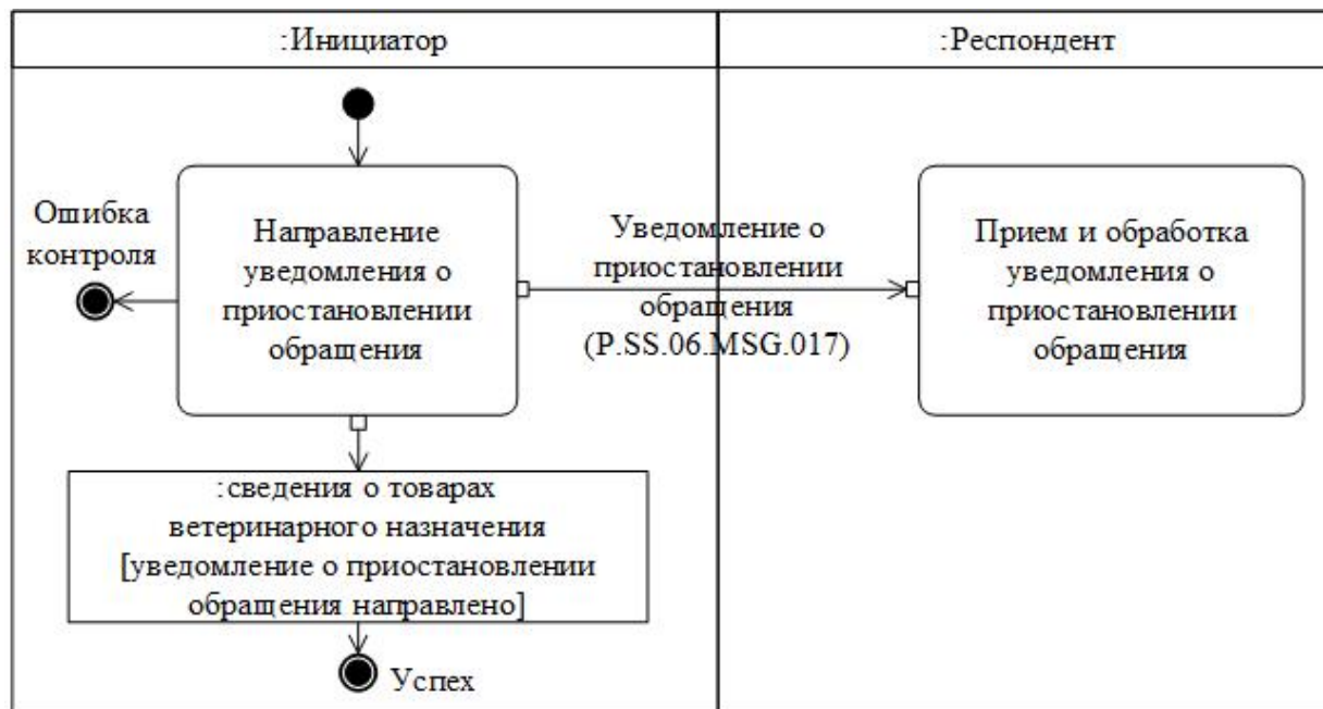
Рис. 11. Схема выполнения транзакции общего процесса "Уведомление о приостановлении обращения" (P.SS.06.TRN.012)
