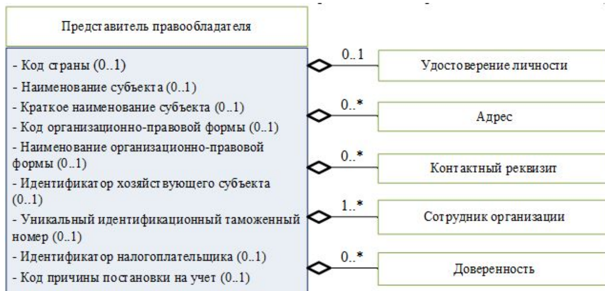
Рис. 13. Реквизиты, входящие в состав реквизита "Представитель правообладателя"
