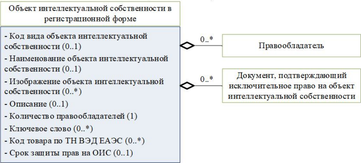
Рис. 3. Реквизиты, входящие в состав реквизита "Объект интеллектуальной собственности в регистрационной форме"
