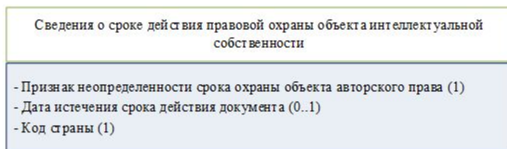
Рис. 11. Реквизиты, входящие в состав реквизита "Сведения о сроке действия правовой охраны объекта интеллектуальной собственности"
