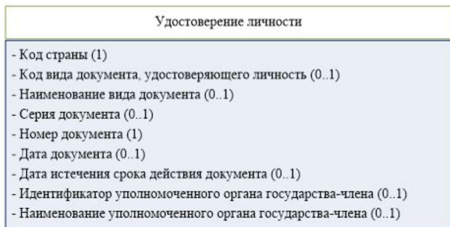
Рис. 5. Реквизиты, входящие в состав реквизита "Удостоверение личности"
