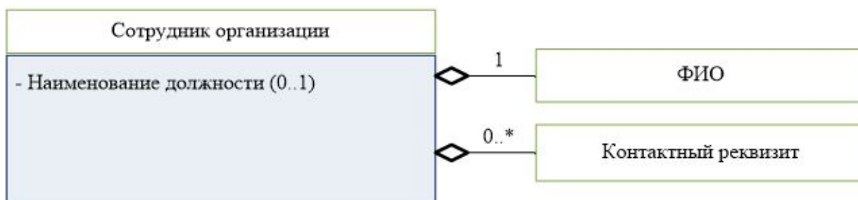
Рис. 8. Реквизиты, входящие в состав реквизита "Сотрудник организации"
