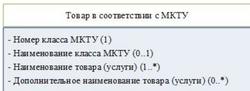
Рис. 12. Реквизиты, входящие в состав реквизита "Товар в соответствии с МКТУ"
