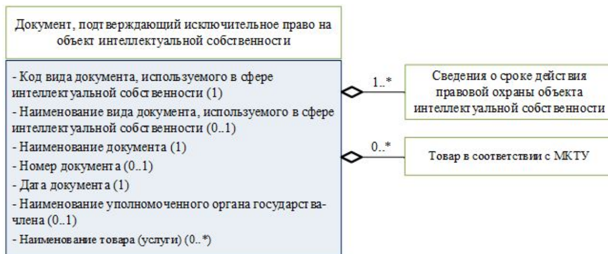
Рис. 10. Реквизиты, входящие в состав реквизита "Документ, подтверждающий исключительное право на объект интеллектуальной собственности"
