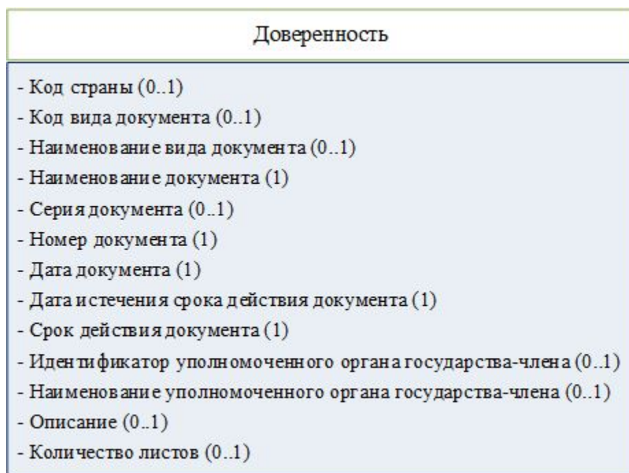
Рис. 14. Реквизиты, входящие в состав реквизита "Доверенность"
