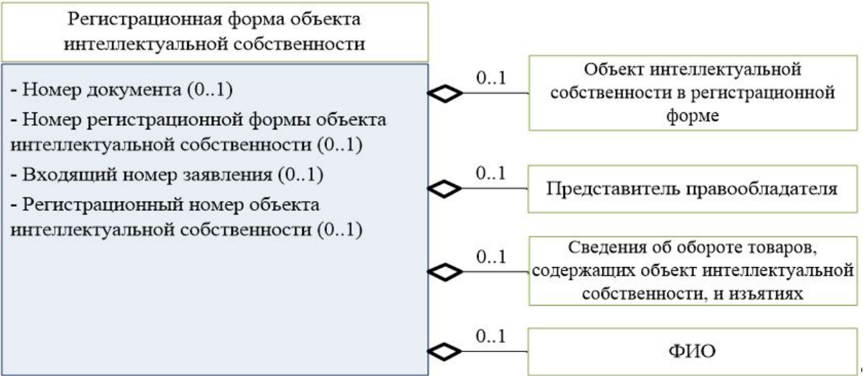
Рис. 2. Реквизиты, входящие в состав реквизита "Регистрационная форма объекта интеллектуальной собственности"
