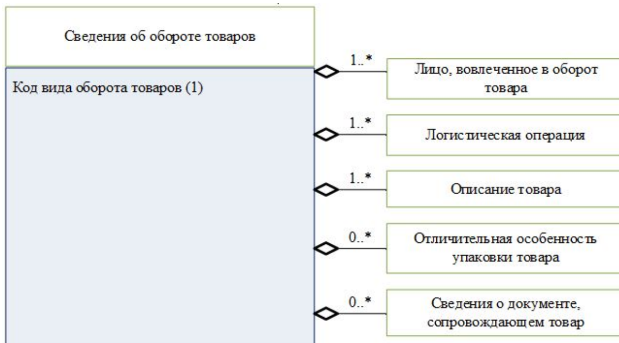
Рис. 16. Реквизиты, входящие в состав реквизита "Сведения об обороте товаров"
