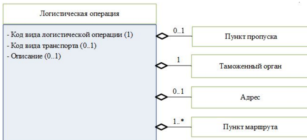
Рис. 18. Реквизиты, входящие в состав реквизита "Логистическая операция"
