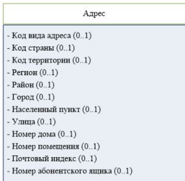
Рис. 6. Реквизиты, входящие в состав реквизита "Адрес"
