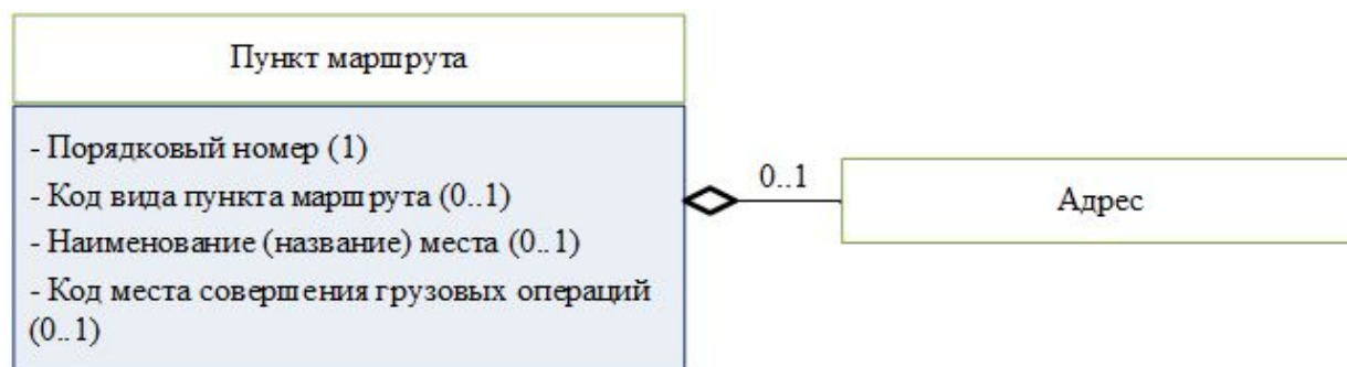
Рис. 22. Реквизиты, входящие в состав реквизита "Пункт маршрута" 3
