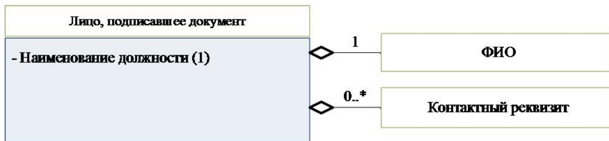
Рис. 28. Реквизиты, входящие в состав реквизита "Лицо, подписавшее документ" 5
