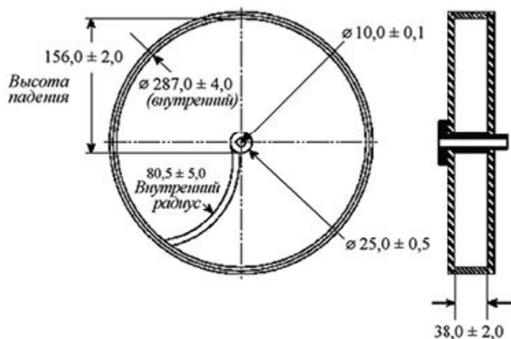
Рисунок 2.1.9.6.-1. – Прибор для определения истираемости таблеток. Размеры указаны в миллиметрах
