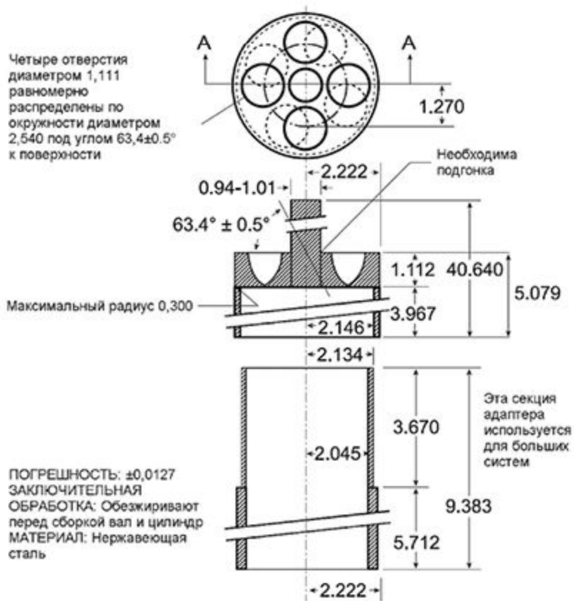
Рисунок 2.1.9.4.-5. – Схема вращающегося цилиндра. Размеры указаны в сантиметрах
