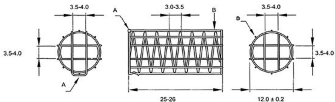
Рисунок 2.1.9.3.-3. – Альтернативное приспособление для погружения (размеры в миллиметрах). А – кислотоустойчивый проволоочный зажим; В – кислотоустойчивая проволоочная основа.
