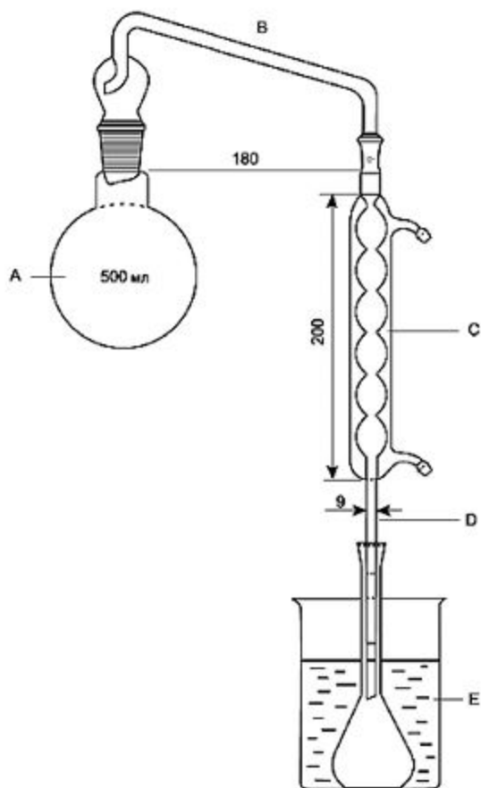
Рисунок 2.1.9.8.-2. - Схема прибора (2) для определения содержания этанола (размеры приведены в миллиметрах)
