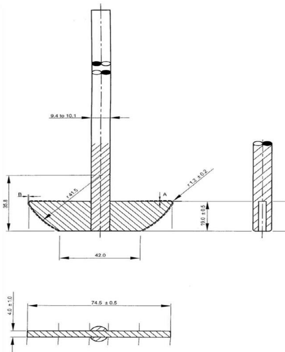
Рисунок 2.1.9.3.-2. – Прибор 2, перемешивающий элемент – лопасть. Размеры в миллиметрах.
