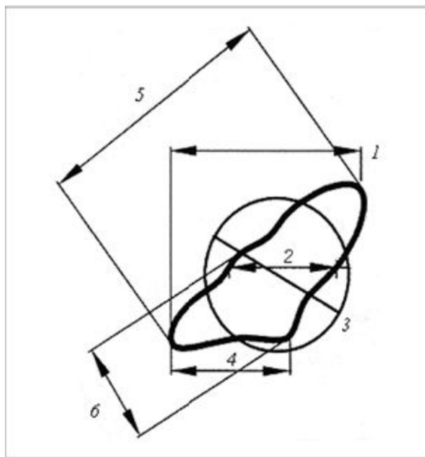
Рисунок 2.1.9.13.-2. - Способы определения размеров частиц неправильной формы.
