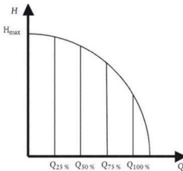
Рис. 3. Профиль нагрузки.
