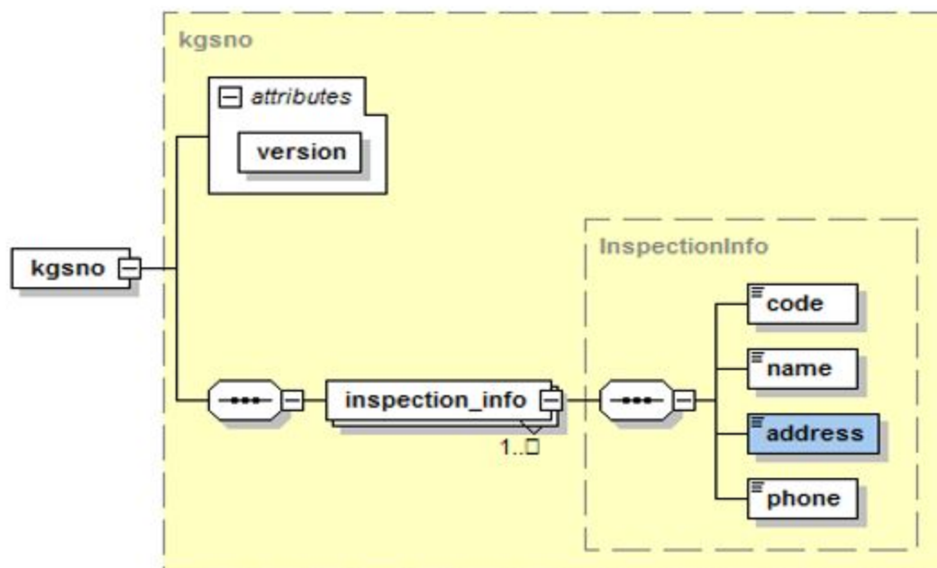
Рисунок Схема файла справочника KGSNO.
