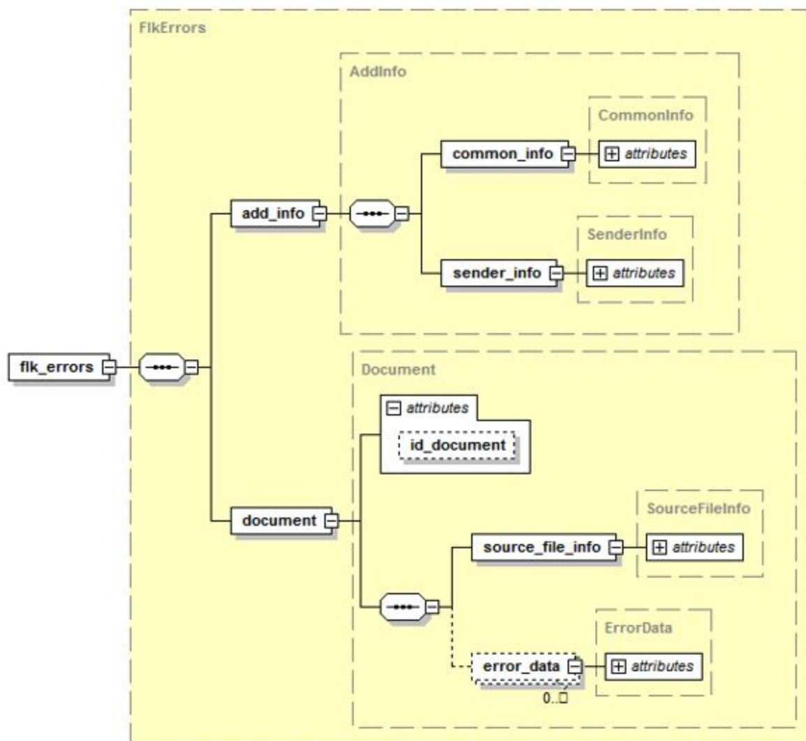
Рисунок 6.3.1 Схема файла протокола ФЛК.
