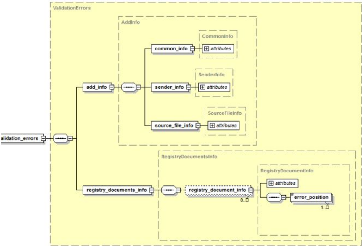
Рисунок 7.3.1 Схема файла протокола идентификации. Структура элементов указанной схемы приведена в следующих таблицах раздела 7.6. настоящего документа:
