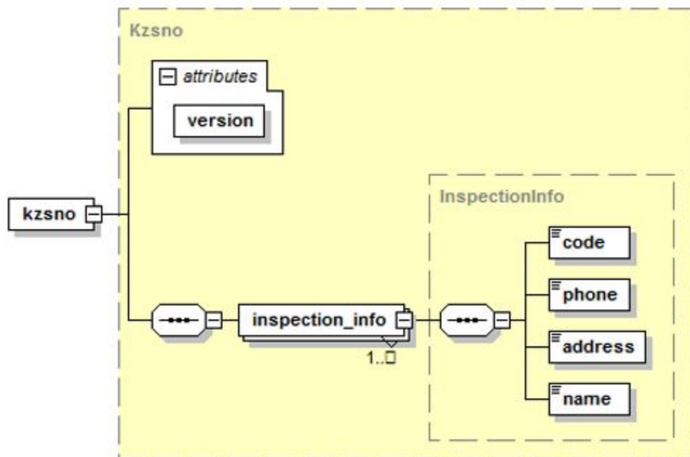
Рисунок 5.2.1. Схема файла справочника KZSNO.
