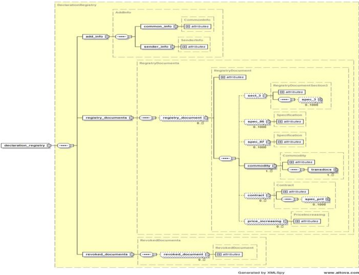
Рисунок 2.3.1 Схема файла реестра заявлений.
