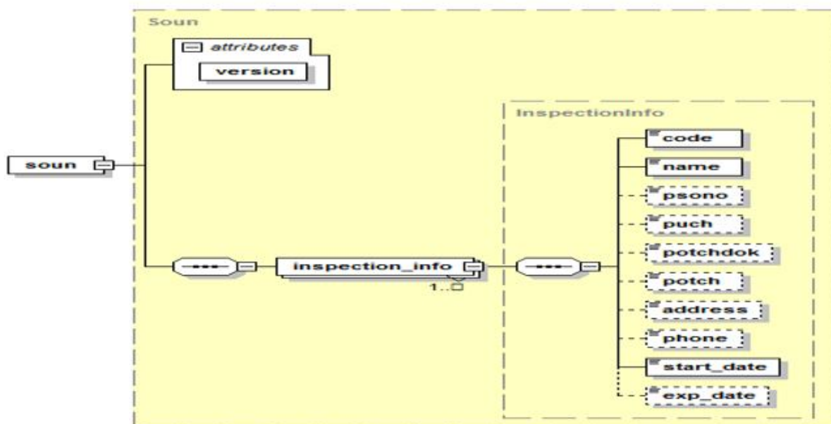
Рисунок 5.3.1. Схема файла справочника СОУН.
