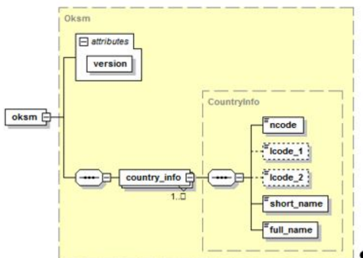
Рисунок 5.5.1. Схема файла справочника ОКСМ.
