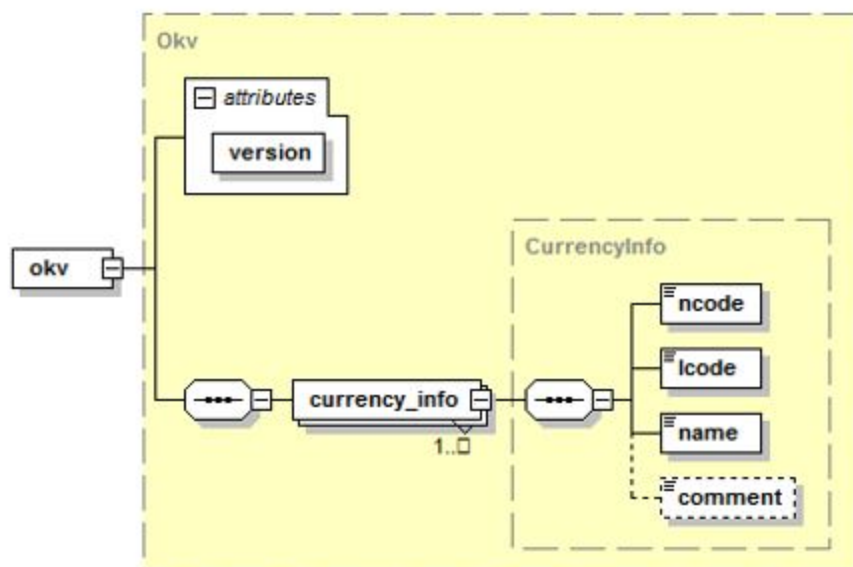
Рисунок 5.8.1. Схема файла справочника ОКВ.
