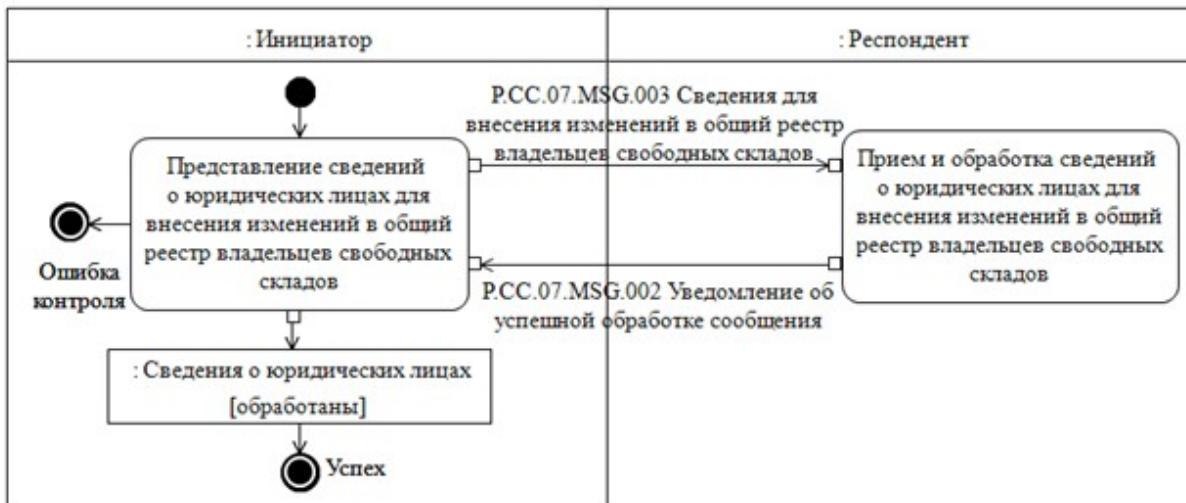
Рис. 5. Схема выполнения транзакции общего процесса «Изменение сведений о юридических лицах в общем реестре владельцев свободных складов» (P.CC.07.TRN.002)
