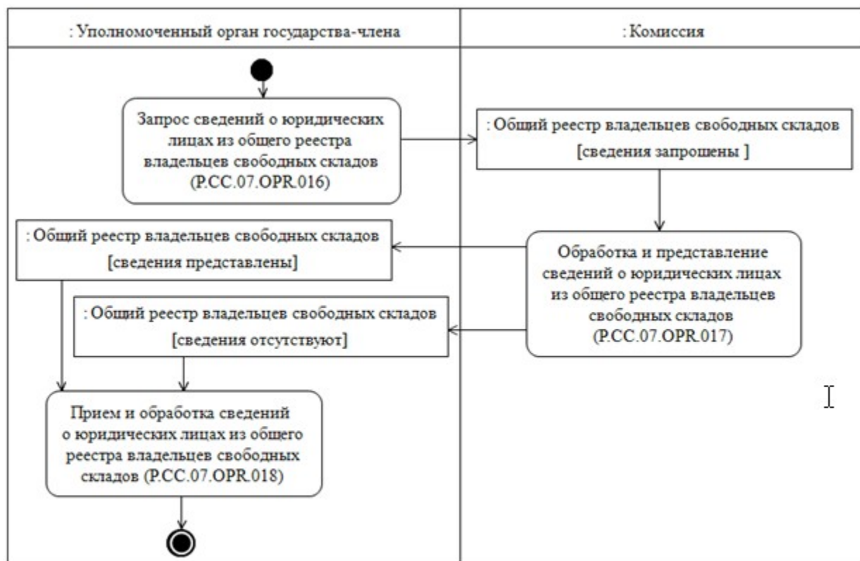
Рис. 9. Схема выполнения процедуры «Получение сведений о юридических лицах из общего реестра владельцев свободных складов» (P.CC.07.PRC.005)
