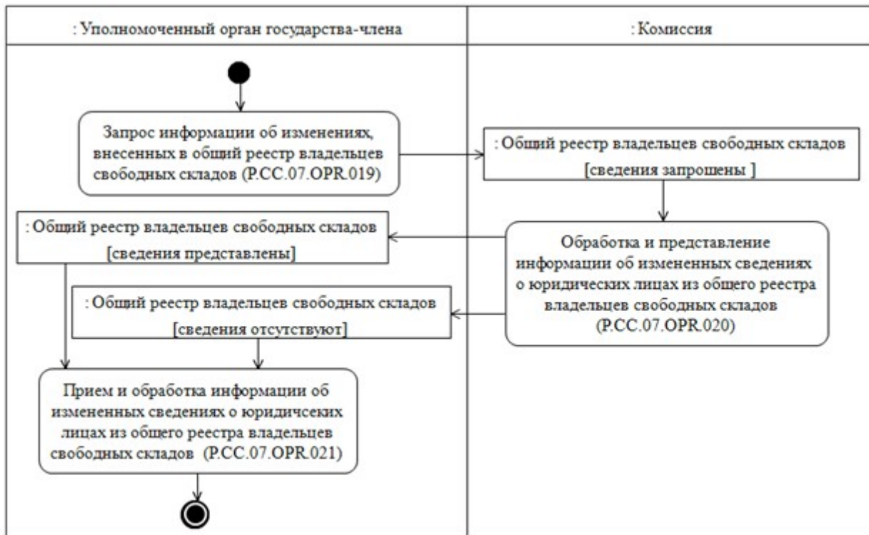
Рис. 10. Схема выполнения процедуры «Получение информации об изменениях, внесенных в общий реестр владельцев свободных складов» (P.CC.07.PRC.006)
