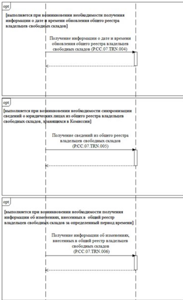
Рис. 3. Схема выполнения транзакций общего процесса при представлении уполномоченным органам государств-членов сведений о юридических лицах, содержащихся в общем реестре владельцев свободных складов
