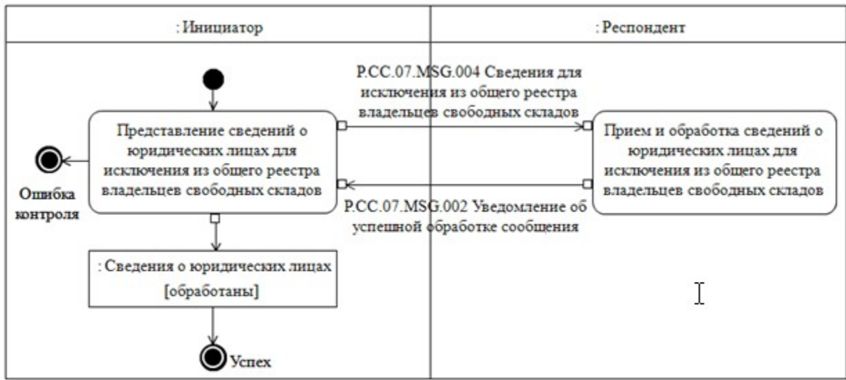
Рис. 6. Схема выполнения транзакции общего процесса «Исключение сведений о юридических лицах из общего реестра владельцев свободных складов» (P.CC.07.TRN.003)
