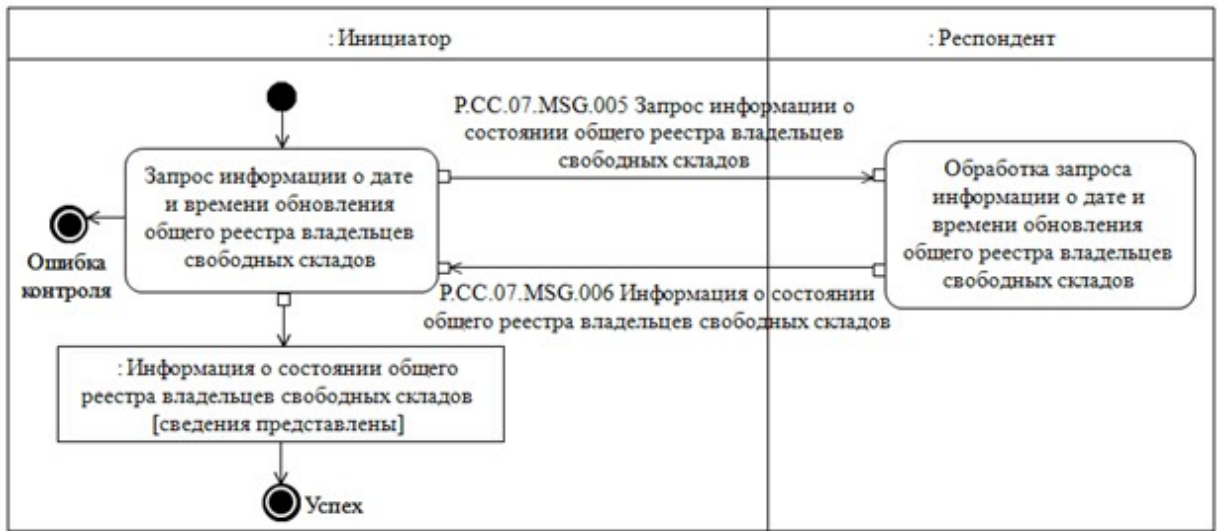
Рис. 7. Схема выполнения транзакции общего процесса «Получение информации о дате и времени обновления общего реестра владельцев свободных складов» (P.СC.07.TRN.004)
