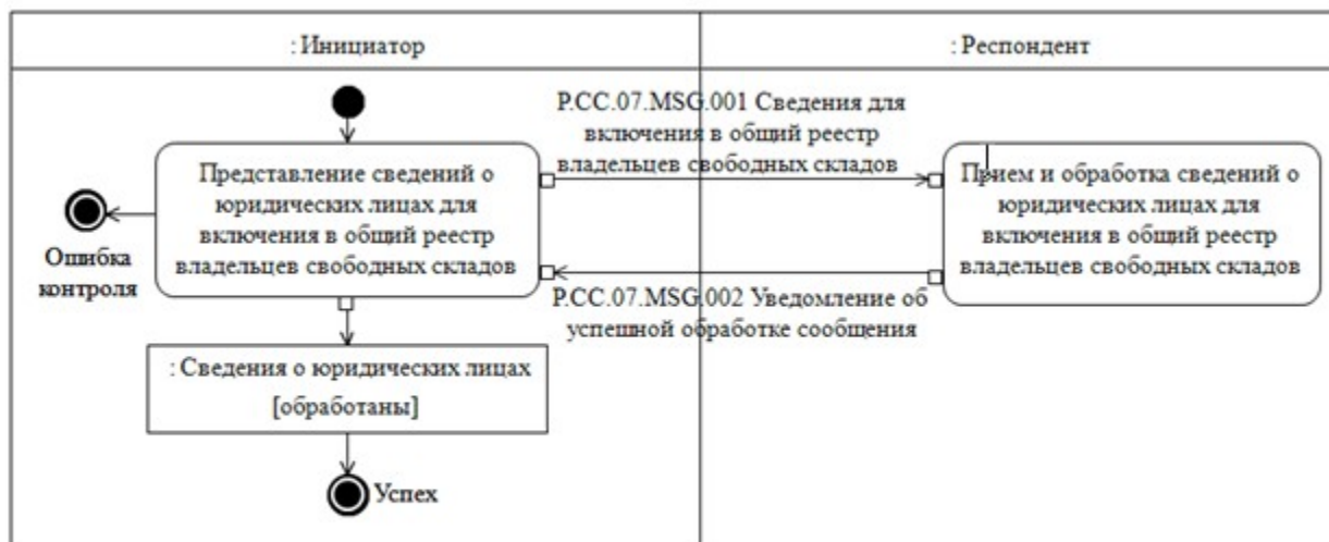
Рис. 4. Схема выполнения транзакции общего процесса «Включение сведений о юридических лицах в общий реестр владельцев свободных складов» (P.CC.07.TRN.001)
