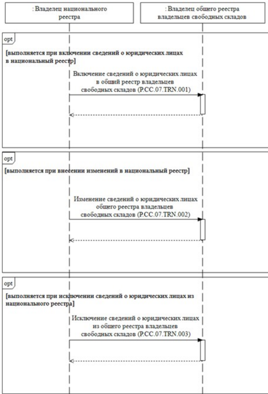
Рис. 2. Схема выполнения транзакций общего процесса при формировании и ведении общего реестра владельцев свободных складов
