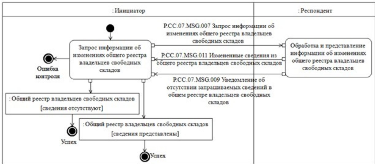
Рис. 9. Схема выполнения транзакции общего процесса «Получение информации об изменениях, внесенных в общий реестр владельцев свободных складов» (P.CC.07.TRN.006)
