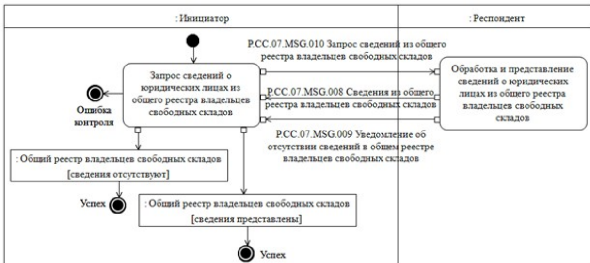
Рис. 8. Схема выполнения транзакции общего процесса «Получение сведений о юридических лицах из общего реестра владельцев свободных складов» (P.CC.07.TRN.005)
