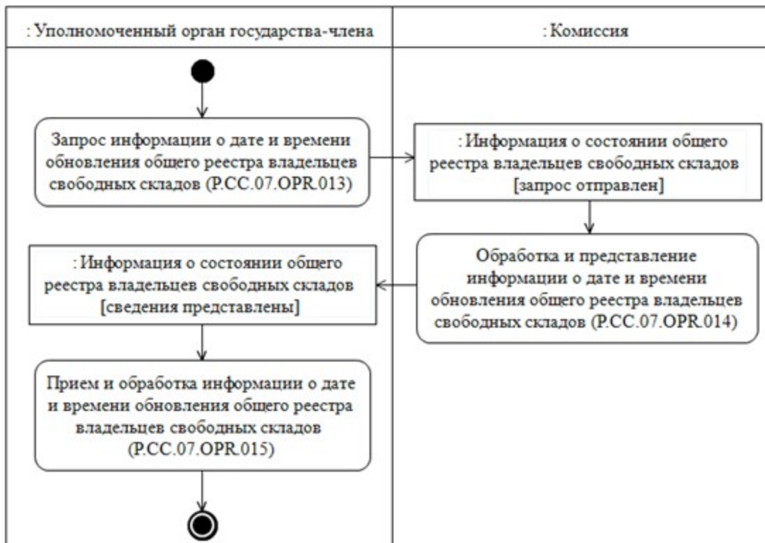
Рис. 8. Схема выполнения процедуры «Получение информации о дате и времени обновления общего реестра владельцев свободных складов» (Р.СС.07.ПРС.004)
