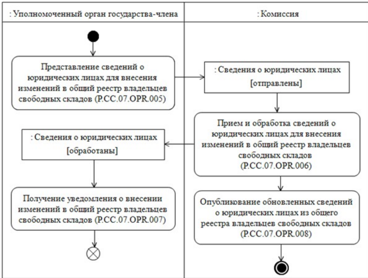
Рис. 6. Схема выполнения процедуры «Изменение сведений о юридических лицах, содержащихся в общем реестре владельцев свободных складов» (P.CC.07.PRC.002)
