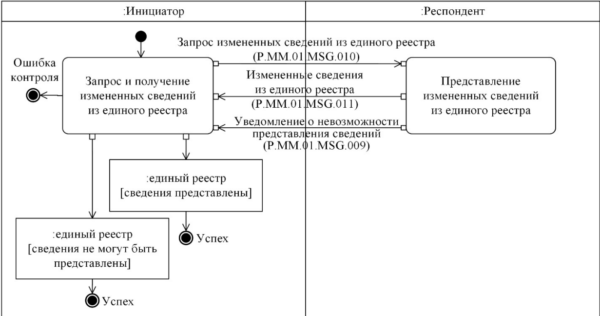
Рис. 9. Схема выполнения транзакции общего процесса "Получение измененных сведений из единого реестра" (P.MM.01.TRN.006)
