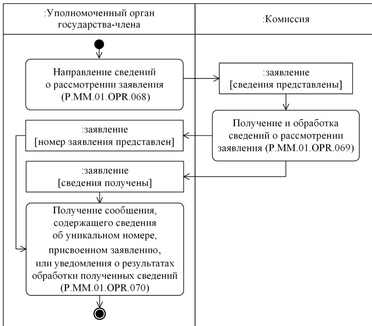
Рис. 25. Схема выполнения процедуры "Направление сведений о рассмотрении заявления" (P.MM.01.PRC.023)
