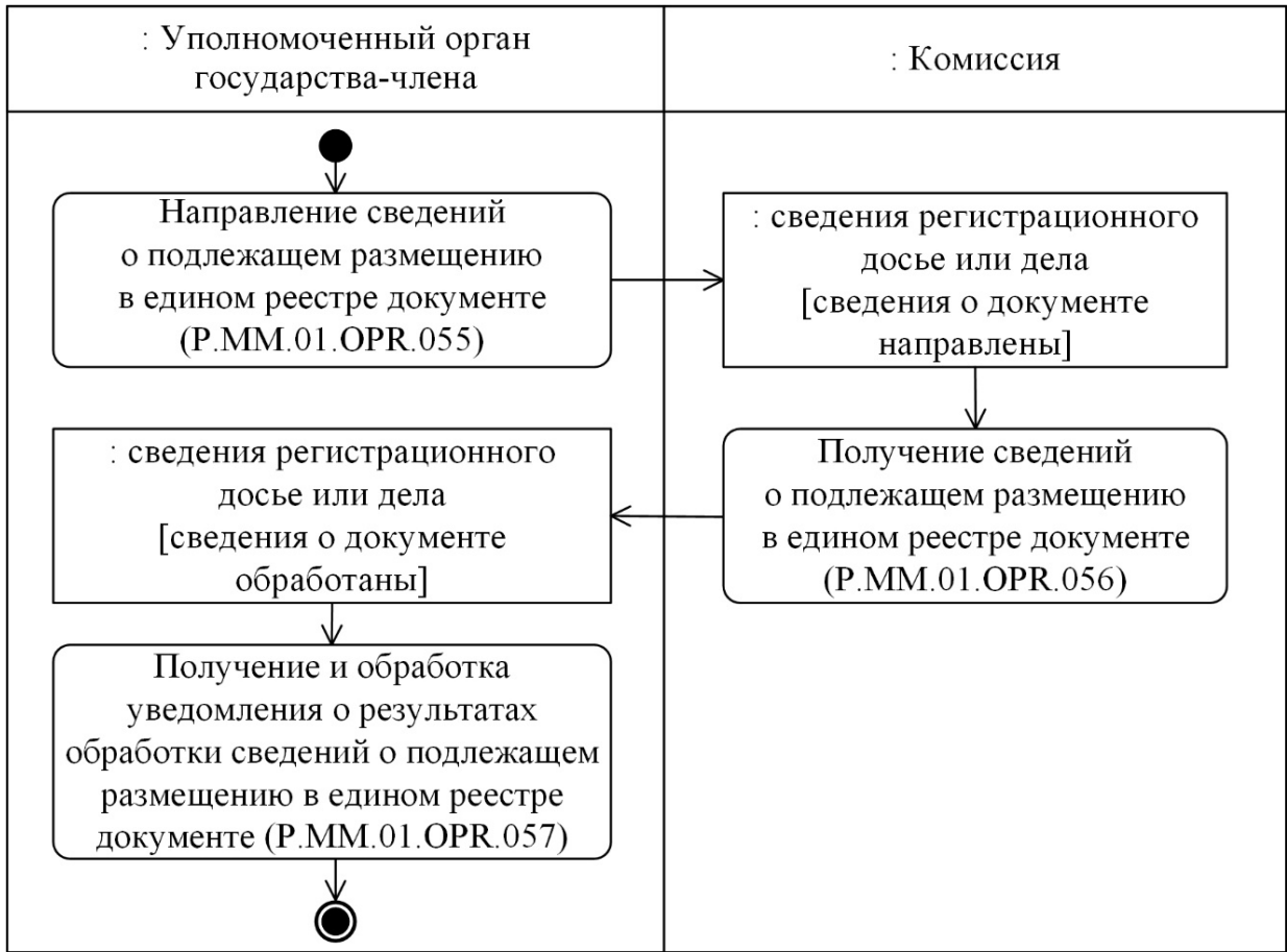
Рис. 12. Схема выполнения процедуры "Направление сведений о подлежащем размещению в едином реестре документе" (P.MM.01.PRC.019)
