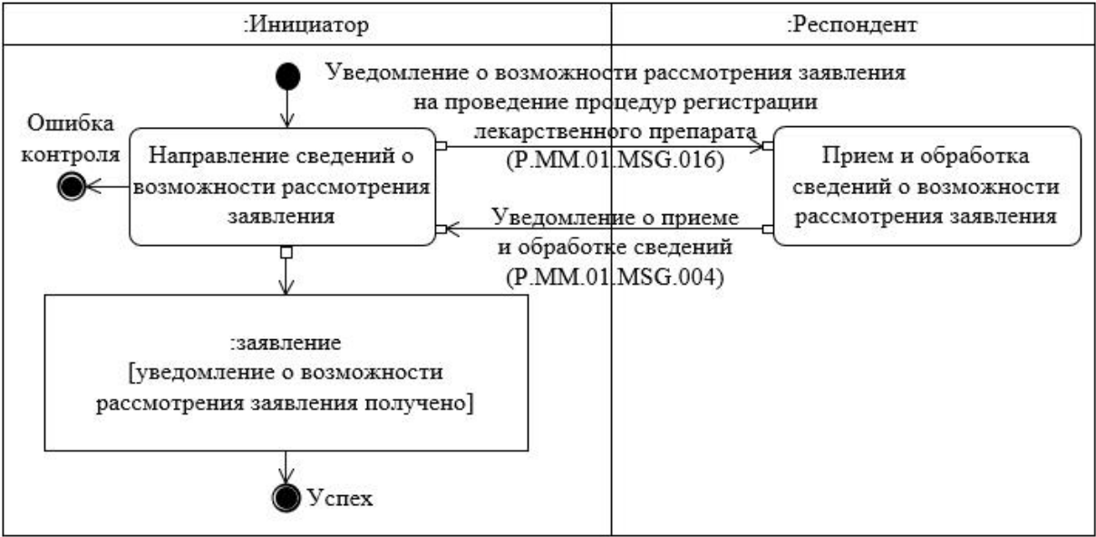
Рис. 7. Схема выполнения транзакции общего процесса "Уведомление о возможности рассмотрения заявления на проведение процедур регистрации лекарственного препарата" (P.MM.01.TRN.010)
