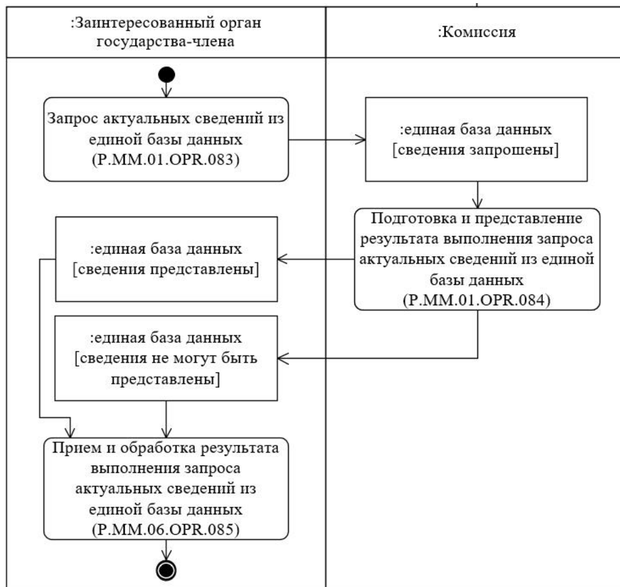
Рис. 36. Схема выполнения процедуры "Получение актуальных сведений из единой базы данных" (P.MM.01.PRC.028)
