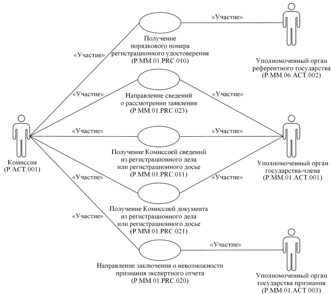
Рис. 5. Общая схема группы процедур "Процедуры взаимодействия с Комиссией при рассмотрении заявления" (P.MM.01.PGR.004)
