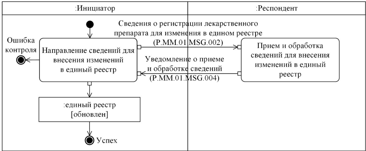
Рис. 6. Схема выполнения транзакции общего процесса "Изменение сведений, содержащихся в едином реестре" (P.MM.01.TRN.002)
