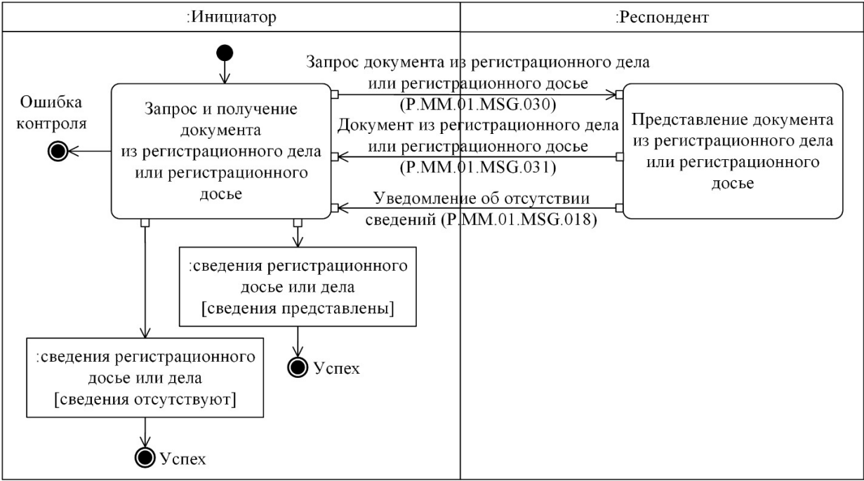
Рис. 16. Схема выполнения транзакции общего процесса "Получение Комиссией документа из регистрационного дела или регистрационного досье" (P.MM.01.TRN.021) Таблица 17
