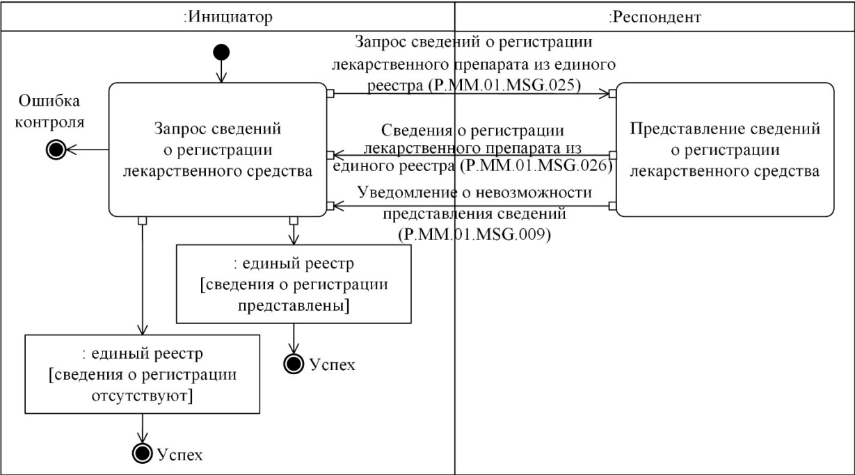
Рис. 12. Схема выполнения транзакции общего процесса "Получение сведений о регистрации лекарственного препарата из единого реестра" (P.MM.01.TRN.017)
