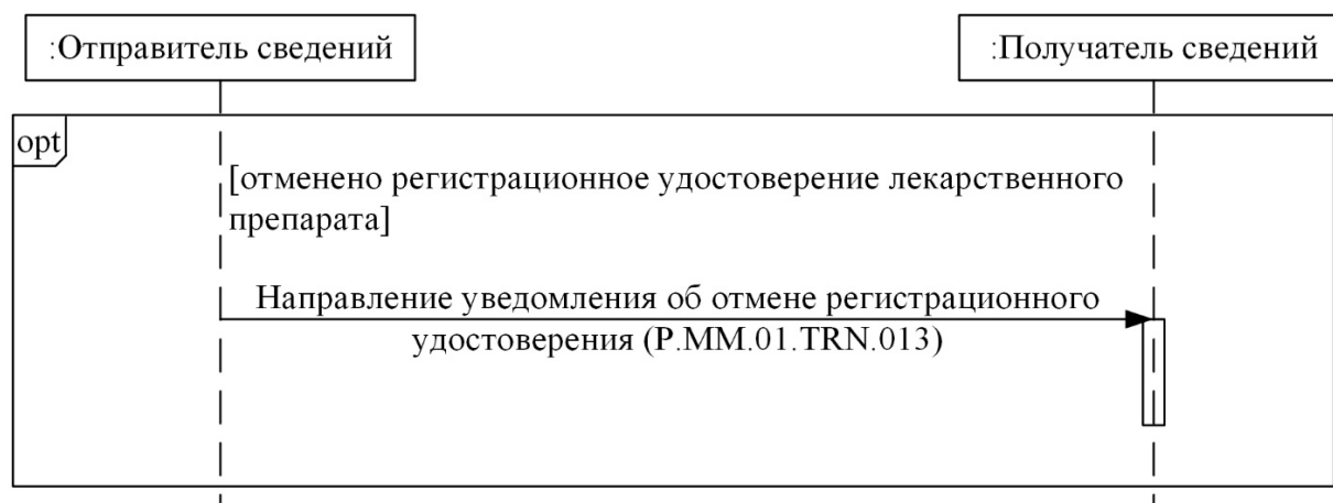
Рис. 4. Схема выполнения транзакций общего процесса при уведомлении об отмене регистрационного удостоверения
