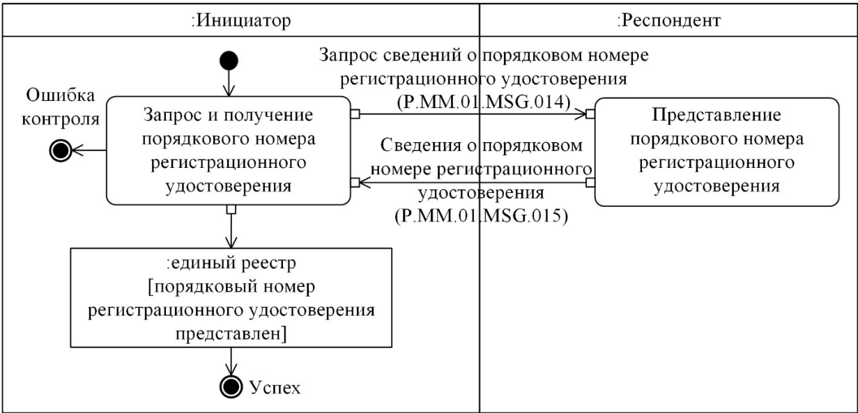
Рис. 10. Схема выполнения транзакции общего процесса "Получение порядкового номера регистрационного удостоверения" (P.MM.01.TRN.007)
