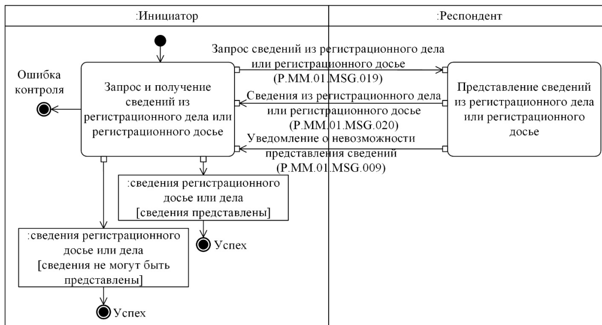
Рис. 9. Схема выполнения транзакции общего процесса "Получение сведений из регистрационного дела или регистрационного досье" (P.MM.01.TRN.012)
