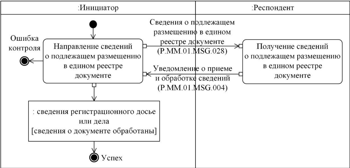
Рис. 14. Схема выполнения транзакции общего процесса "Направление сведений о подлежащем размещению в едином реестре документе" (P.MM.01.TRN.019)
