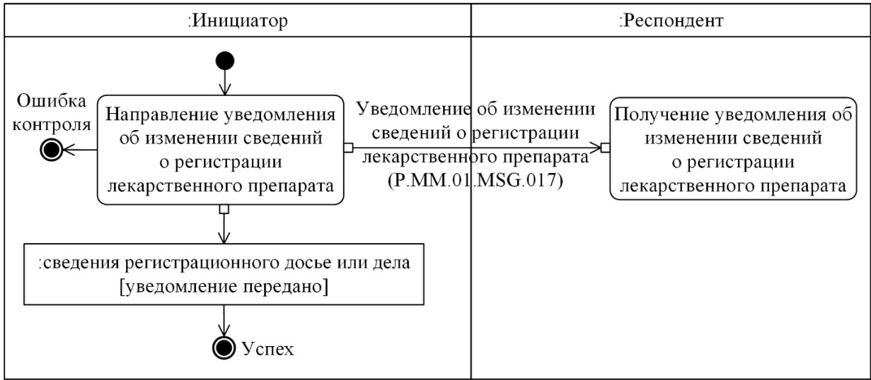
Рис. 8. Схема выполнения транзакции общего процесса "Уведомление об изменении сведений о регистрации лекарственного препарата" (P.MM.01.TRN.011) Таблица 9
