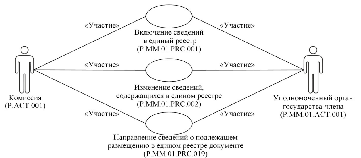
Рис. 2. Общая схема группы процедур "Процедуры формирования и ведения единого реестра" (P.MM.01.PGR.001)
