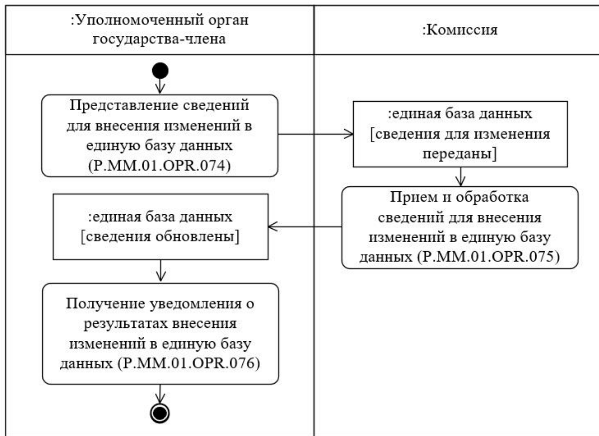
Рис. 33. Схема выполнения процедуры "Изменение сведений, содержащихся в единой базе данных" (Р.ММ.01.PRC.025)
