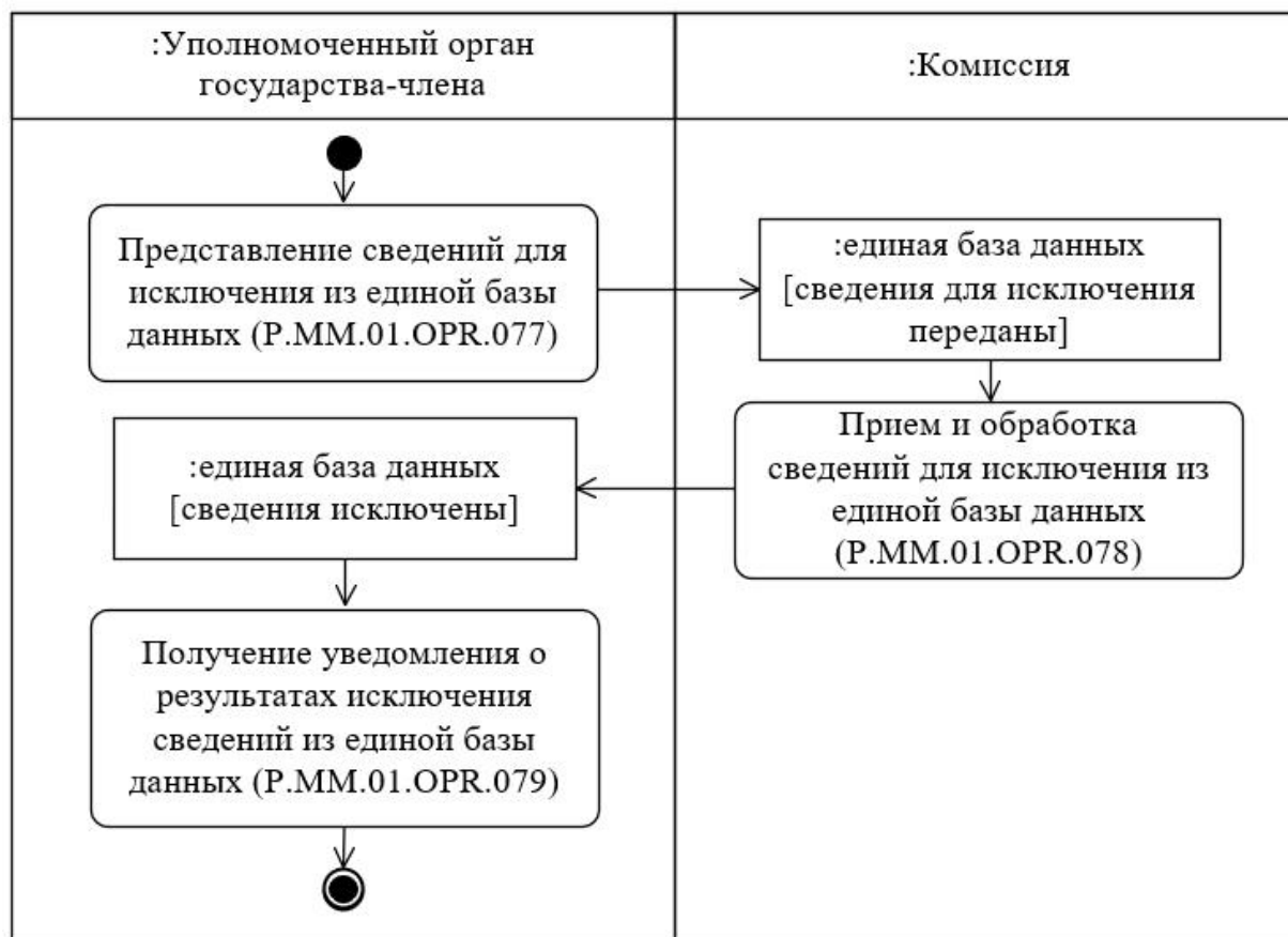
Рис. 34. Схема выполнения процедуры "Исключение сведений из единой базы данных" (P.MM.01.PRC.026)
