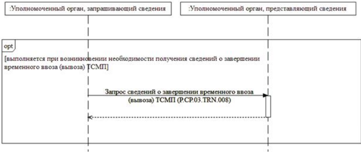
Рис. 6. Схема выполнения транзакций общего процесса при запросе сведений о завершении временного ввоза (вывоза) ТСМП
