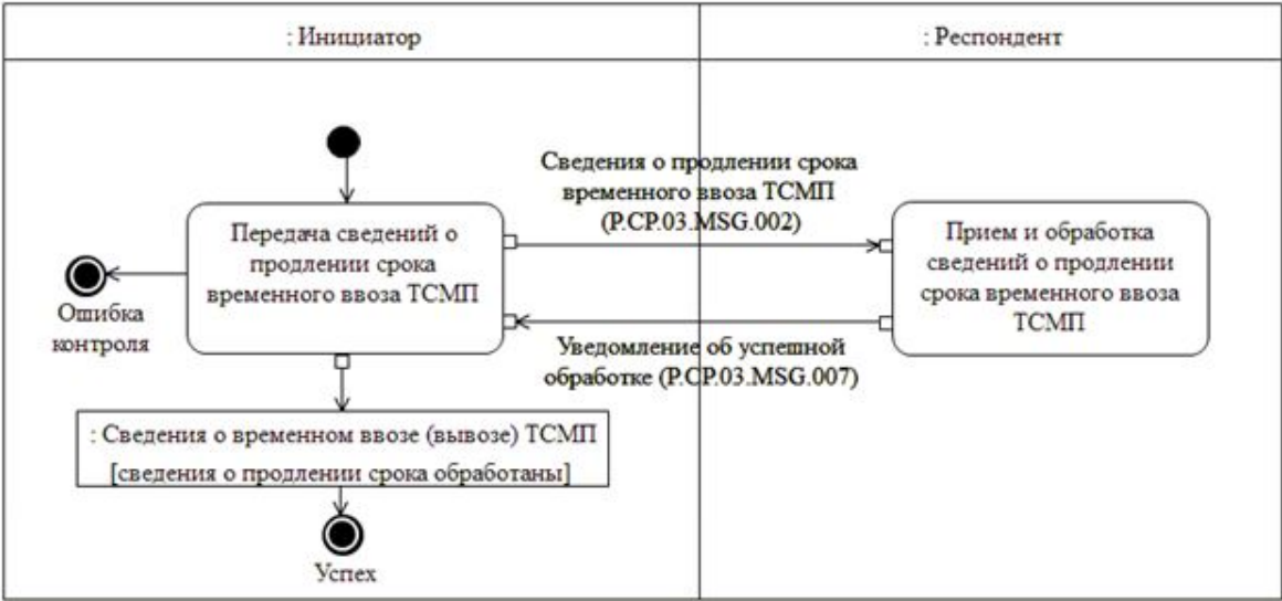
Рис. 7. Схема выполнения транзакции общего процесса "Передача сведений о продлении срока временного ввоза ТСМП" (P.CP.03.TRN.001)
