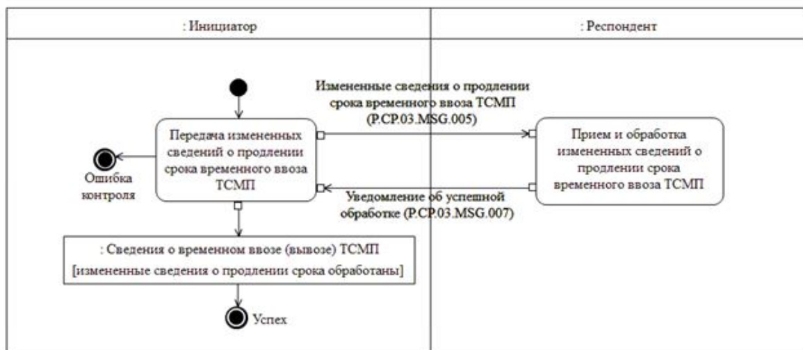
Рис. 8. Схема выполнения транзакции общего процесса "Передача измененных сведений о продлении срока временного ввоза ТСМП" (P.CP.03.TRN.002)
