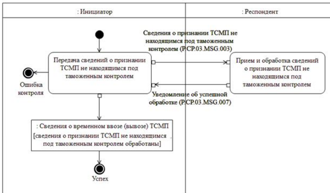
Рис. 11. Схема выполнения транзакции общего процесса "Передача сведений о признании ТСМП не находящимся под таможенным контролем" (P.CR.03.TRN.005)
