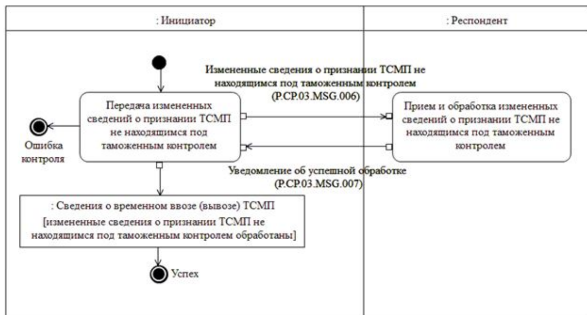
Рис. 12. Схема выполнения транзакции общего процесса "Передача измененных сведений о признании ТСМП не находящимся под таможенным контролем" (P.CP.03.TRN.006)
