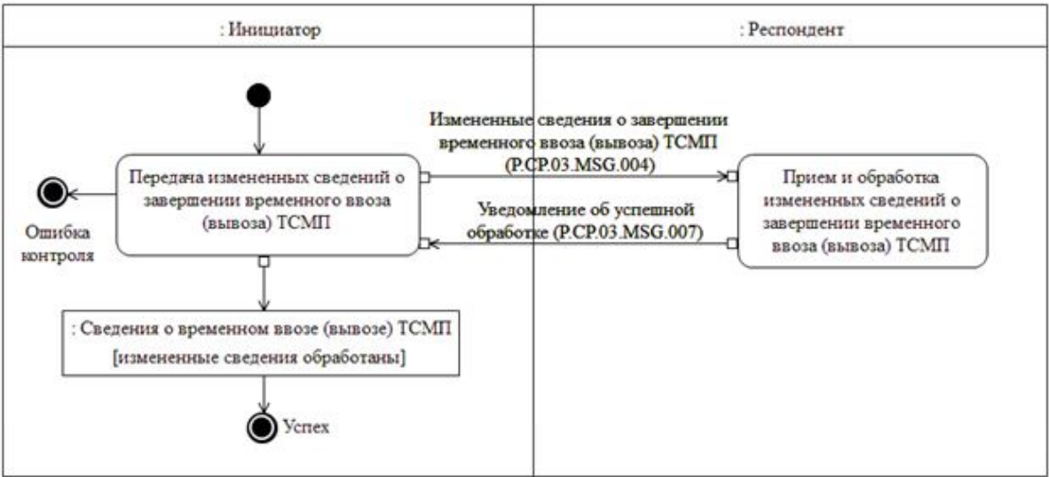
Рис. 10. Схема выполнения транзакции общего процесса "Передача измененных сведений о завершении временного ввоза (вывоза) ТСМП" (P.CP.03.TRN.004) Таблица 11
