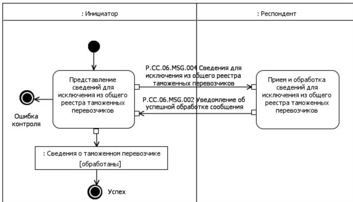
Рис. 6. Схема выполнения транзакции общего процесса "Исключение сведений из общего реестра таможенных перевозчиков" (P.CC.06.TRN.003) Таблица 7
