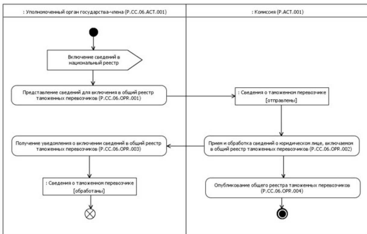
Рис. 5. Схема выполнения процедуры "Включение сведений в общий реестр таможенных перевозчиков" (P.CC.06.PRC.001)
