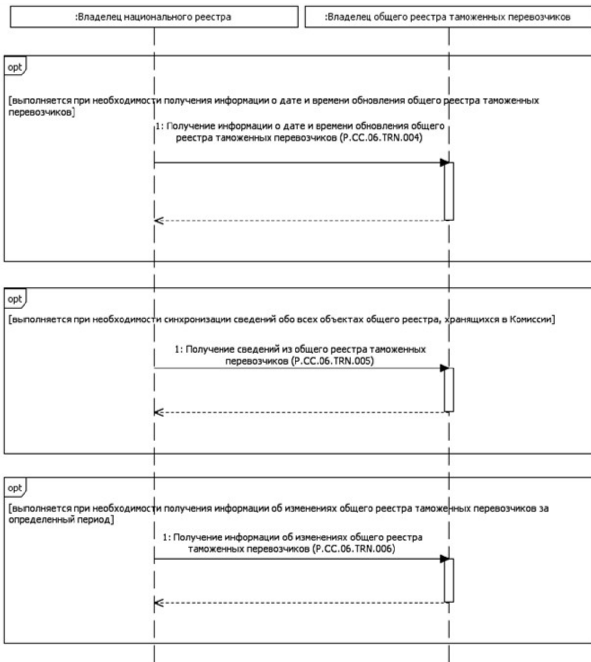
Рис. 3. Схема выполнения транзакций общего процесса при представлении уполномоченным органам государств-членов сведений, содержащихся в общем реестре таможенных перевозчиков
