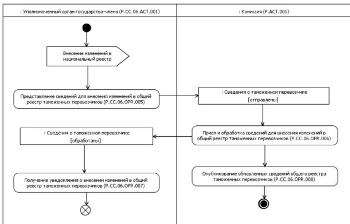
Рис. 6. Схема выполнения процедуры "Изменение сведений, содержащихся в общем реестре таможенных перевозчиков" (Р.С.С.06.ПРС.002)
