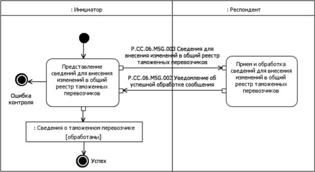
Рис. 5. Схема выполнения транзакции общего процесса "Изменение сведений общего реестра таможенных перевозчиков" (P.CC.06.TRN.002) Таблица 6
