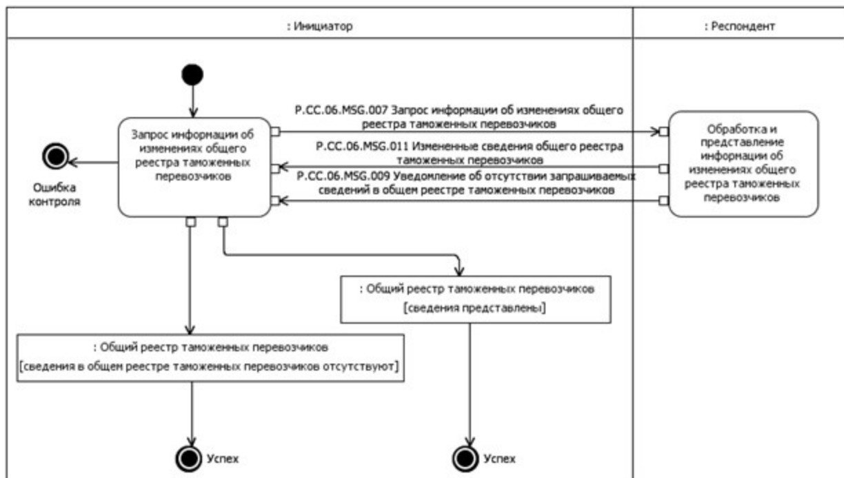
Рис. 9. Схема выполнения транзакции общего процесса "Получение информации об изменениях, внесенных в общий реестр таможенных перевозчиков" (P.06.TRN.006)
