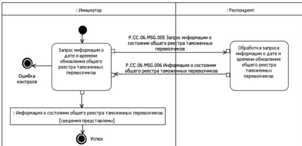
Рис. 7. Схема выполнения транзакции общего процесса "Получение информации о дате и времени обновления общего реестра таможенных перевозчиков" (P.СC.06.TRN.004)
