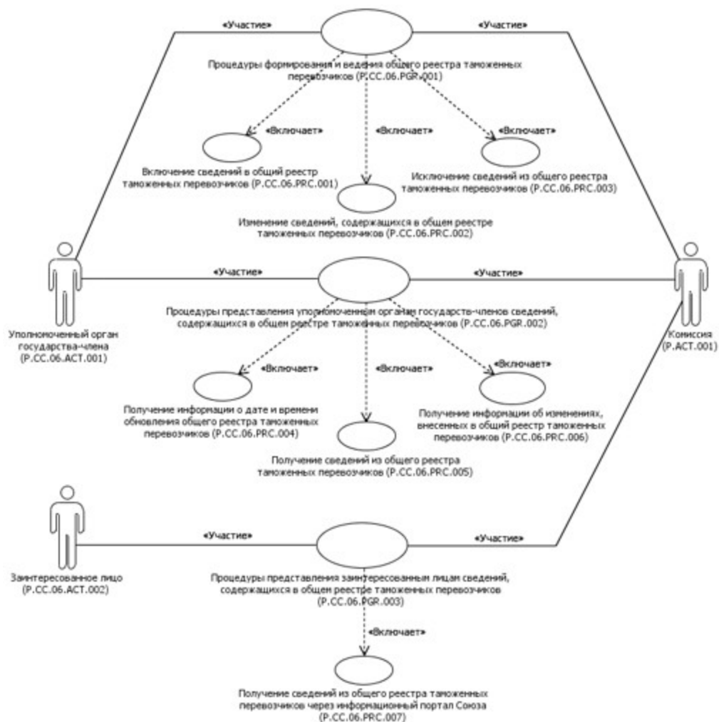
Рис. 1. Структура общего процесса
