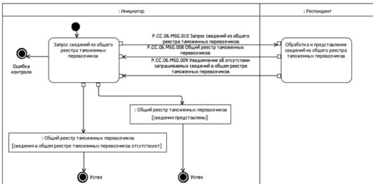
Рис. 8. Схема выполнения транзакции общего процесса "Получение сведений из общего реестра таможенных перевозчиков" (P.СC.06.TRN.005) Таблица 9
