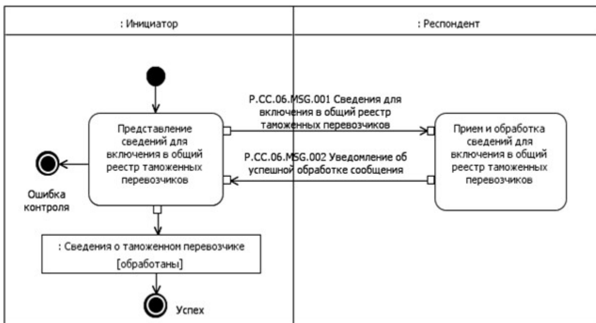
Рис. 4. Схема выполнения транзакции общего процесса "Включение сведений в общий реестр таможенных перевозчиков" (P.CC.06.TRN.001)
