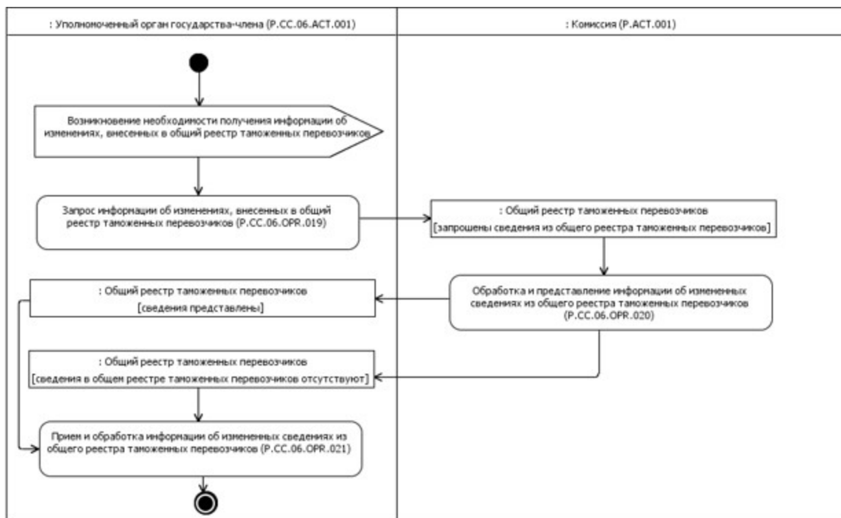
Рис. 10. Схема выполнения процедуры "Получение информации об изменениях, внесенных в общий реестр таможенных перевозчиков" (P.CC.06.PRC.006)
