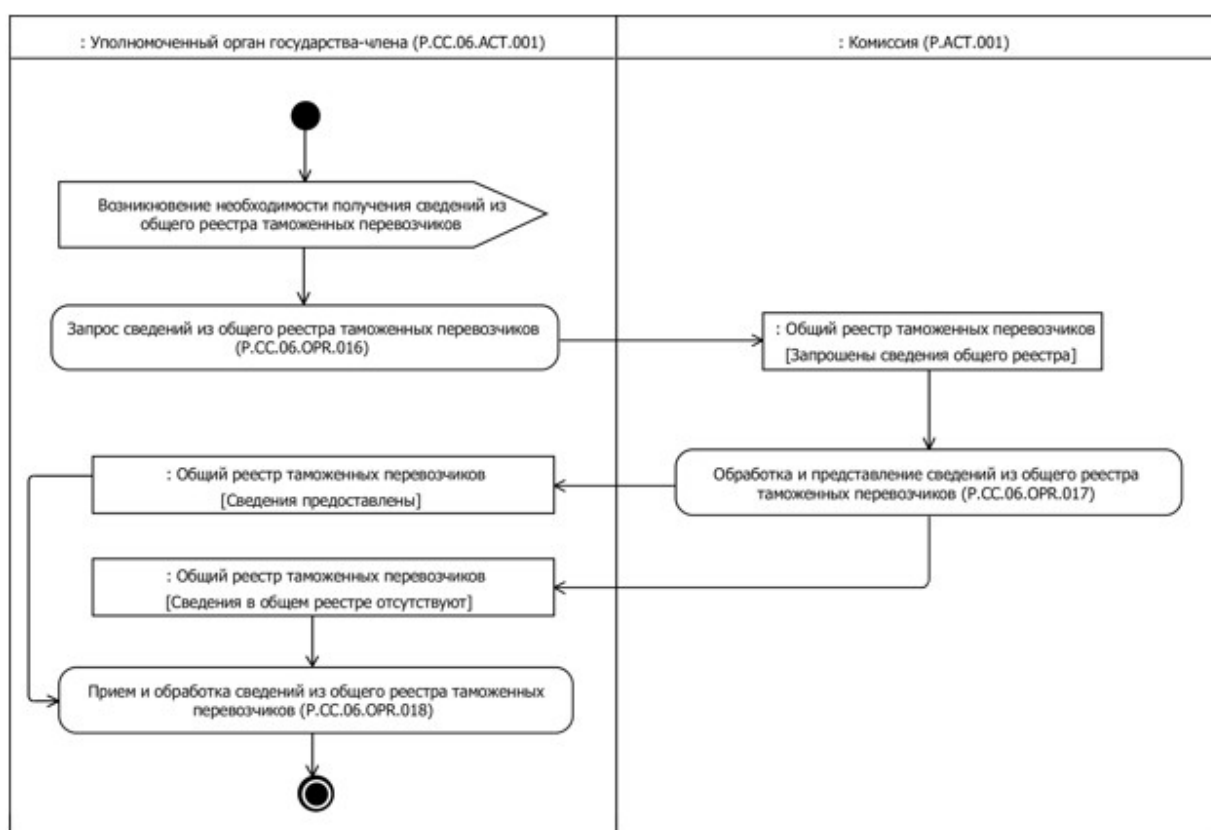
Рис. 9. Схема выполнения процедуры "Получение сведений из общего реестра таможенных перевозчиков" (P.CC.06.PRC.005)
