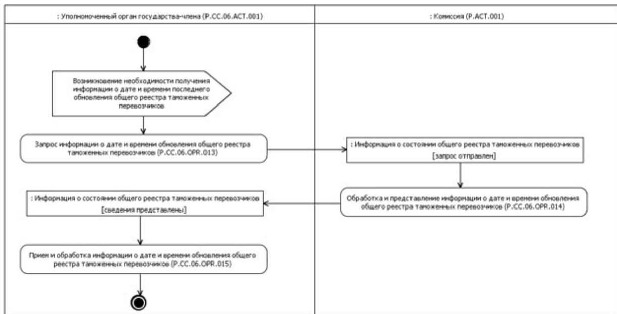
Рис. 8. Схема выполнения процедуры "Получение информации о дате и времени обновления общего реестра таможенных перевозчиков" (P.CC.06.PRC.004)
