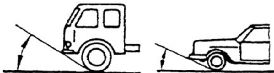
Рисунок 1. Угол въезда
