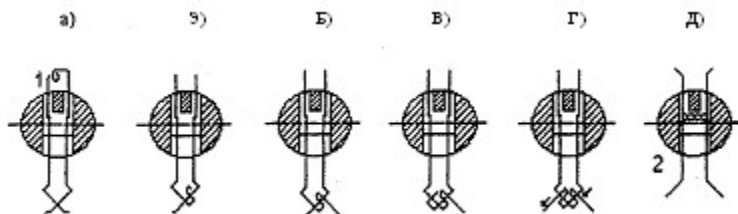
3-сурет. Камералы полиэтилен пломбаларды ілу тәсілінің схемасы:
