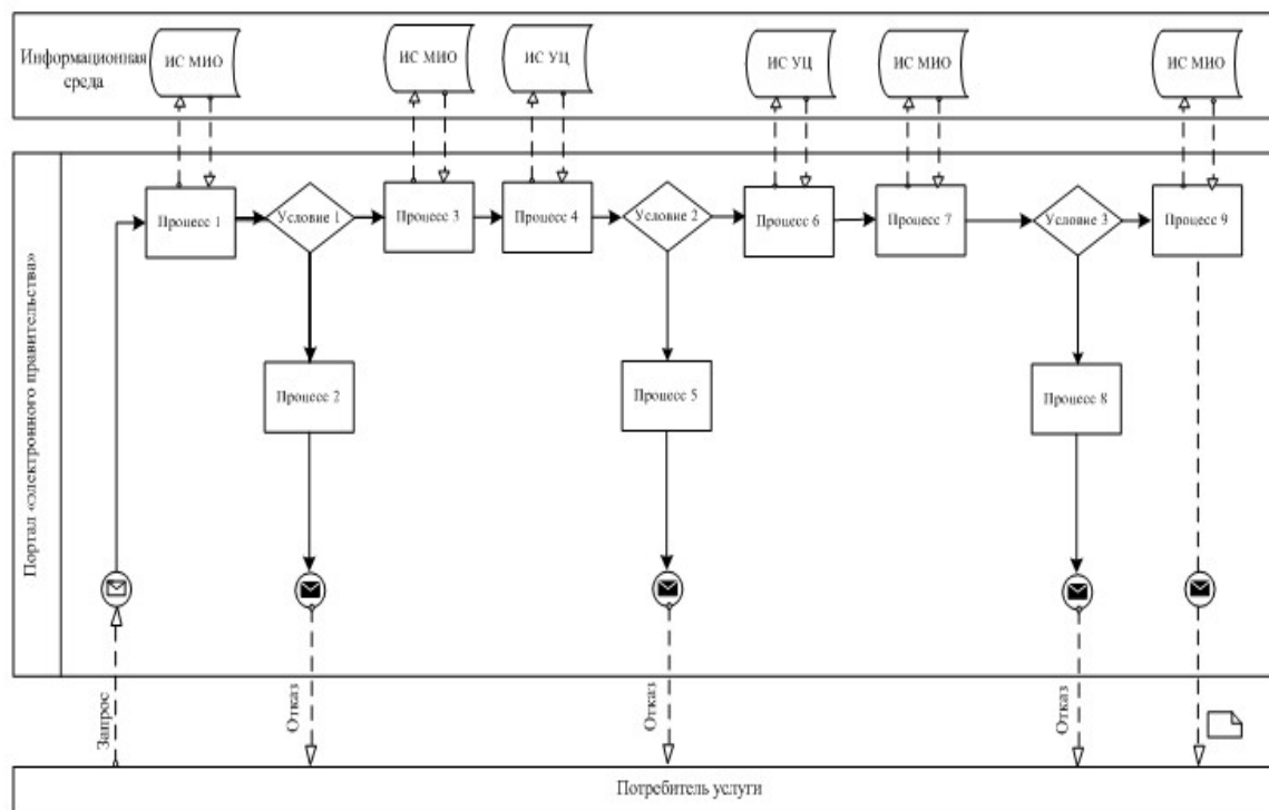
1 сурет. ЖАО АЖ арқылы «ішінара автоматтандырылған» электрондық мемлекеттік қызмет көрсету кезін функционалдык өзара іс-әрекет диаграммасы
