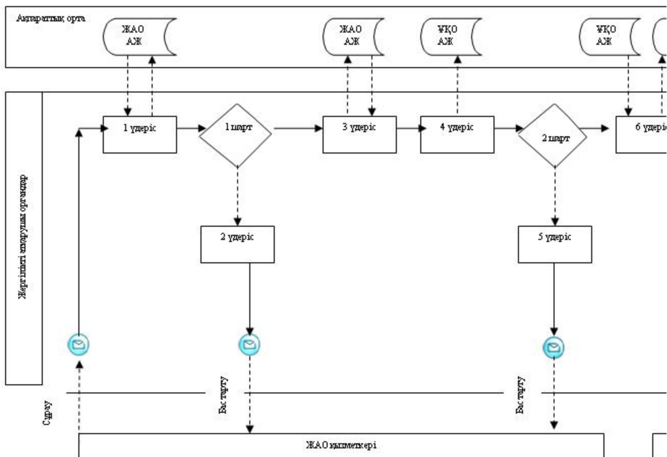
1 сурет. ЖАӨ АЖ арқылы «жартылай автоматтандырылған» электрондық мемл өзара функционалдық әрекеттесу диаграммасы
