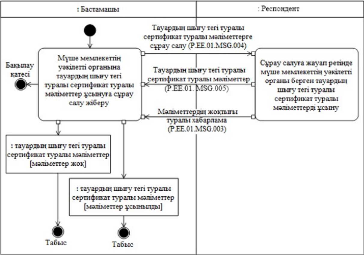
4-сурет. "Сұрау салу бойынша тауардың шығу тегі туралы сертификат туралы мәліметтерді ұсыну" (P.EE.01.TRN.005) жалпы процесінің транзакциясын орындау схемасы
