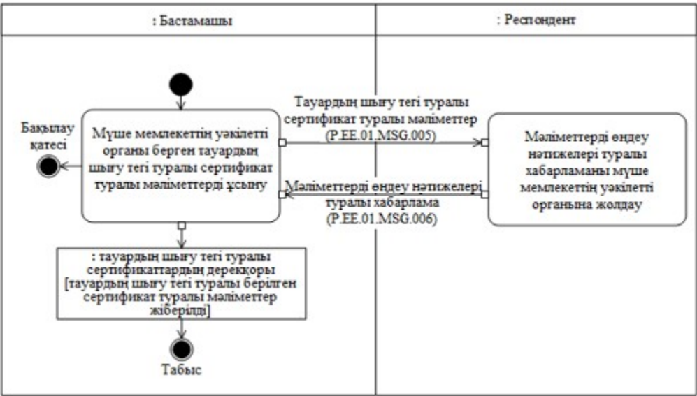
5-сурет. "Тауардың шығу тегі туралы сертификат туралы мәліметтерді ұсыну" (P.EE.01.TRN.006) жалпы процесінің транзакциясын орындау схемасы 6-кесте
