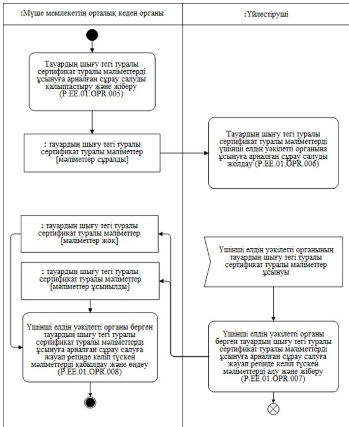
5-сурет. "Сұрау салу бойынша тауардың шығу тегі туралы сертификат туралы мәліметтерді алу" (P.EE.01.PRC.002) рәсімін орындау схемасы
