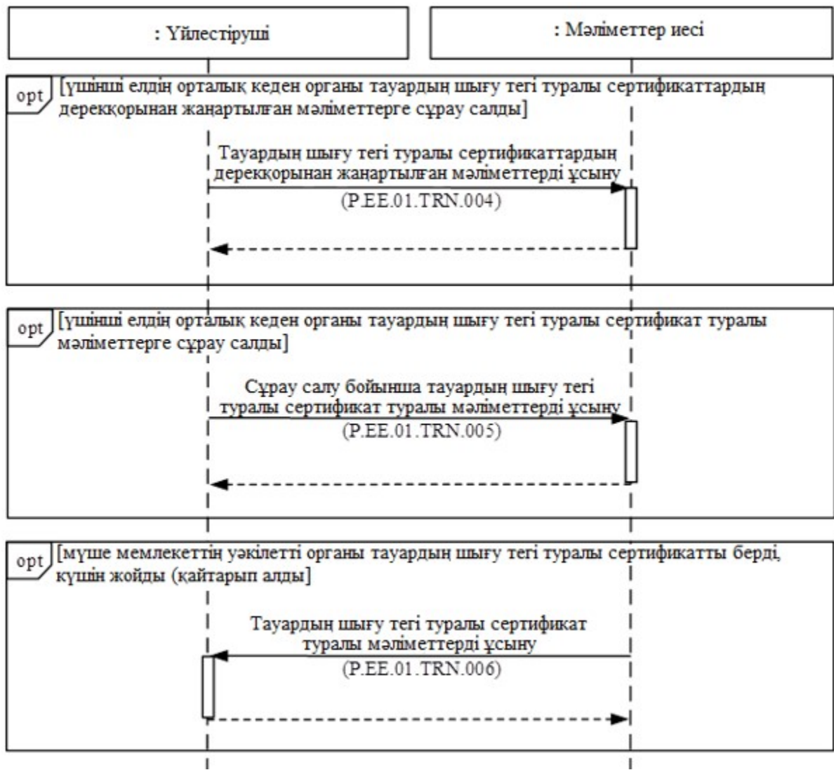
2-сурет. Тауардың шығу тегі туралы сертификаттар туралы мәліметтерді ұсыну кезінде жалпы процестің транзакцияларын орындау схемасы 2-кесте
