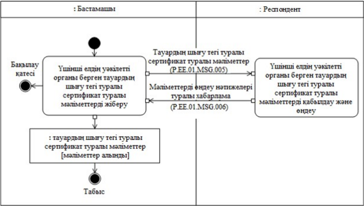
5-сурет. "Үшінші елдің уәкілетті органы берген тауардың шығу тегі туралы сертификат туралы мәліметтерді алу" (P.EE.01.TRN.003) жалпы процесінің транзакциясын орындау схемасы
