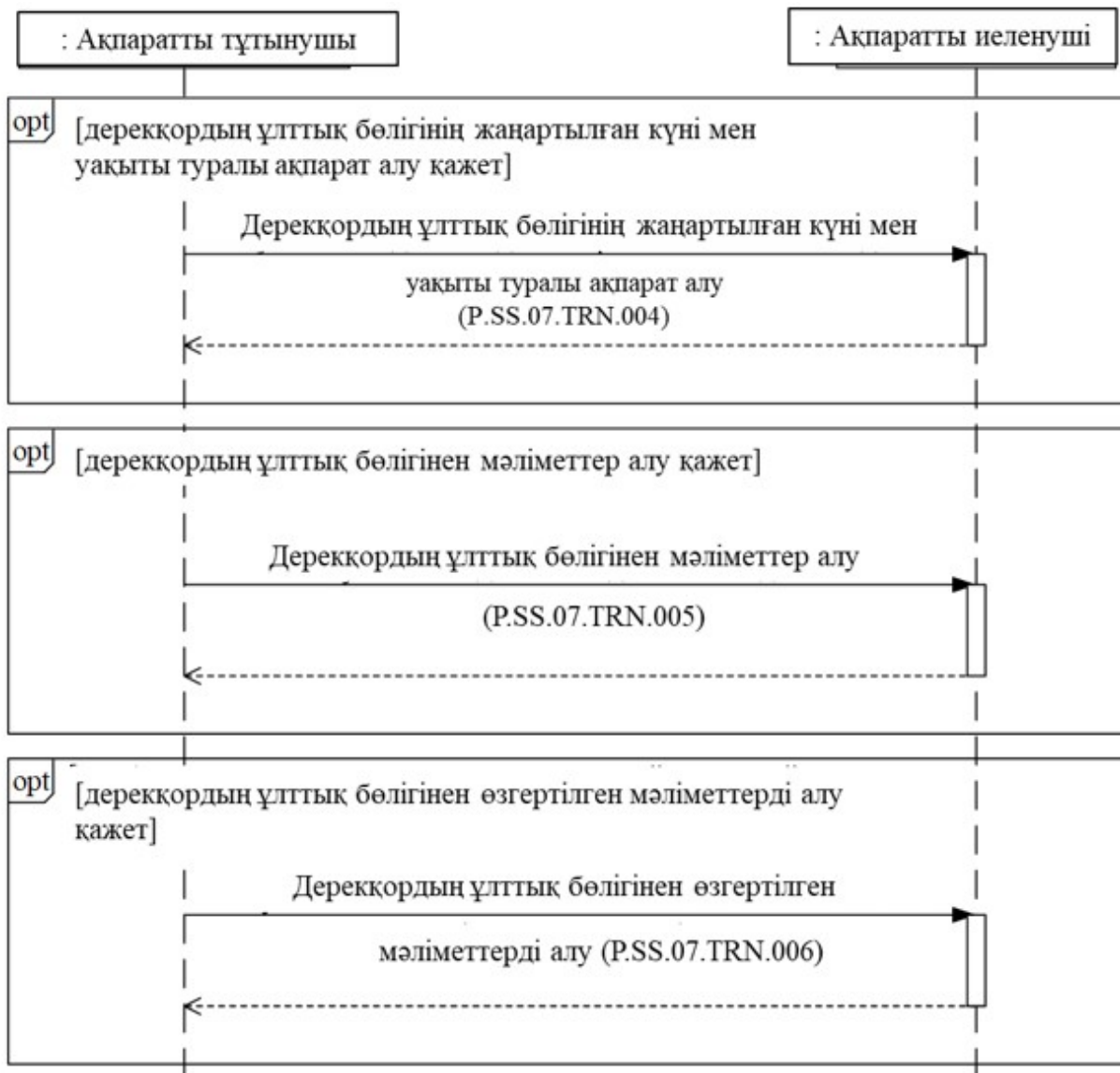
3-сурет. Дерекқордан мәліметтер алу кезіндегі жалпы процесс транзакцияларының орындалу схемасы 3-кесте
