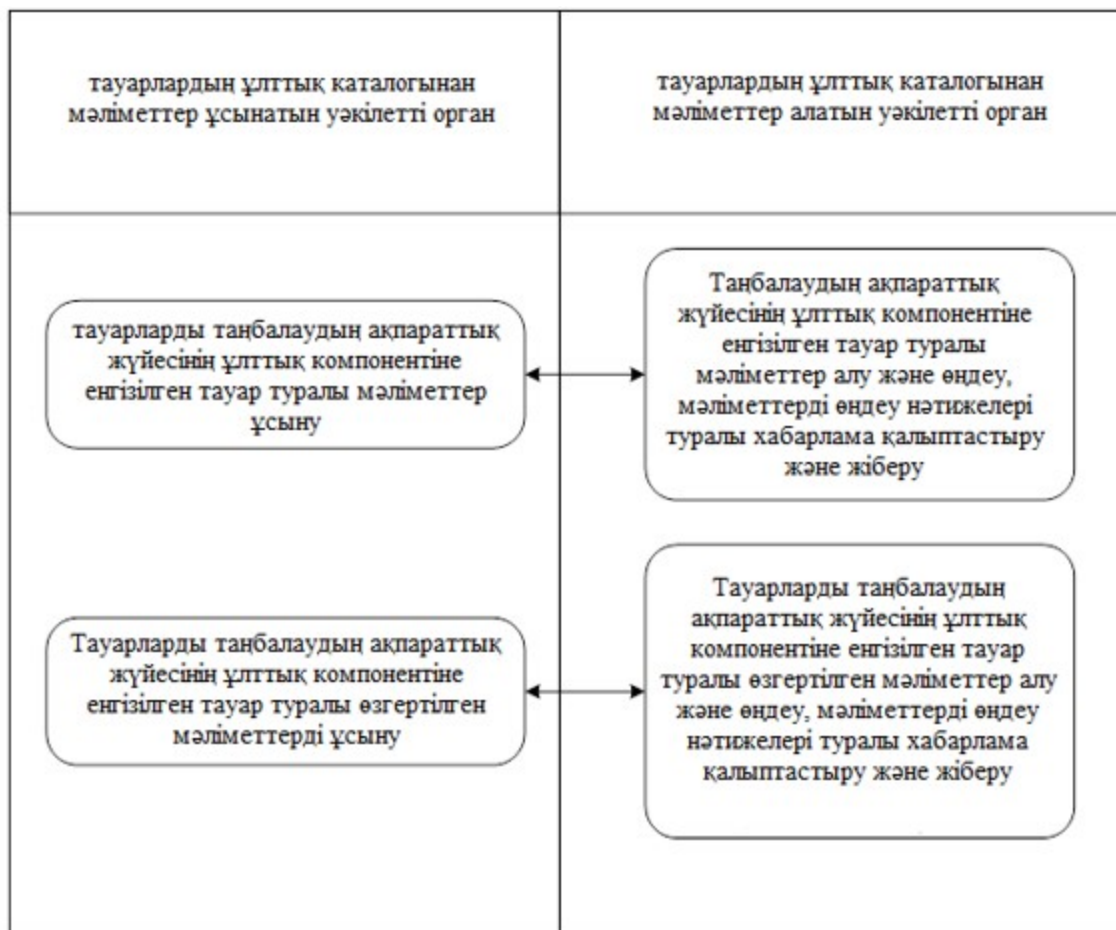
1-сурет. Тауарлардың сипаттамалары туралы мәліметтерді үндестіру мақсатында тауарлар туралы мәліметтерді ұсыну кезіндегі мүше мемлекеттердің уәкілетті органдары арасындағы ақпараттық өзара іс-қимылдың функционалдық схемасы
