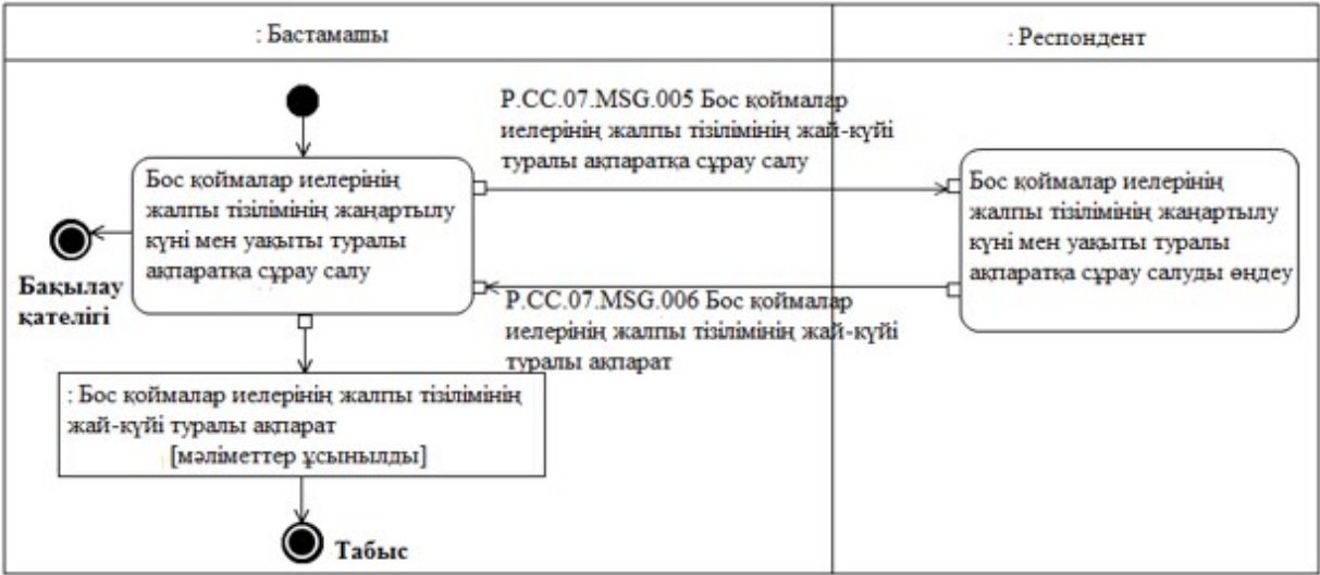
7-сурет. "Бос қоймалар иелерінің жалпы тізілімінің жаңартылу күні мен уақыты туралы ақпаратты алу" (P.CC.07.TRN.004) жалпы процесінің транзакциясын орындау схемасы 8-кесте
