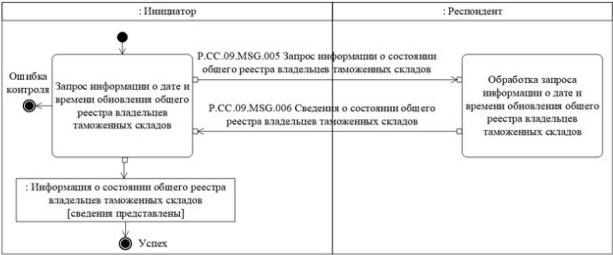
7-сурет. "Кеден қоймалары иелерінің жалпы тізілімінің жаңартылу күні мен уақыты туралы ақпарат алу" (P.CC.09.TRN.004) жалпы процесінің транзакциясын орындау схемасы 8-кесте
