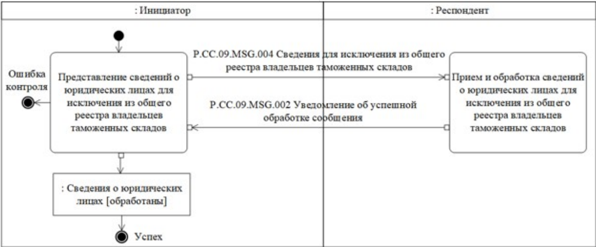
6-сурет. "Кеден қоймалары иелерінің жалпы тізілімінен заңды тұлғалар туралы мәліметтерді алып тастау" (P.CC.09.TRN.003) жалпы процесінің транзакциясын орындау схемасы
