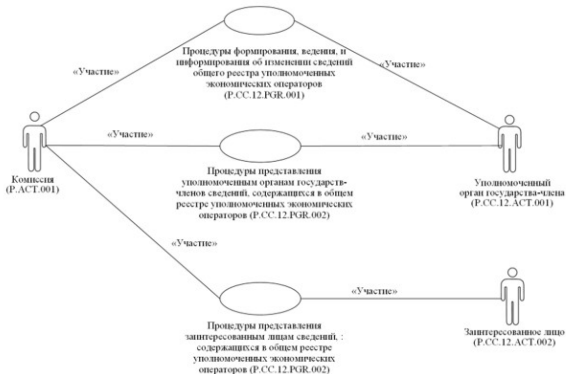
1-сурет. Жалпы процесс құрылымы
