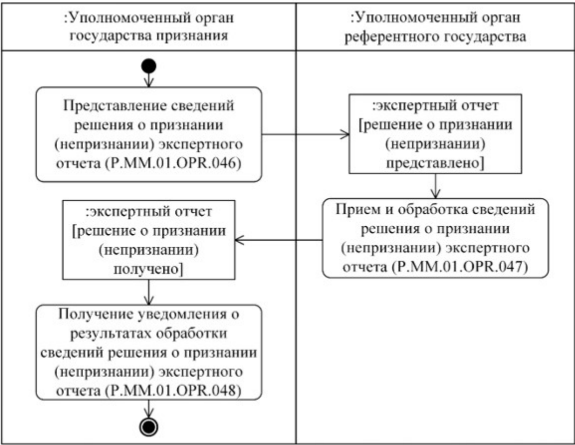
30-сурет. "Сарапшылық есепті тану (танымау) туралы шешімді жіберу" (P.MM.01.PRC.016) рәсімін орындау схемасы
