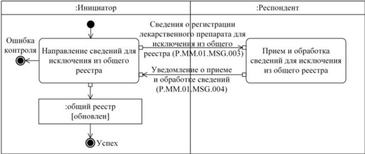
7-сурет. Схема выполнения транзакции общего процесса "Мәліметтерді жалпы тізілімнен алып тастау" (P.MM.01.TRN.003) жалпы процесінің транзакциясын орындау схемасы
