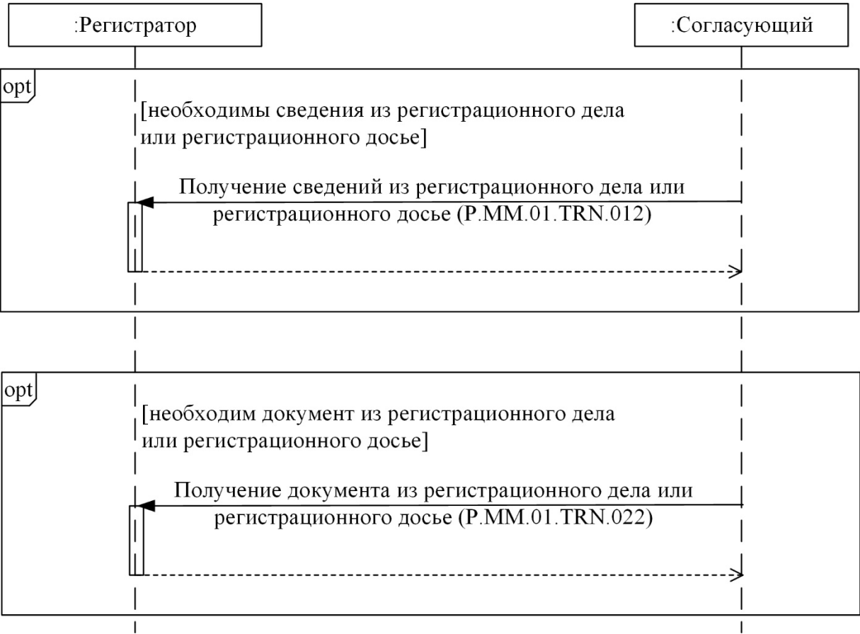
3-сурет. Тіркеу ісінде немесе тіркеу дерекнамасында қамтылған мәліметтер мен құжаттарды алған кезде жалпы процесс транзакцияларын орындау схемасы 3-кесте
