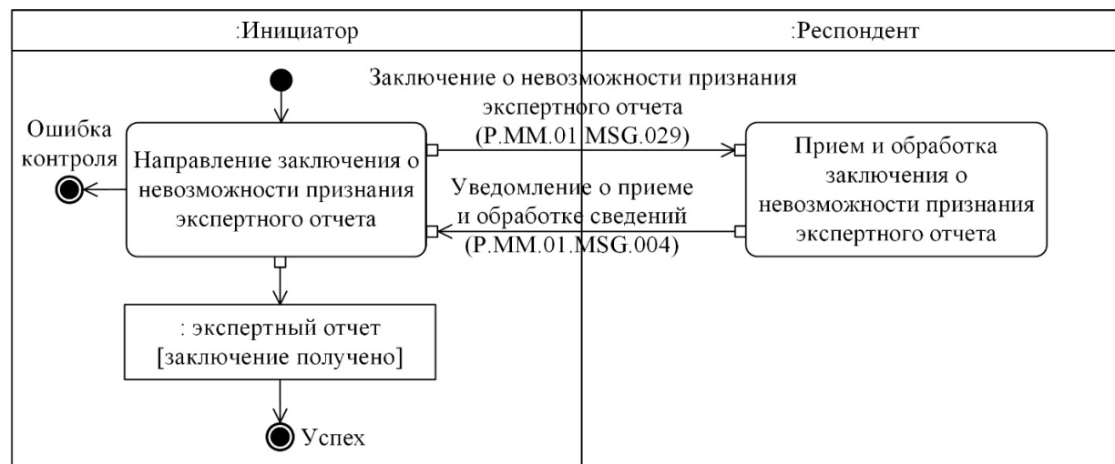
16-сурет. "Сарапшылық есепті танудың мүмкін еместігі туралы қорытынды жіберу" (P.MM.01.TRN.020) жалпы процесі транзакциясын орындау схемасы
