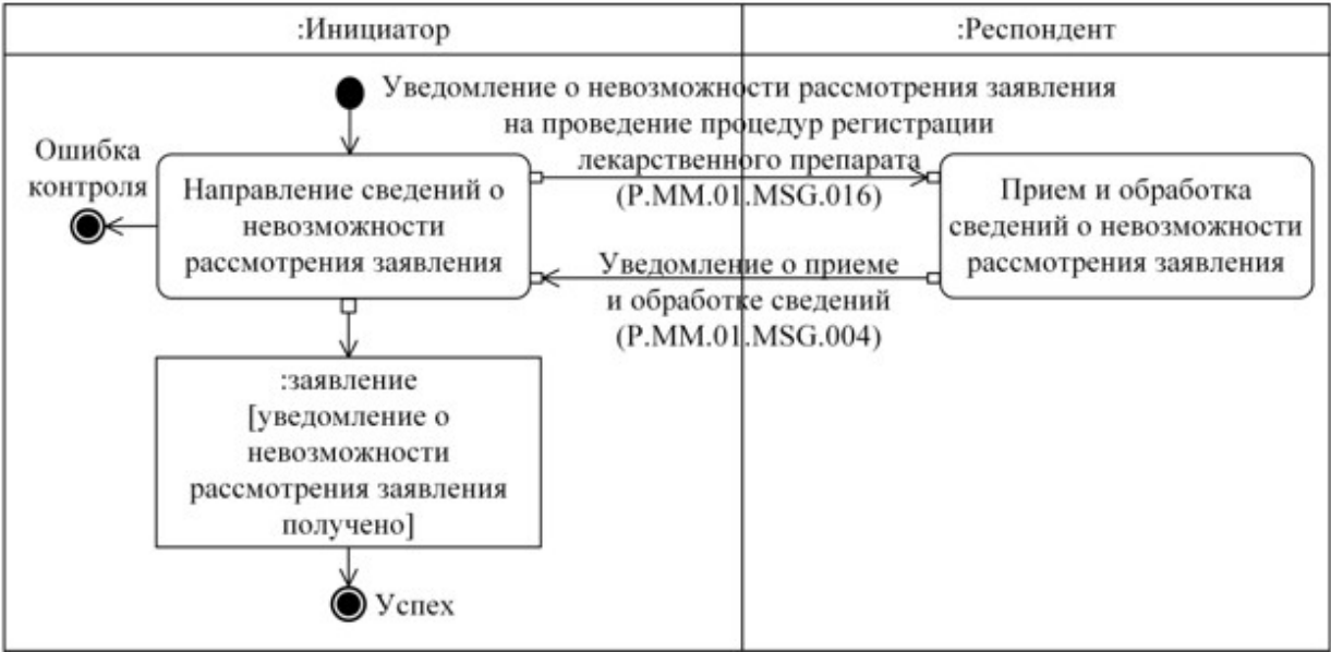
7-сурет. "Дәрілік препаратты тіркеу рәсімдерін жүргізуге өтінішті қараудың мүмкін еместігі туралы хабарлама" (P.MM.01.TRN.010) жалпы процесінің транзакциясын орындау схемасы
