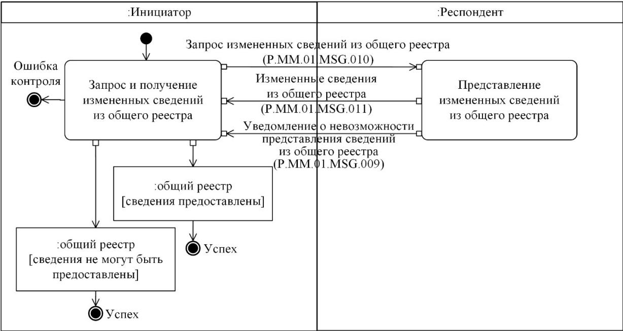
10-сурет. "Жалпы тізілімнен өзгертілген мәліметтерді алу" (P.MM.01.TRN.006) жалпы процесі транзакциясын орындау схемасы 11-кесте
