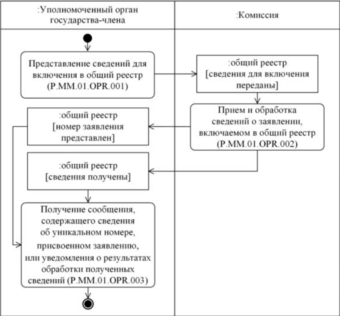
9-сурет. "Мәліметтерді жалпы тізілімге енгізу" (P.MM.01.PRC.001) рәсімін орындау схемасы
