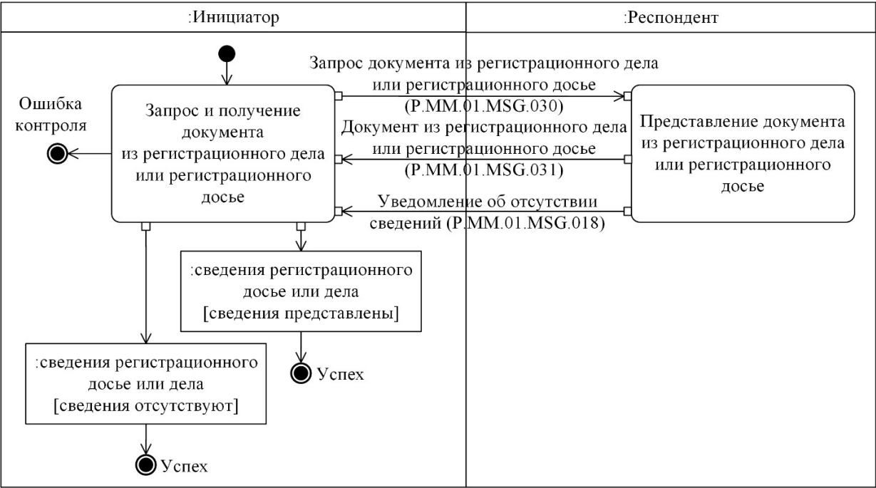
17-сурет. "Комиссияның тіркеу ісінен немесе тіркеу дерекнамасынан құжат алуы" ( P.MM.01.TRN.021) жалпы процесі транзакциясын орындау схемасы 18-кесте
