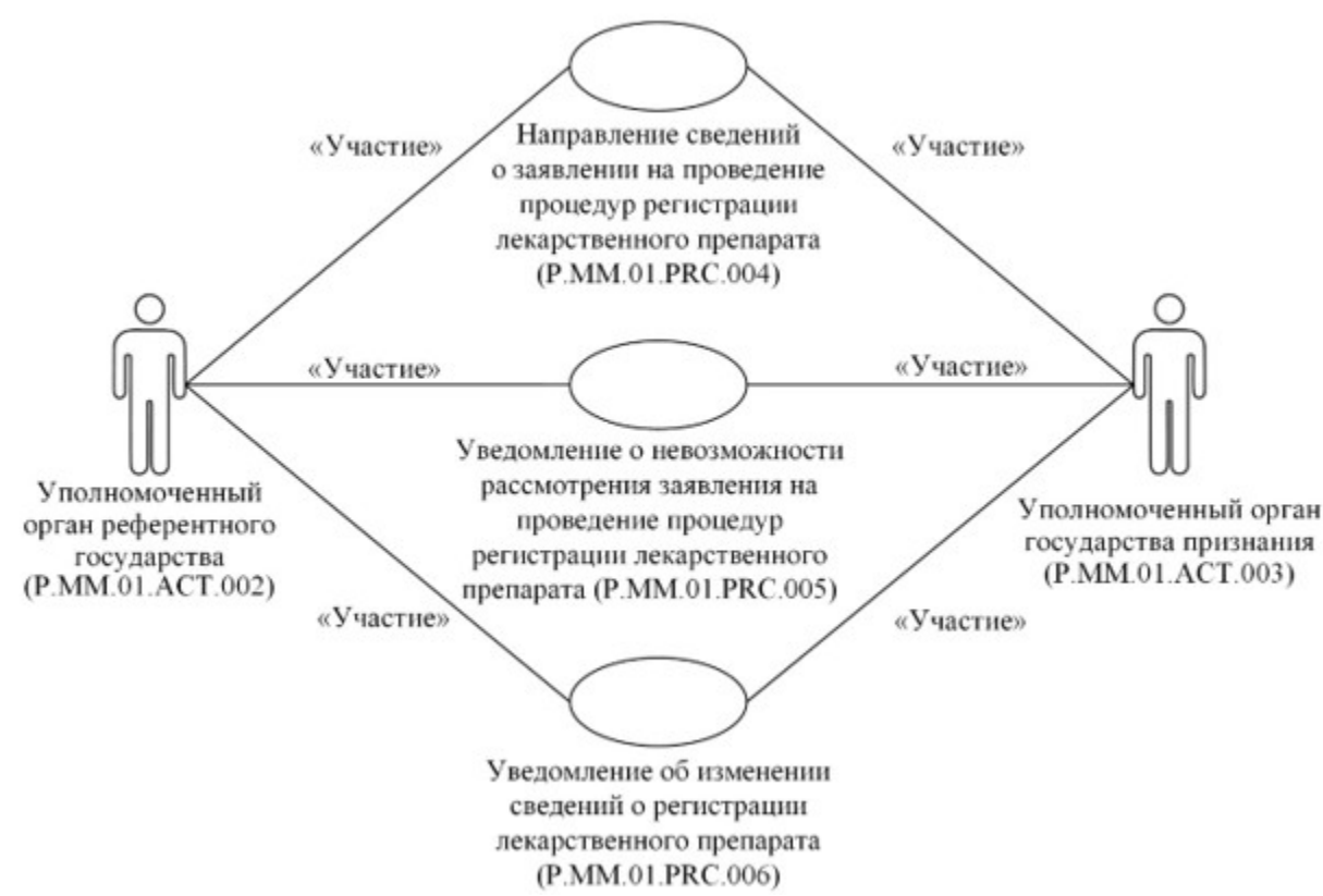
3-сурет. "Дәрілік препараттың тіркелгені туралы мәліметтерді жіберу және дәрілік препаратты тіркеу рәсімдерін жүргізуге арналған өтініш туралы мәліметтерді қарау рәсімдері" (P.MM.01.PGR.002) рәсімдер тобының жалпы схемасы
