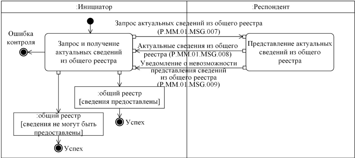
9-сурет. "Жалпы тізілімнен өзекті мәліметтер алу" (P.MM.01.TRN.005) жалпы процесі транзакциясын орындау схемасы 10-кесте
