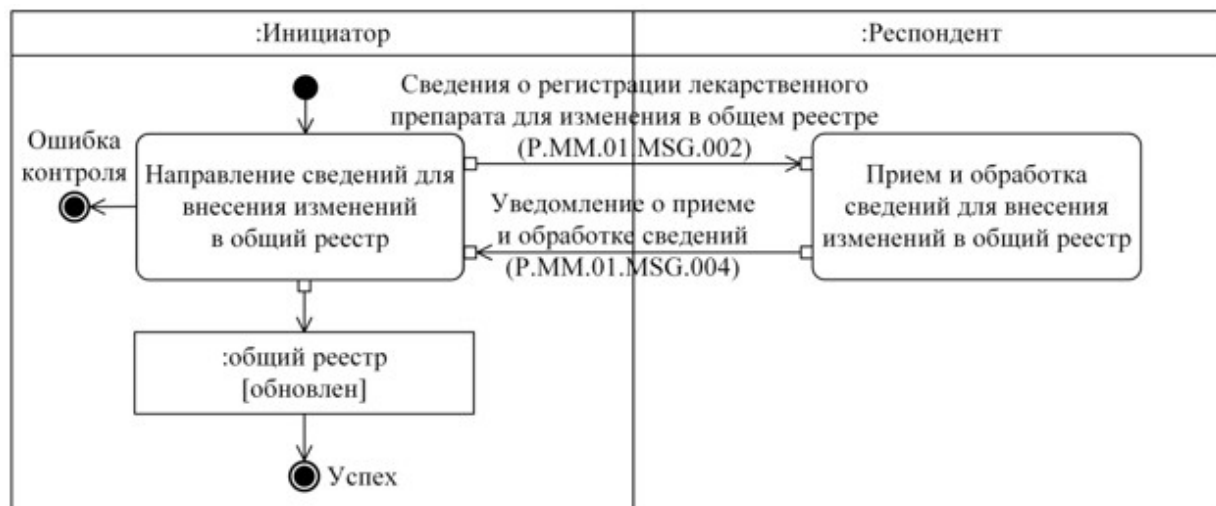
6-сурет. "Жалпы тізілімде қамтылған мәліметтерді өзгерту" (P.MM.01.TRN.002) жалпы процесінің транзакциясын орындау схемасы
