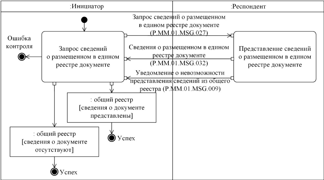
14-сурет. "Бірыңғай тізілімде орналастырылған құжат туралы мәліметтерді алу" ( Р.ММ.01.TRN.018) жалпы процесі транзакциясын орындау схемасы 15-кесте
