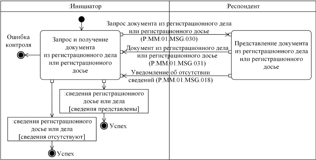
14-сурет. "Тіркеу ісінен немесе тіркеу дерекнамасынан құжат алу" (P.MM.01.TRN.022) жалпы процесі транзакциясын орындау схемасы 15-кесте
