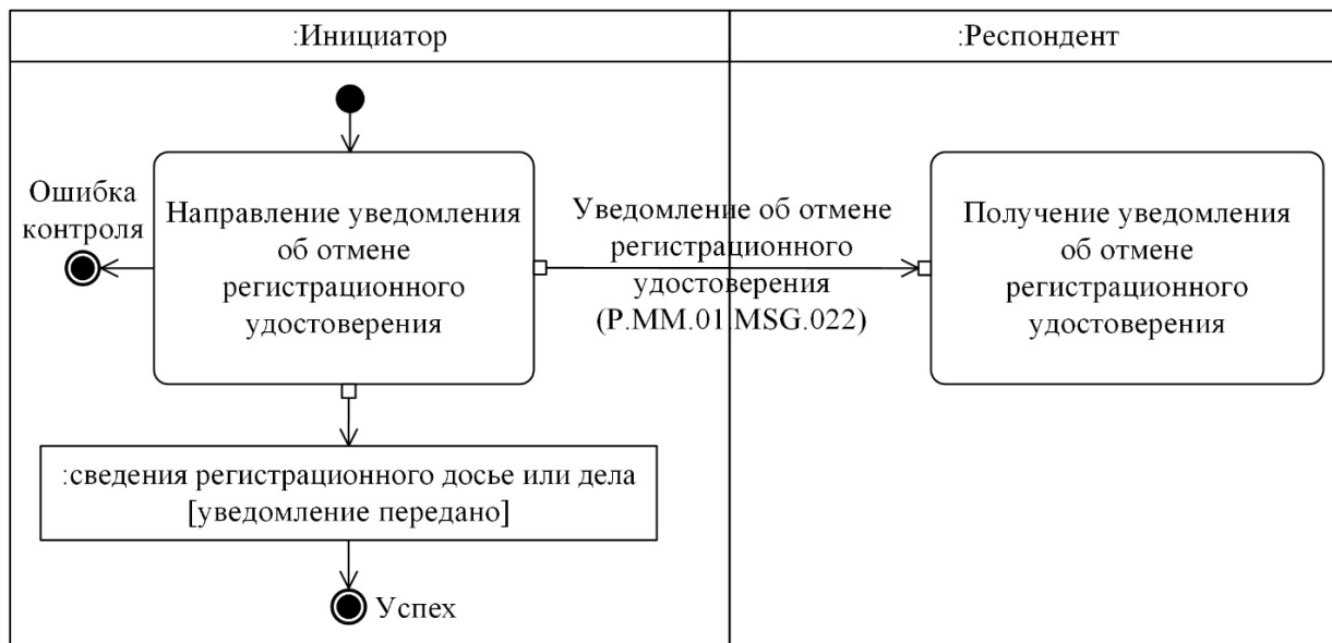
10-сурет. "Тіркеу куәлігін жою туралы хабарлама жіберу" (P.MM.01.TRN.013) жалпы процесі транзакциясын орындау схемасы 11-кесте
