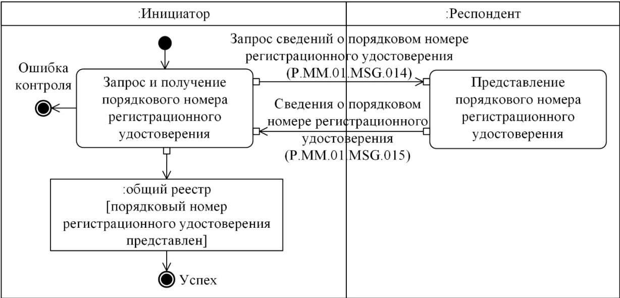
11-сурет. "Тіркеу куәлігінің реттік нөмірін алу" (P.MM.01.TRN.007) жалпы процесі транзакциясын орындау схемасы 12-кесте
