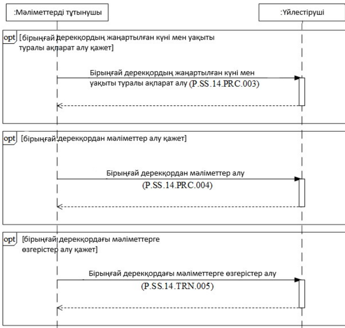
3-сурет. Бірыңғай дерекқордан мәліметтер алу кезінде жалпы процестің транзакцияларын орындау схемасы
