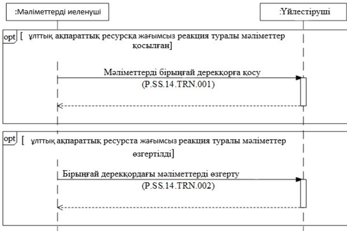
2-сурет. Бірыңғай дерекқорды қалыптастыру және жүргізу кезіндегі жалпы процестің транзакцияларын орындау схемасы 2-кесте
