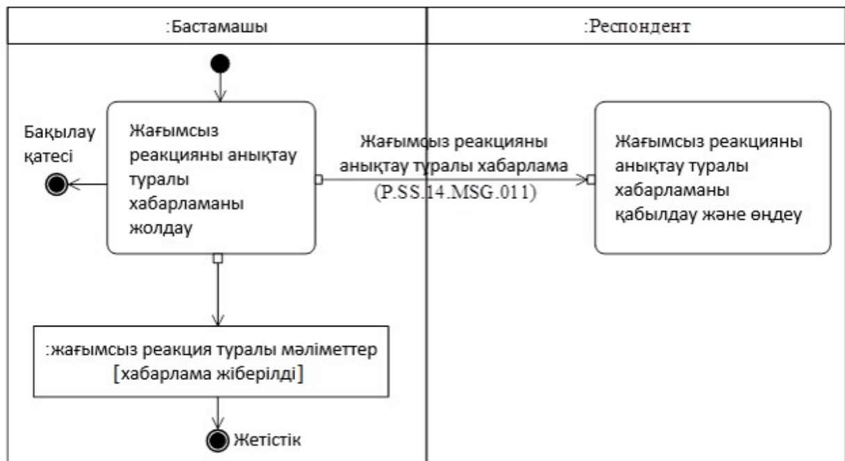
3-сурет. "Жағымсыз реакцияны анықтау туралы хабарлама" (P.SS.14.TRN.006) жалпы процесс транзакциясын орындау схемасы 4-кесте
