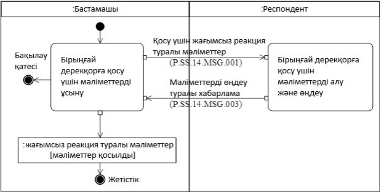
4-сурет. "Мәліметтерді бірыңғай дерекқорға қосу" (P.SS.14.TRN.001) жалпы процесінің транзакциясын орындау схемасы 5-кесте
