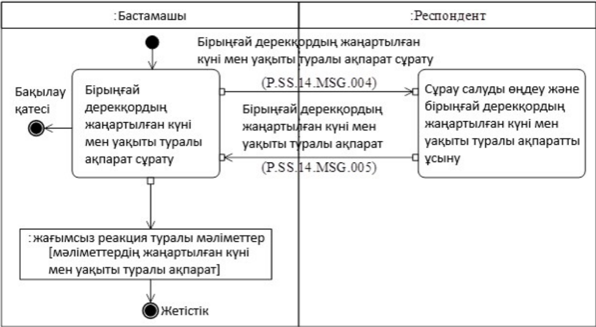
6-сурет. "Бірыңғай дерекқордың жаңартылған күні мен уақыты туралы ақпарат алу" (P.SS.14.TRN.003) жалпы процесс транзакциясын орындау схемасы 7-кесте
