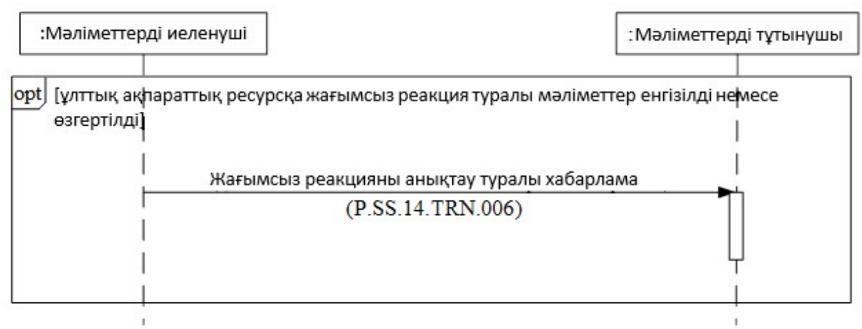
2-сурет. Уәкілетті органдарды хабардар ету кезіндегі жалпы процестің транзакцияларын орындау схемасы
