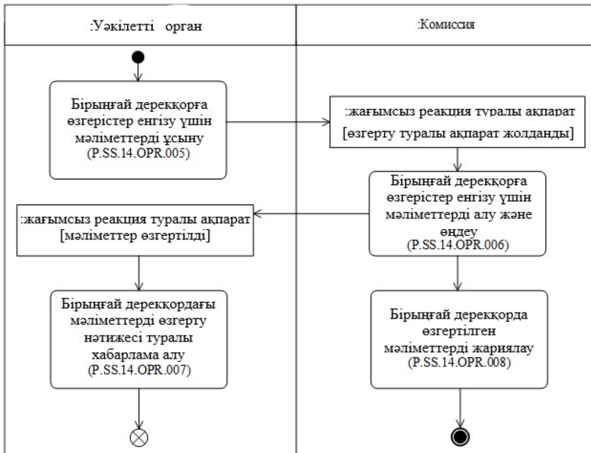
6-сурет. "Бірыңғай дерекқорда мәліметтерді өзгерту" (P.SS.14.PRC.002) рәсімін орындау схемасы
