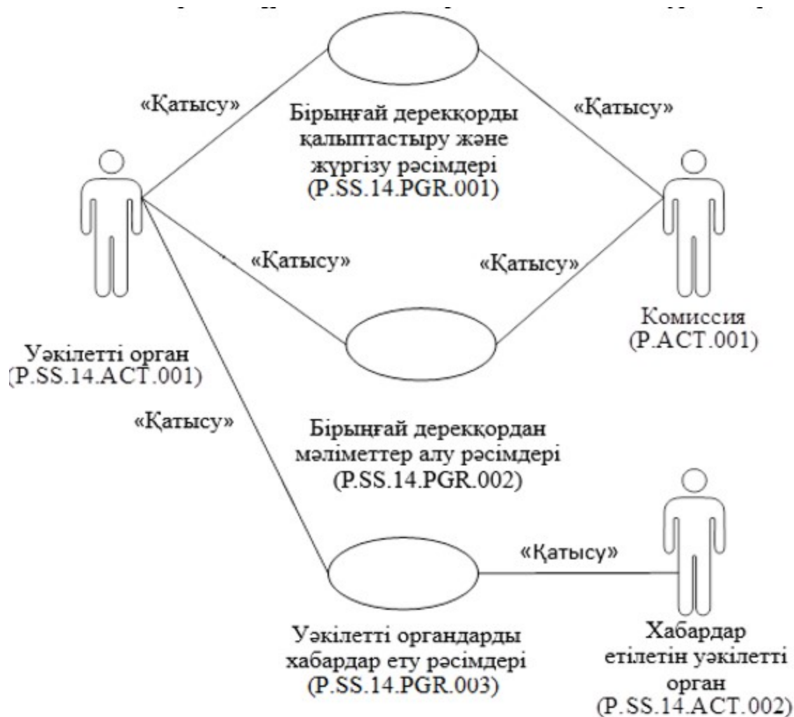
1-сурет. Жалпы процестің құрылымы
