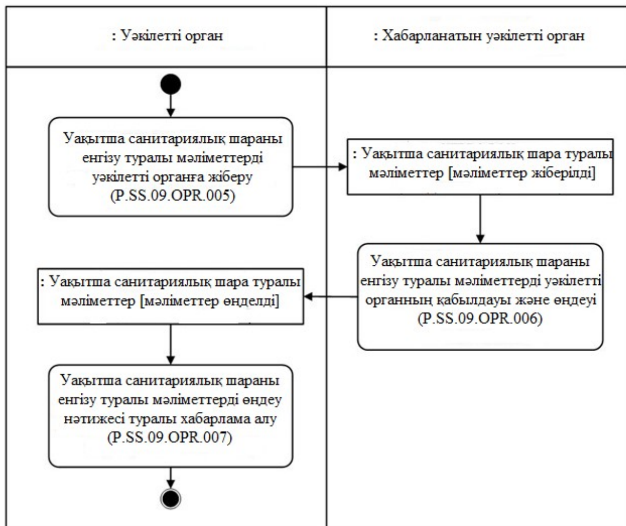
Рис. 7. "Уақытша санитариялық шараны енгізу туралы мәліметтерді уәкілетті органға ұсыну" (P.SS.09.PRC.002) рәсімін орындау схемасы
