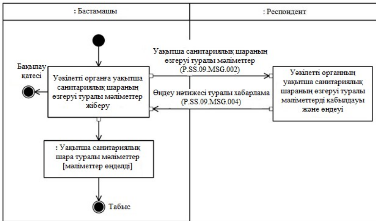
6-сурет. "Уақытша санитариялық шараның өзгеруі туралы мәліметтерді уәкілетті органға ұсыну" (P.SS.09.TRN.009) жалпы процесінің транзакциясын орындау схемасы 7-сурет
