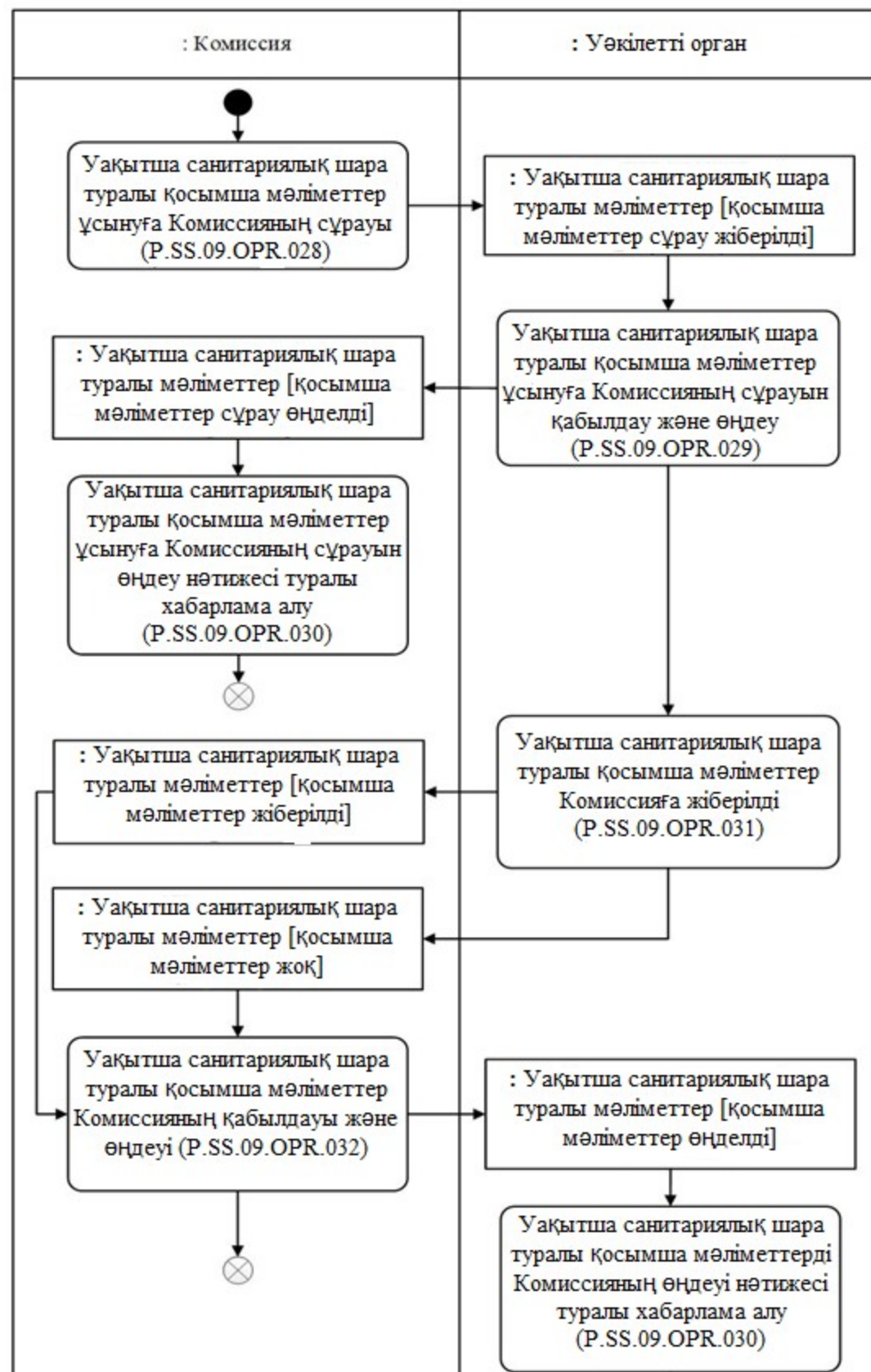
14-сурет. "Уақытша санитарлық шара туралы қосымша мәліметтерді Комиссияға ұсыну" (P. SS.09.PRC.009) рәсімін орындау схемасы
