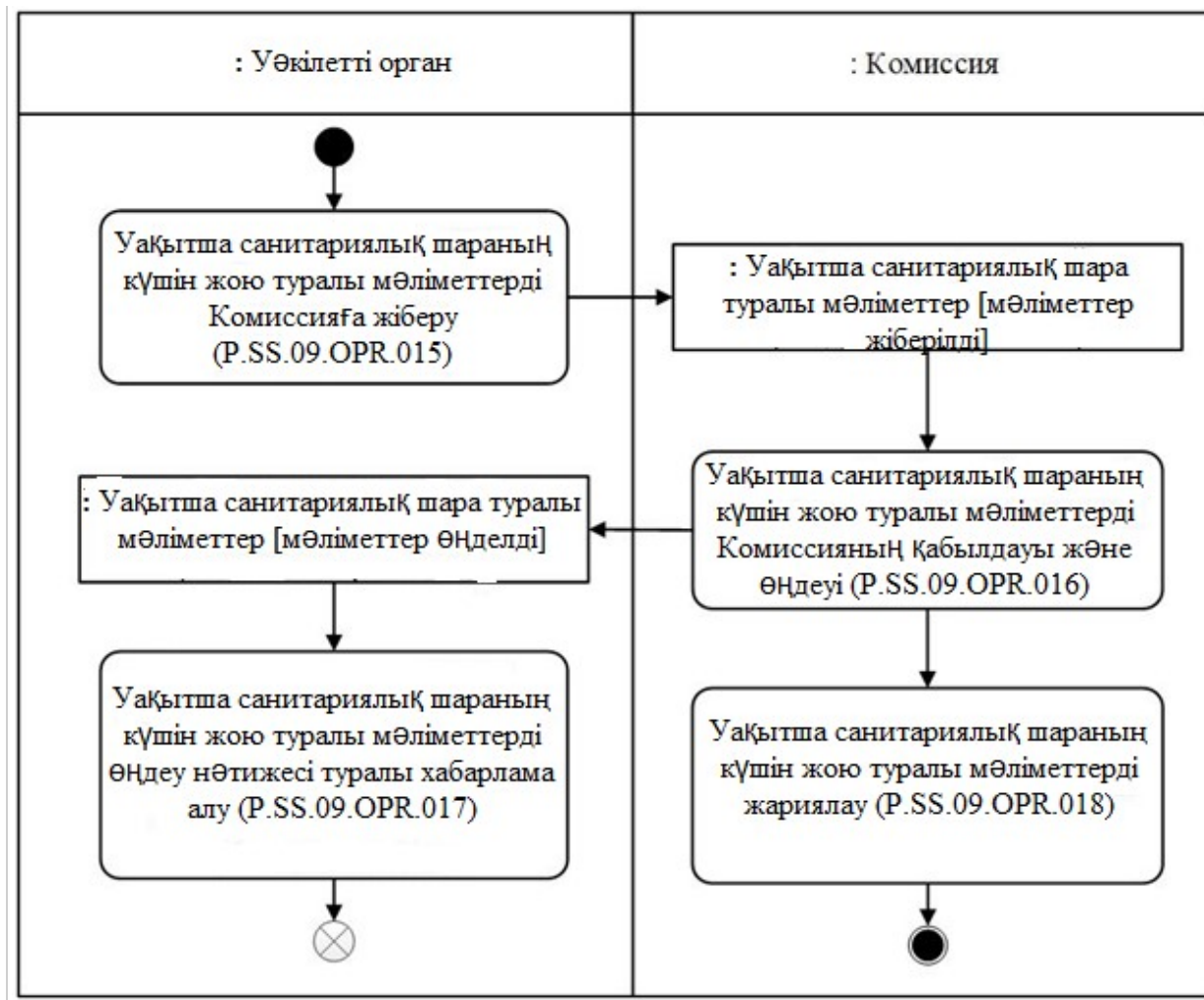
10-сурет. "Уақытша санитариялық шараның күшін жою туралы мәліметтерді комиссияға ұсыну" (P. SS.09.PRC.005) рәсімін орындау схемасы
