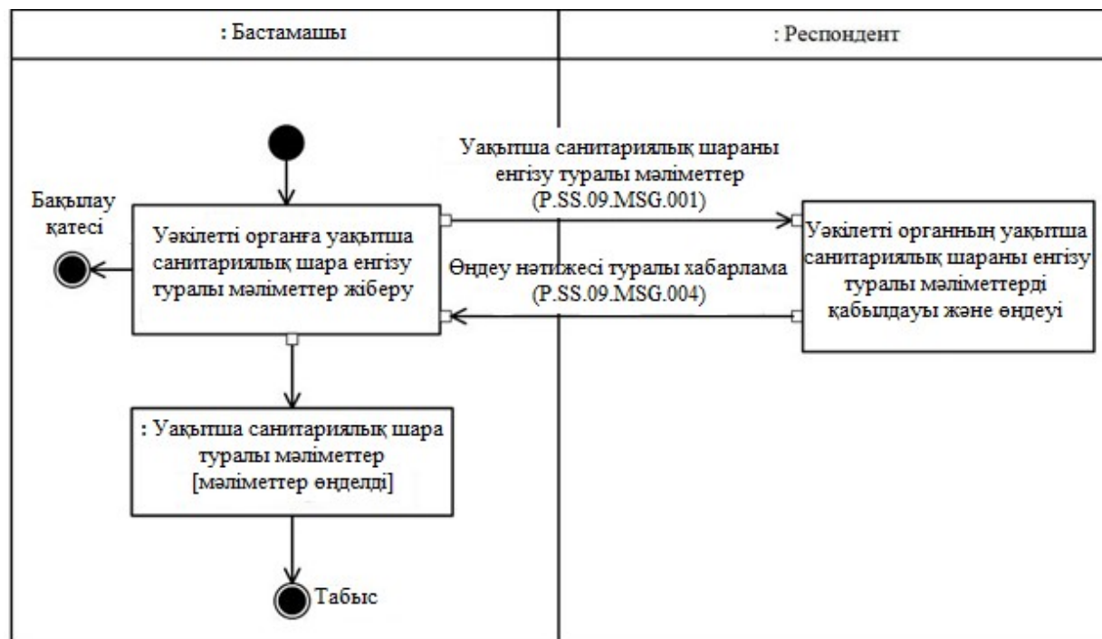
5-сурет. "Уақытша санитариялық шараны енгізу туралы мәліметтерді уәкілетті органға ұсыну" (P.SS.09.TRN.008) жалпы процесінің транзакциясын орындау схемасы 6-кесте
