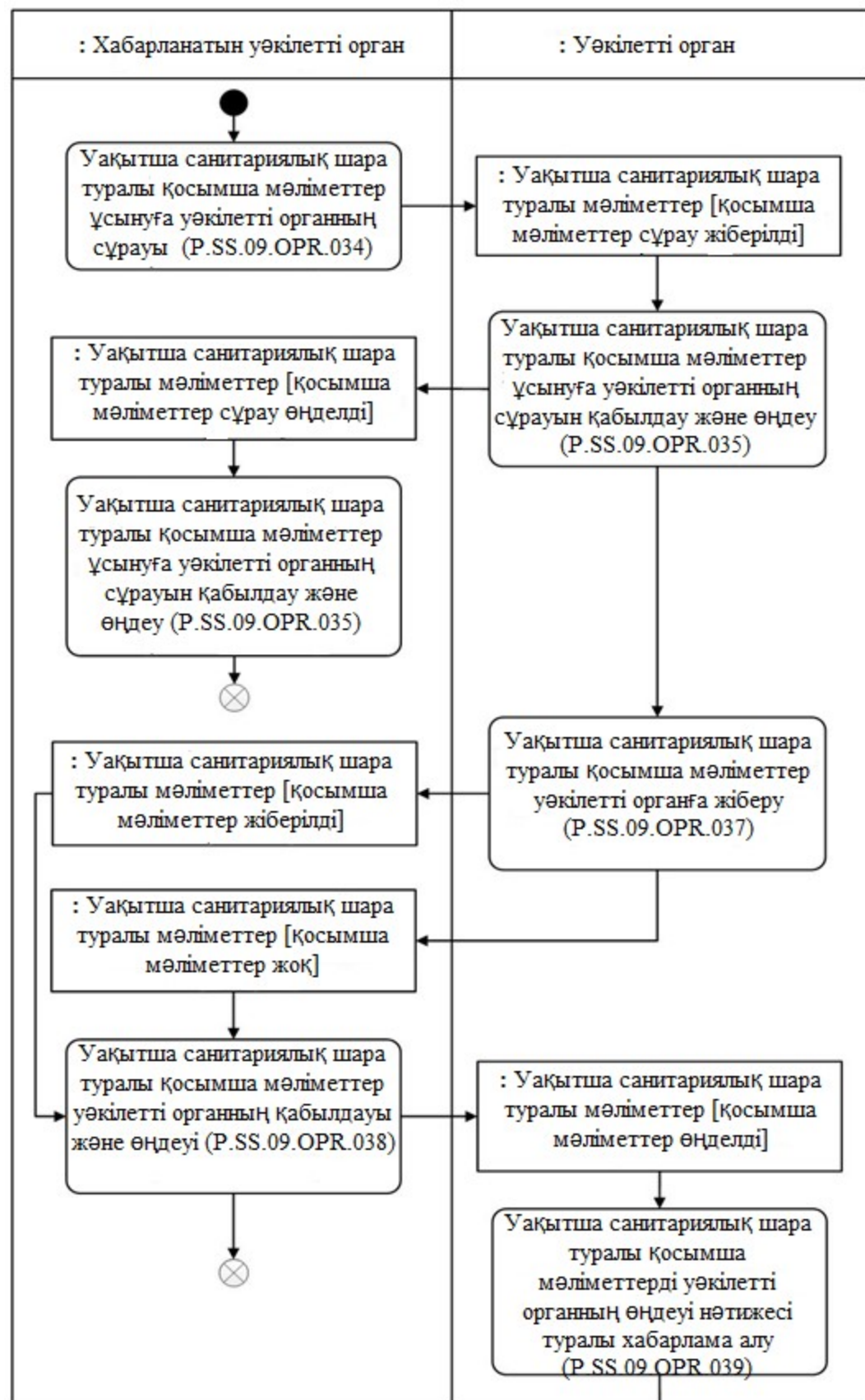
15-сурет. "Уақытша санитарлық шара туралы қосымша мәліметтерді уәкілетті органға ұсыну" (P. SS.09.PRC.010) рәсімін орындау схемасы
