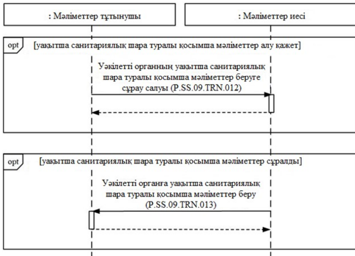
4-сурет. Уәкілетті орган уақытша санитариялық шара туралы қосымша мәліметтер алған кездегі жалпы процестің транзакцияларын орындау схемасы 4-кесте
