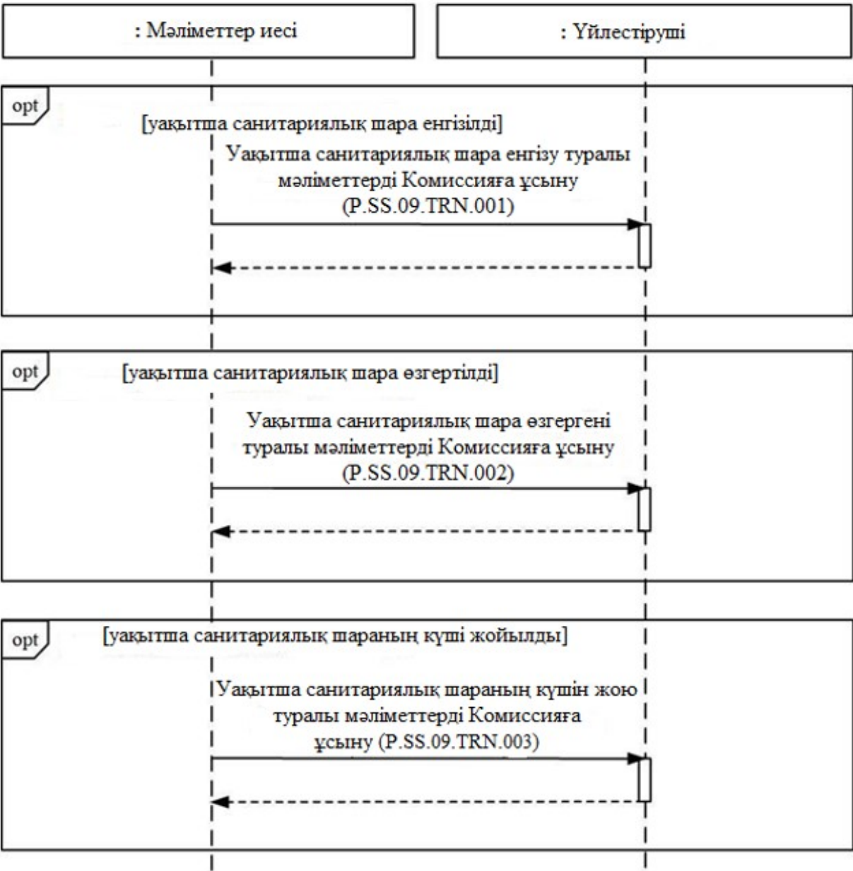
2-сурет. Уақытша санитариялық шара туралы мәліметтерді Комиссияға ұсыну кезіндегі жалпы процестің транзакцияларын орындау схемасы 2-кесте
