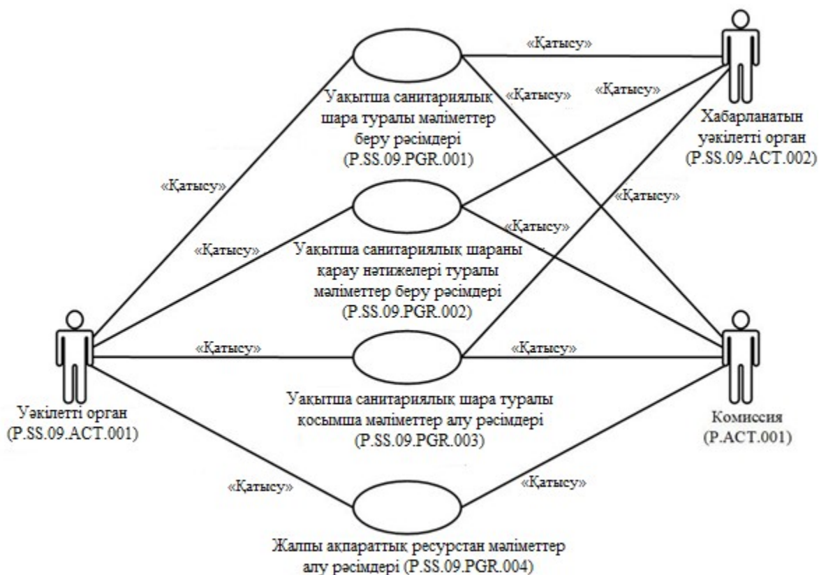
1-сурет. Жалпы процестің құрылымы
