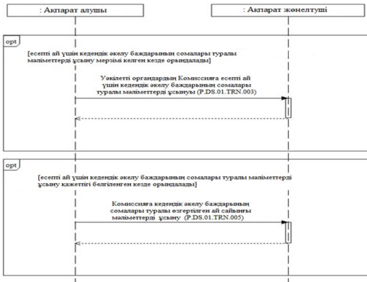
2-сурет. Уәкілетті органдар Комиссияға мәліметтер берген кездегі жалпы процесс транзакцияларын орындау схемасы 2-кесте
