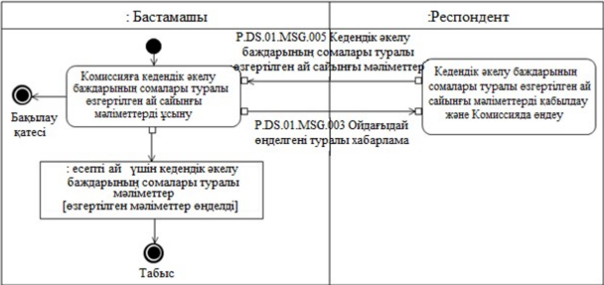
4-сурет. "Комиссияға кедендік әкелу баждарының есепті ай үшін сомалары туралы ай сайынғы өзгертілген мәліметтерді беру" (P.DS.01.TRN.005) жалпы процесінің транзакциясын орындау схемасы
