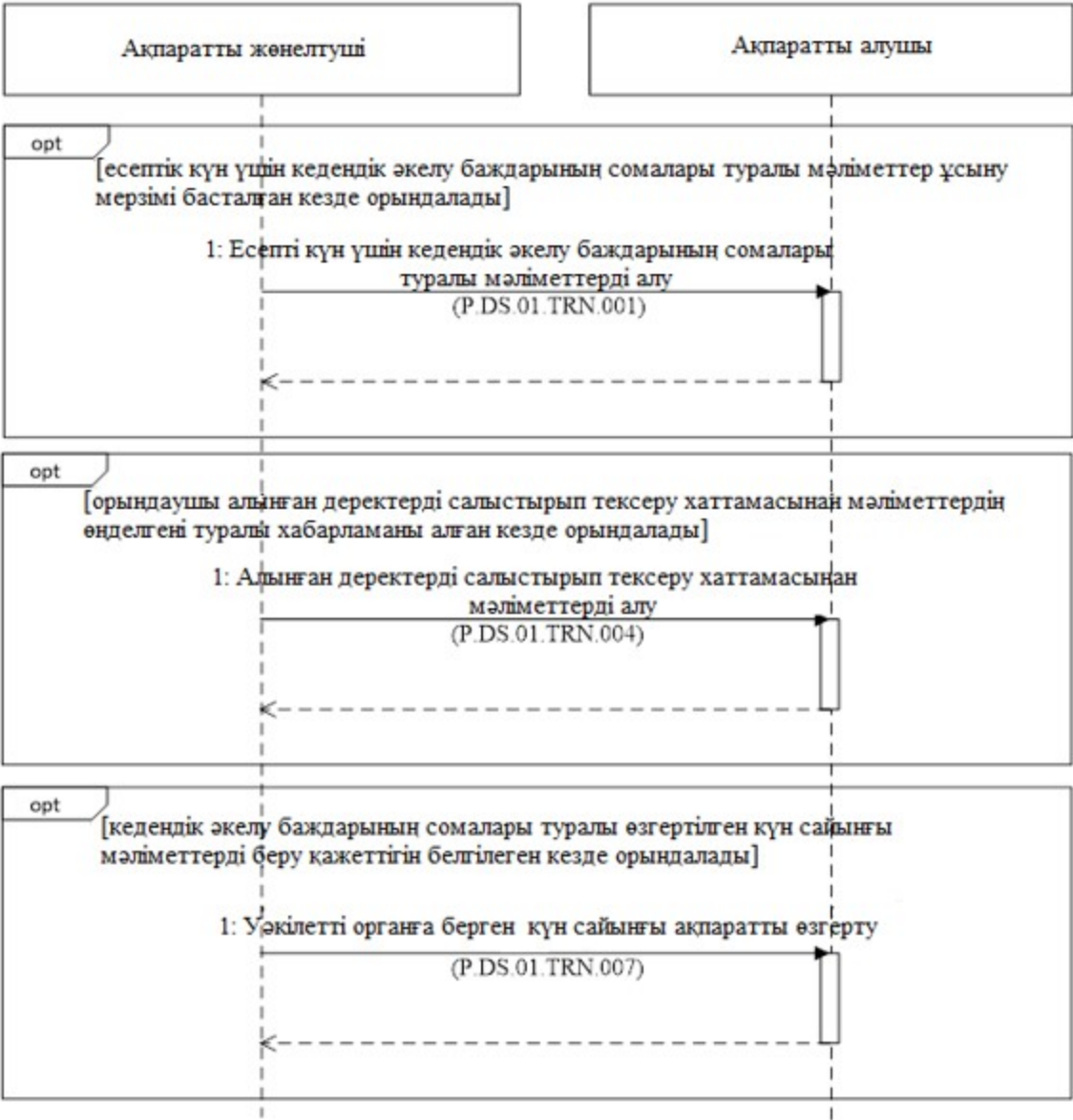
2-сурет. Уәкілетті органдар бір біріне мәліметтерді берген кездегі жалпы процесс транзакцияларын орындау схемасы
