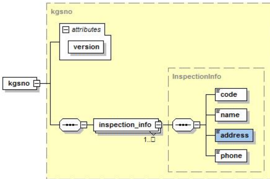
Сурет. KGSNO анықтамалығы файлының сызбасы.
