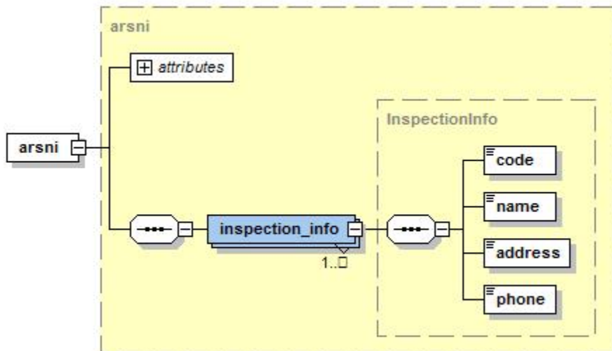
5.3.1-сурет. ARSNI анықтамалық файлының сызбасы.
