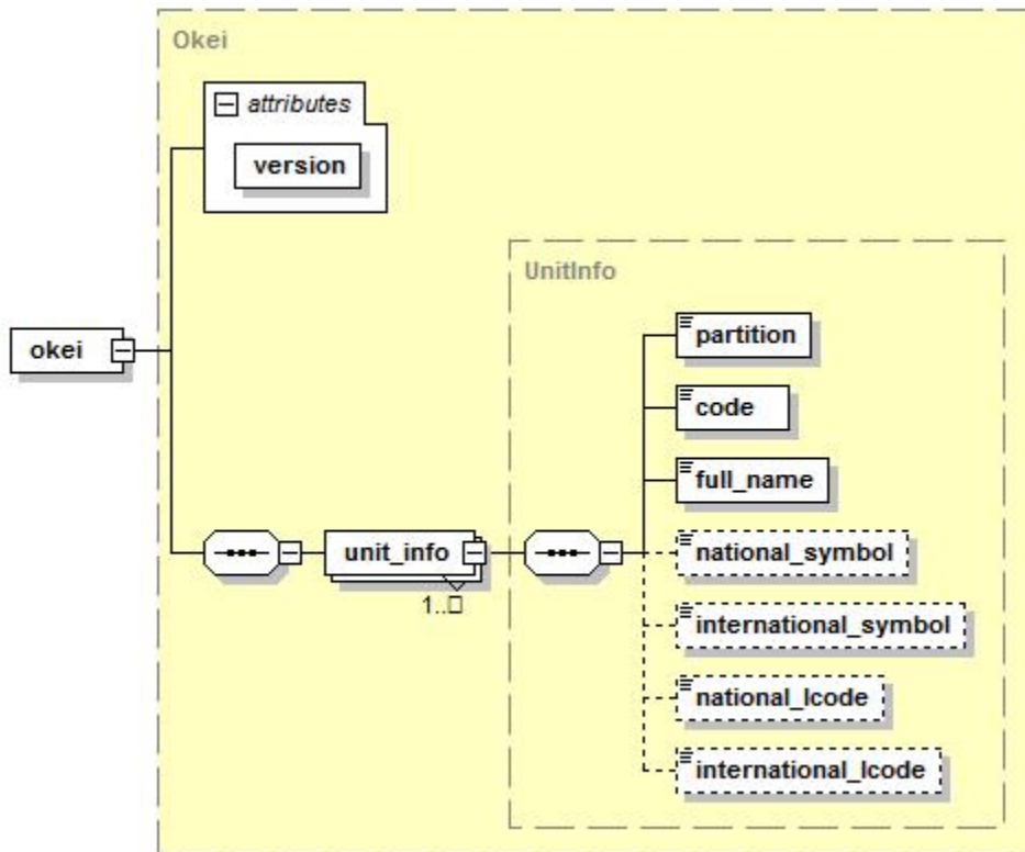
5.7.1-сурет. ӨБЖС анықтамалығы файлының сызбасы
