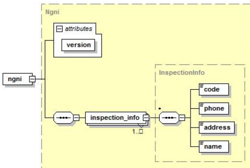
5.1.1-сурет. NGNI анықтамалық файлының сызбасы.
