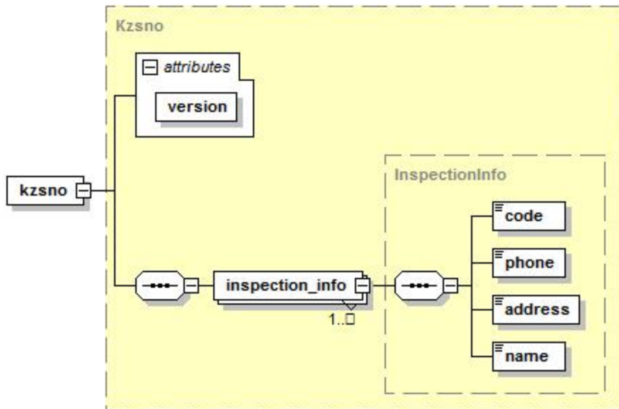
5.2.1-сурет. KZSNO анықтамалық файлының сызбасы.
