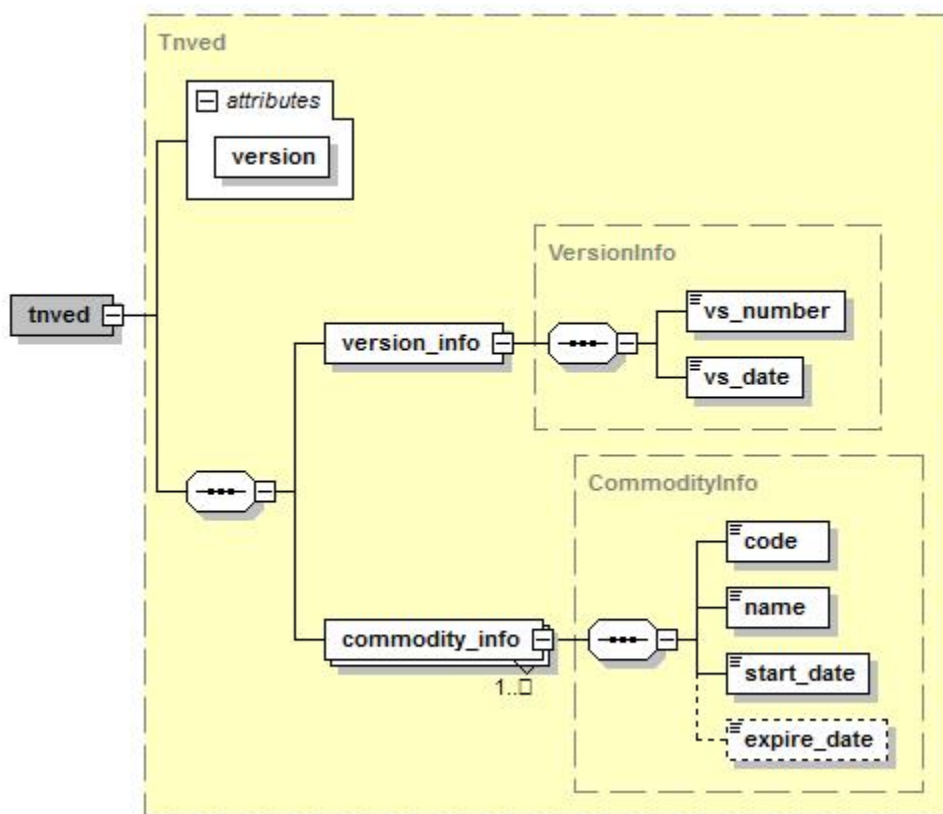
5.10.1-сурет. СЭҚ ТН анықтамалық файлының сызбасы.
