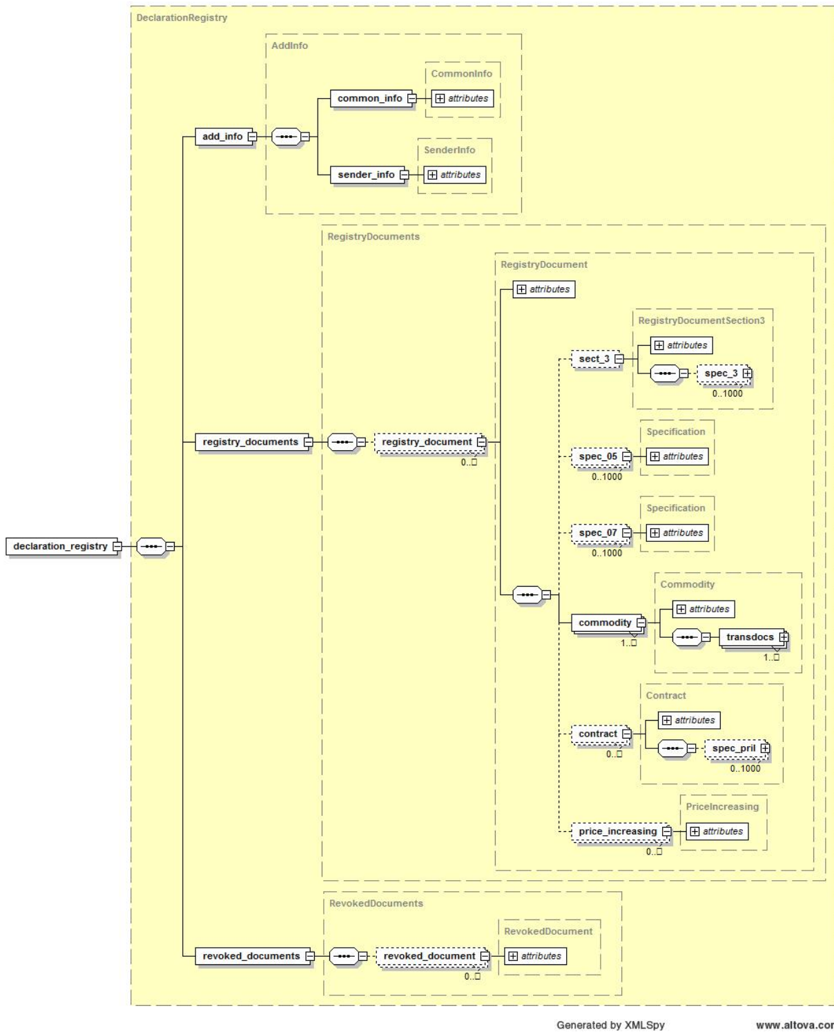
2.3.1-сурет. Өтініштер тізілімі файлының сызбасы.
