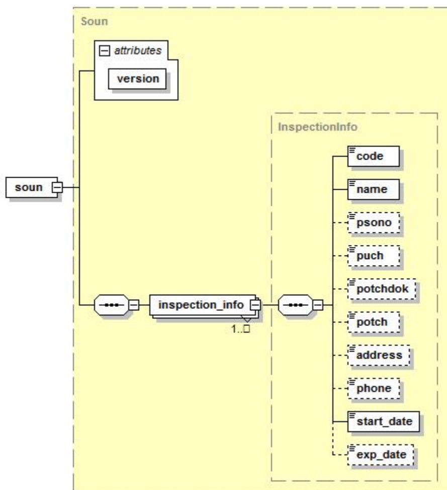
5.3.1-сурет. СЕБК анықтамалық файлының сызбасы.
