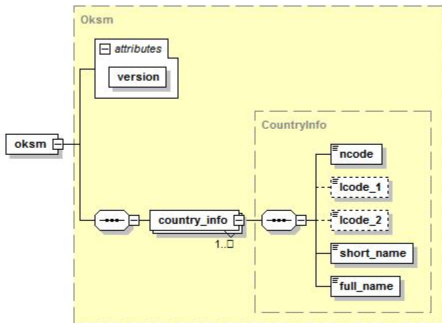
5.5.1-сурет. ӘЕЖС анықтамалығы файлының сызбасы.
