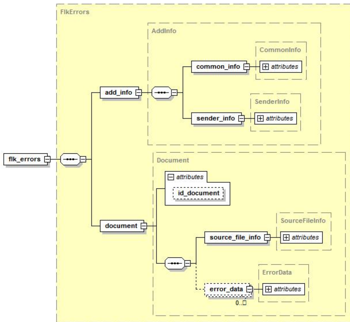
6.3.1-сурет. ФЛБ хаттамасы файлының сызбасы.
