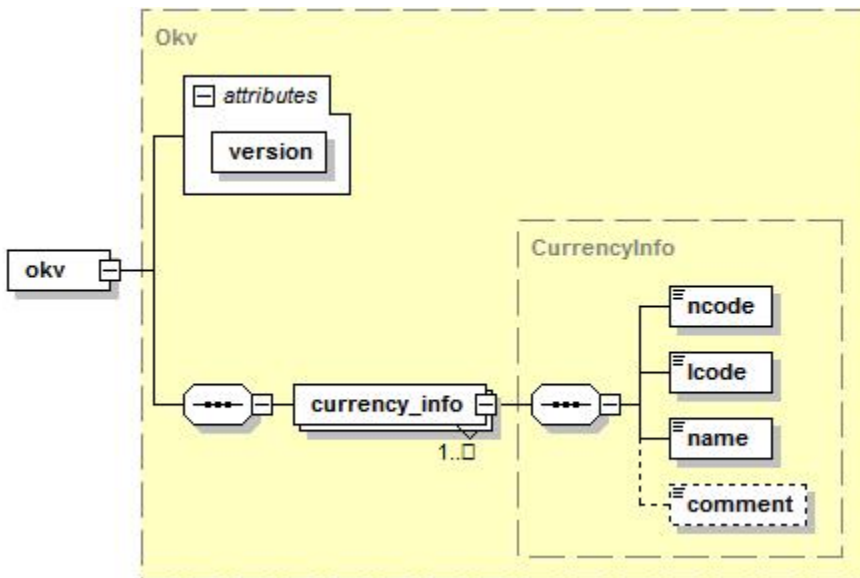
5.8.1-сурет. ВЖС анықтамалық файлының сызбасы.
