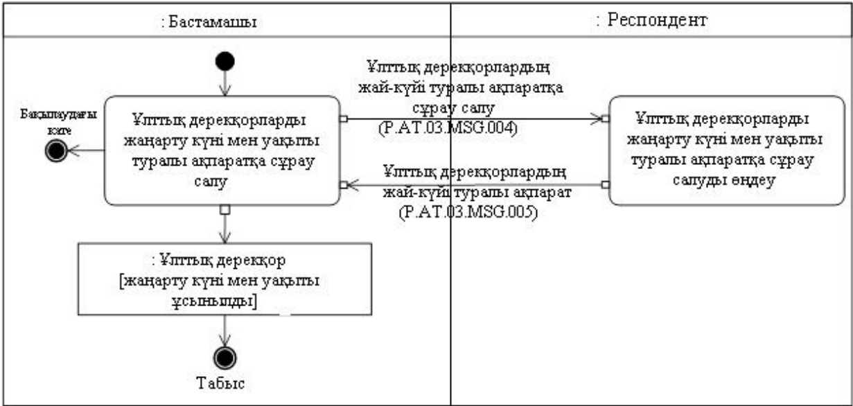
3-сурет. "Ұлттық дерекқорларды жаңарту күні мен уақыты туралы ақпарат алу" ( P.AT.03.TRN.003) жалпы процесс транзакциясын орындау схемасы 4-кесте
