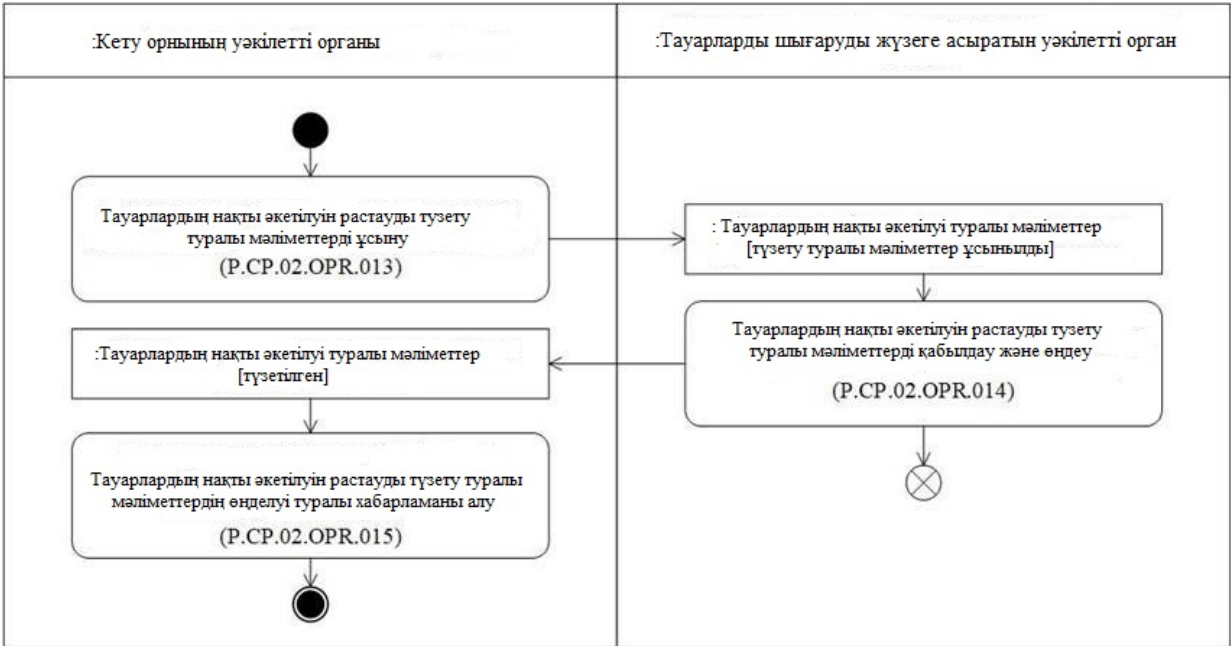
8-сурет. "Тауарлардың нақты әкетілуі туралы мәліметтерді түзету" (P.CP.02.PRC.005) рәсімін орындау схемасы.
