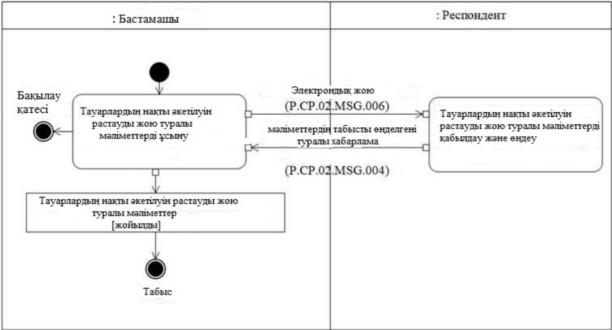
8-сурет. "Тауарлардың нақты әкетілуі туралы мәліметтерді жою" (P.CP.02.TRN.003) жалпы процесс транзакцияларын орындау схемасы 9-кесте
