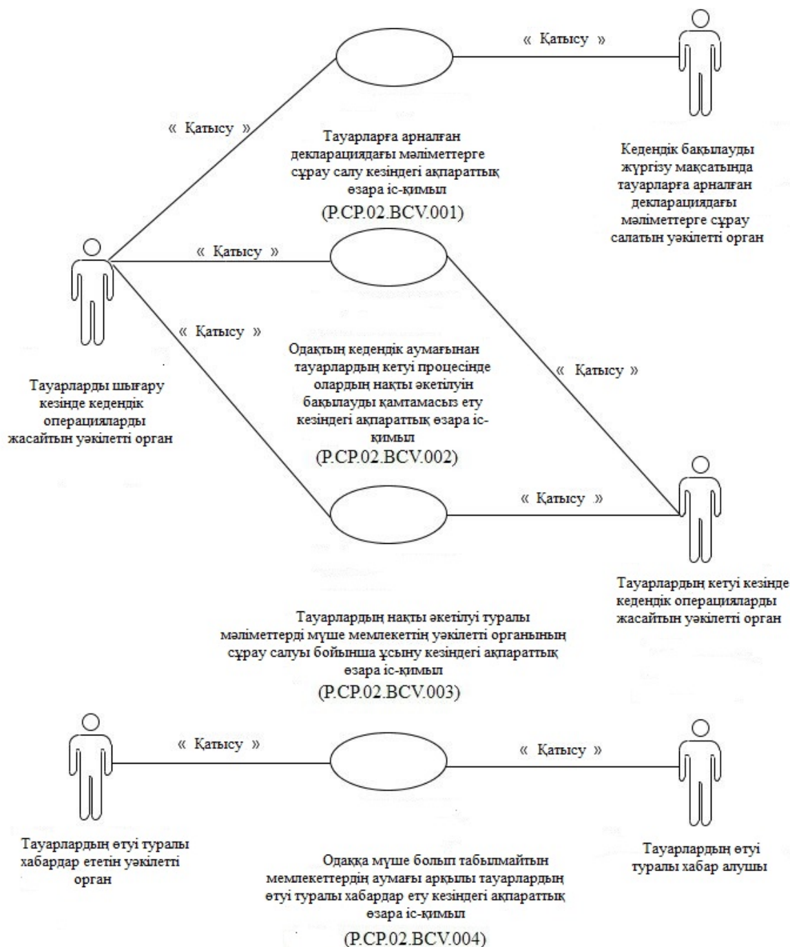
1-сурет. Мүше мемлекеттердің уәкілетті органдары арасындағы ақпараттық өзара іс-қимыл құрылымы
