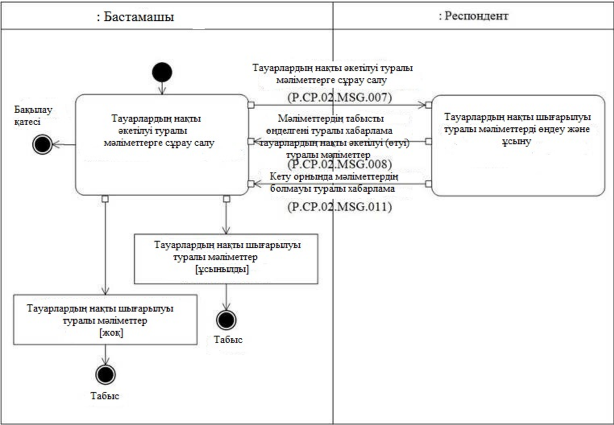
9-сурет. "Тауарлардың нақты әкетілуі туралы мәліметтерге сұрау салу" (P.CP.02. TRN.004) жалпы процесс транзакцияларын орындау схемасы 10-кесте
