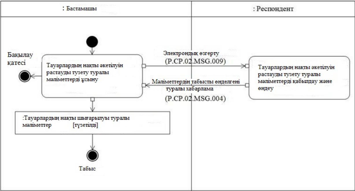
10-сурет. "Тауарлардың нақты әкетілуі туралы мәліметтерді түзету" (P.CP.02.TRN.005) жалпы процесс транзакцияларын орындау схемасы 11-кесте
