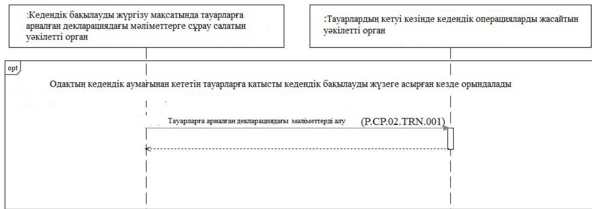
2-сурет. Тауарларға арналған декларациядағы мәліметтерге сұрау салу кезіндегі жалпы процесс транзакцияларын орындау схемасы 2-кесте
