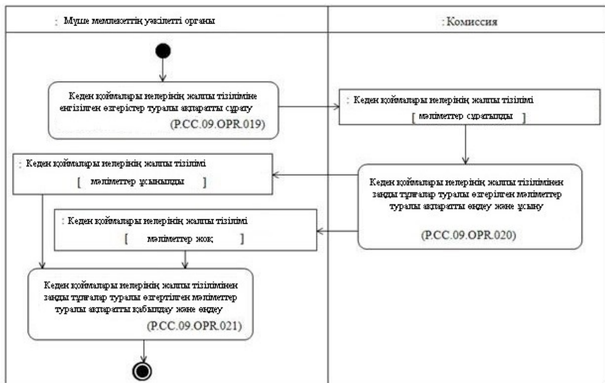
10-сурет. "Кеден қоймалары иелерінің жалпы тізіліміне енгізілген өзгерістер туралы ақпаратты алу" (P.CC.09.PRC.006) рәсімін орындау схемасы
