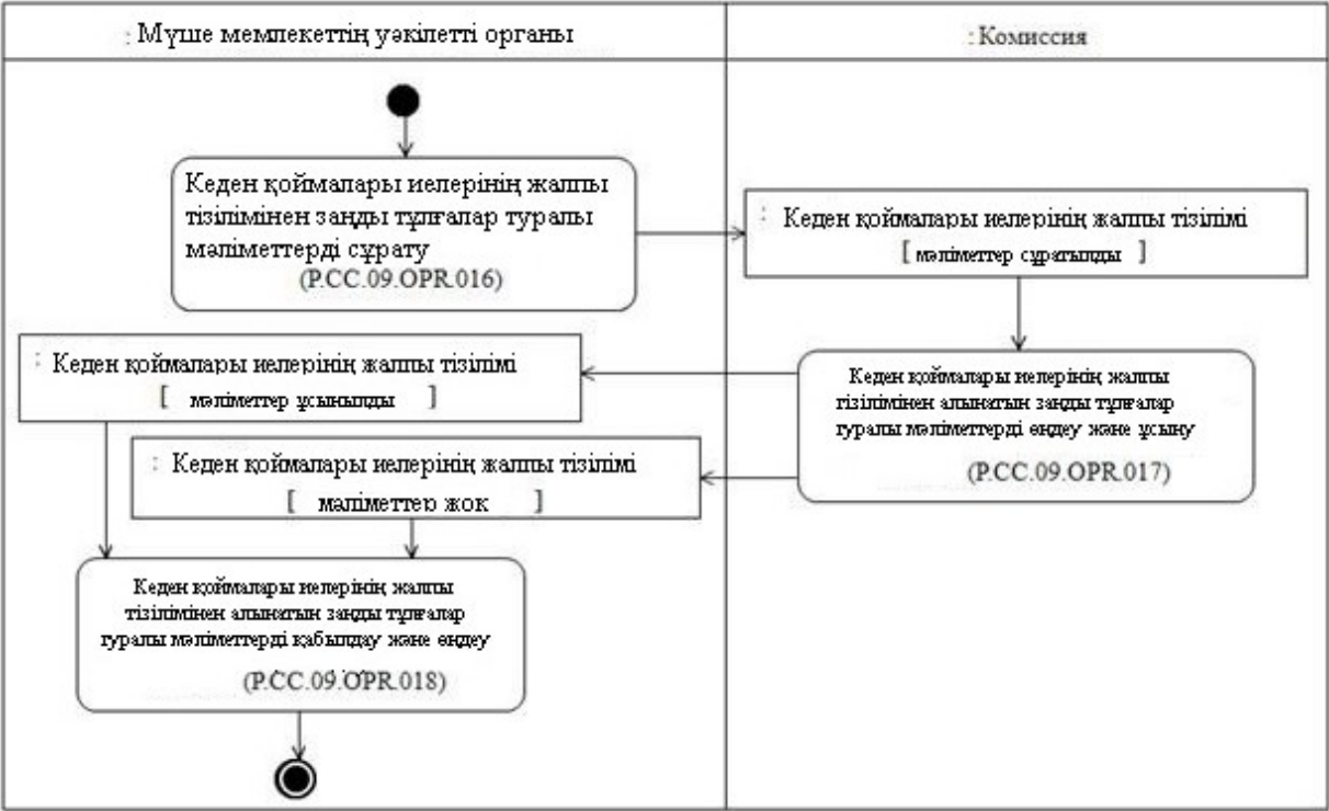
9-сурет. "Кеден қоймалары иелерінің жалпы тізілімінен заңды тұлғалар туралы мәліметтерді алу" (P.CC.09.PRC.005) рәсімін орындау схемасы
