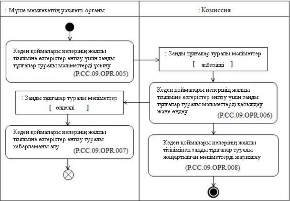
6-сурет. "Кеден қоймалары иелерінің жалпы тізілімінде қамтылған заңды тұлғалар туралы мәліметтерді өзгерту" (P.CC.09.PRC.002) рәсімін орындау схемасы
