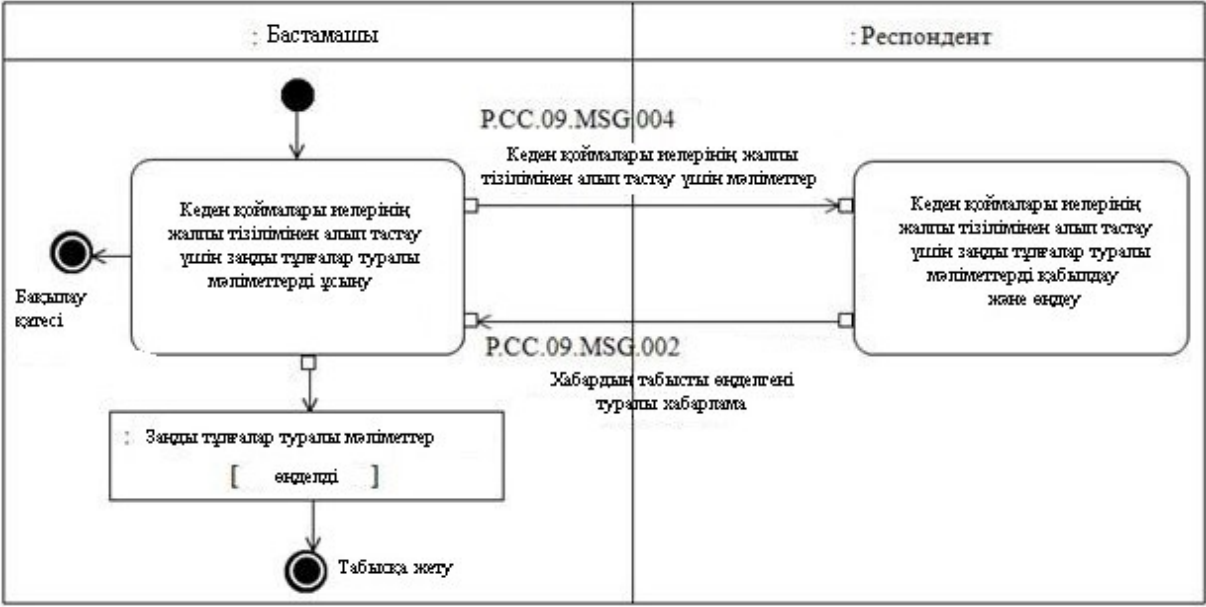
6-сурет. "Кеден қоймалары иелерінің жалпы тізілімінен заңды тұлғалар туралы мәліметтерді алып тастау" (P.CC.09.TRN.003) жалпы процесінің транзакциясын орындау схемасы 7-кесте
