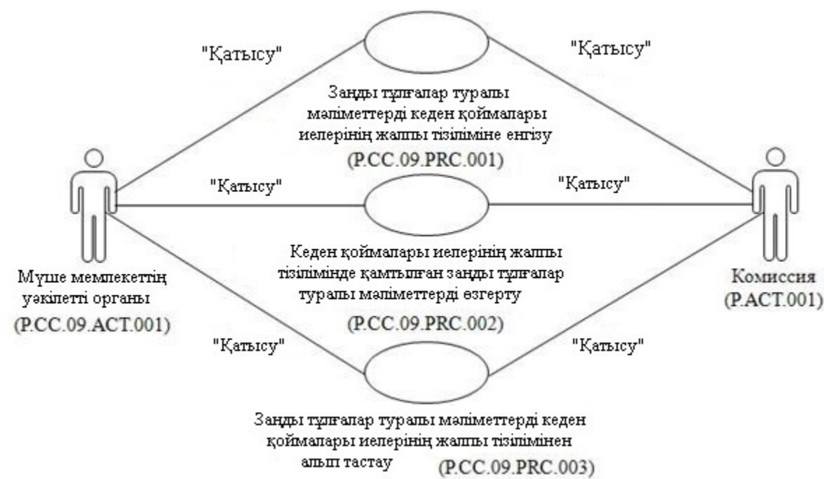
2-сурет. Кеден қоймалары иелерінің жалпы тізілімін қалыптастыру мен жүргізу рәсімдері тобының жалпы схемасы
