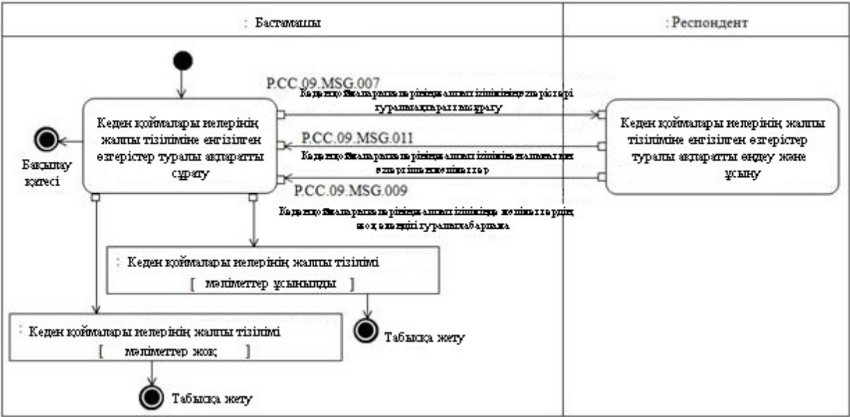
9-сурет. "Кеден қоймалары иелерінің жалпы тізіліміне енгізілген өзгерістер туралы ақпаратты алу" (P.CC.09.TRN.006) жалпы процесінің транзакциясын орындау схемасы 10-кесте
