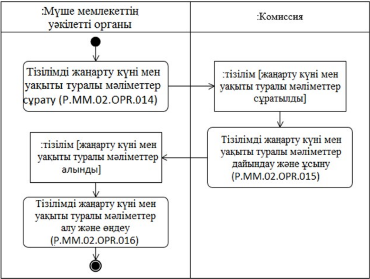
7-сурет. "Тізілімді жаңарту күні және уақыты туралы мәліметтер алу" (P.MM.02.PRC.004) рәсімін орындау схемасы
