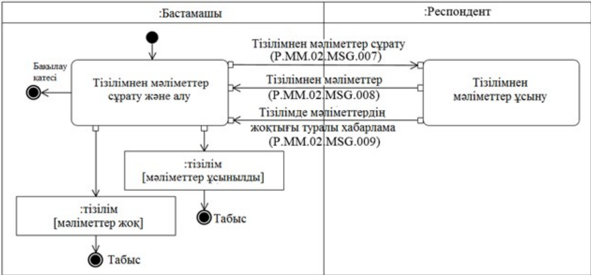
8-сурет. "Тізілімнен мәліметтер алу" (P.MM.02.TRN.005) жалпы процесінің транзакциясын орындау схемасы 9-кесте
