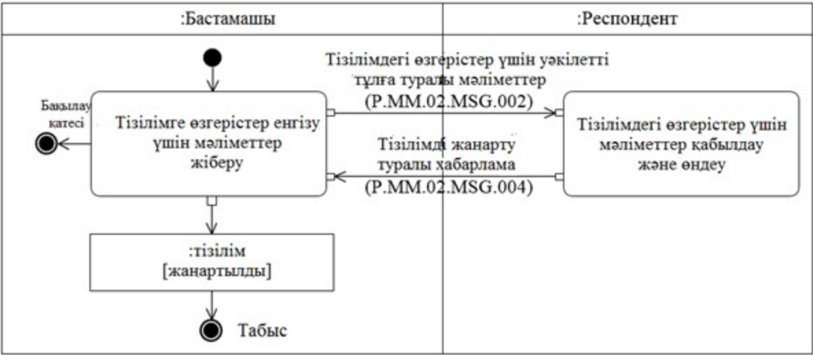
5-сурет. "Тізілімге енгізілетін өзгерістер үшін уәкілетті тұлға туралы мәліметтер беру" (P.MM.02.TRN.002) жалпы процесінің транзакциясын орындау схемасы 6-кесте
