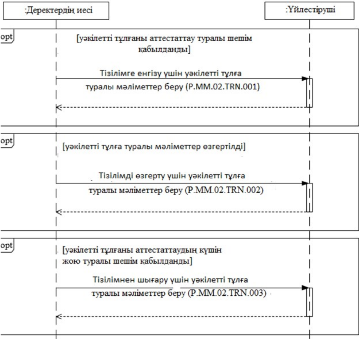
2-сурет. Тізілімді қалыптастыру және жүргізу кезінде жалпы процестің транзакцияларын орындау схемасы
