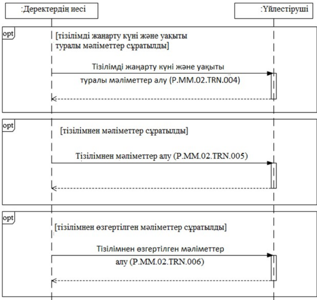
3-сурет. Тізілімнен мәліметтер алу кезінде жалпы процестің транзакцияларын орындау схемасы
