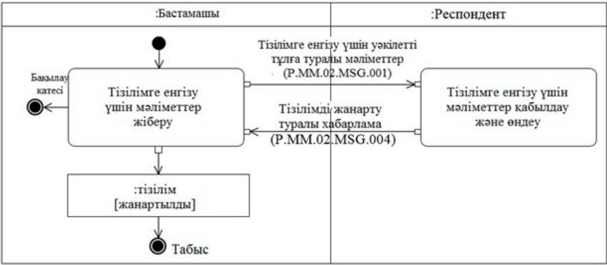
4-сурет. "Тізілімге енгізу үшін уәкілетті тұлға туралы мәліметтер беру" (P.MM.02.TRN.001) жалпы процесінің транзакциясын орындау схемасы
