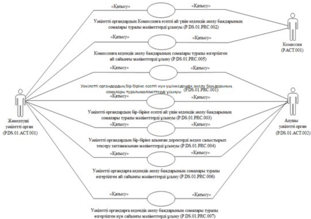
1-сурет. Жалпы процестің құрылымы
