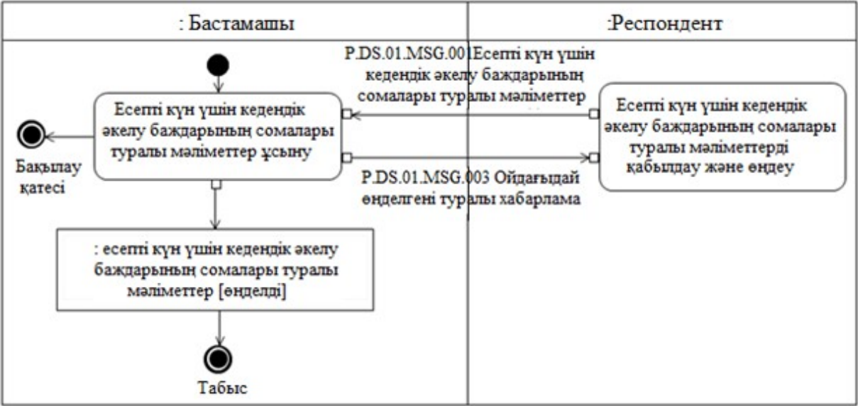
3-сурет. "Есепті күн үшін кедендік әкелу баждарының сомалары туралы мәліметтер ұсыну" (P.DS.01.TRN.001) жалпы процесс транзакциясын орындау схемасы 4-кесте
