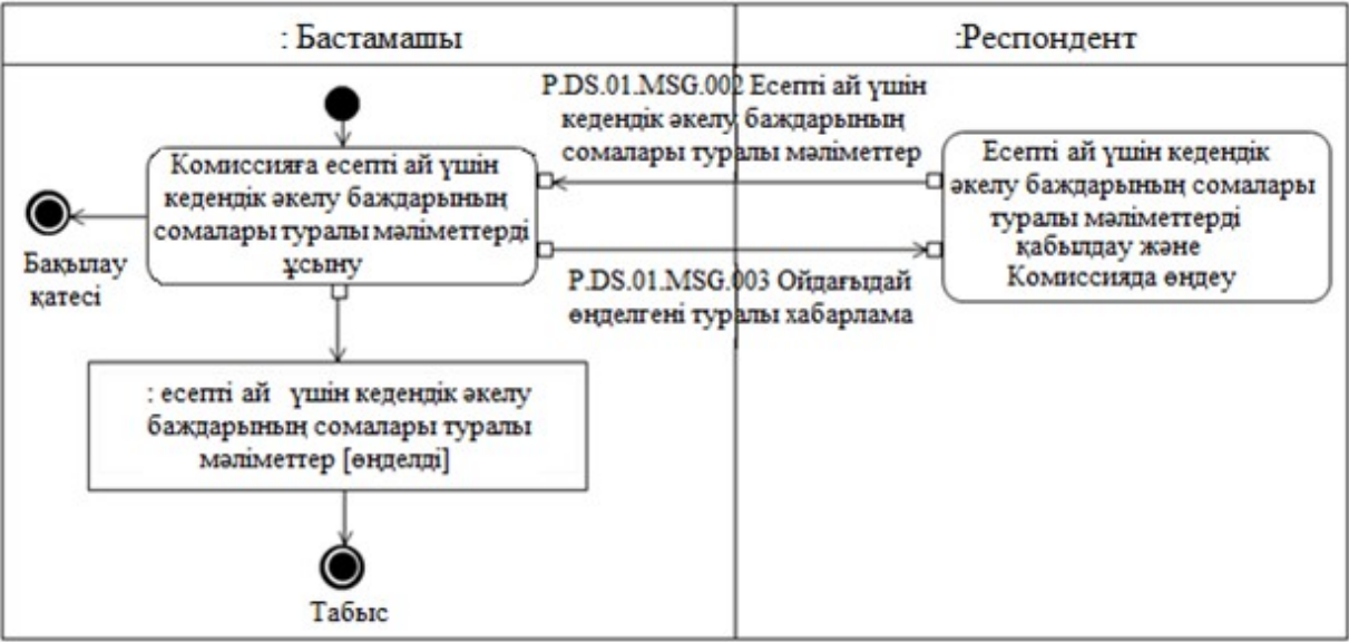
3-сурет. "Уәкілетті органдардың Комиссияға есепті ай үшін кедендік әкелу баждарының сомалары туралы мәліметтерді ұсынуы" (P.DS.01.TRN.003) жалпы процесс транзакциясын орындау схемасы
