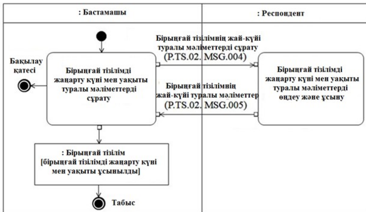
6-сурет. "Бірыңғай тізілімді жаңарту күні мен уақыты туралы мәліметтерді беру" ( P.TS.02.TRN.003) жалпы процесс транзакциясын орындау схемасы 7-кесте
