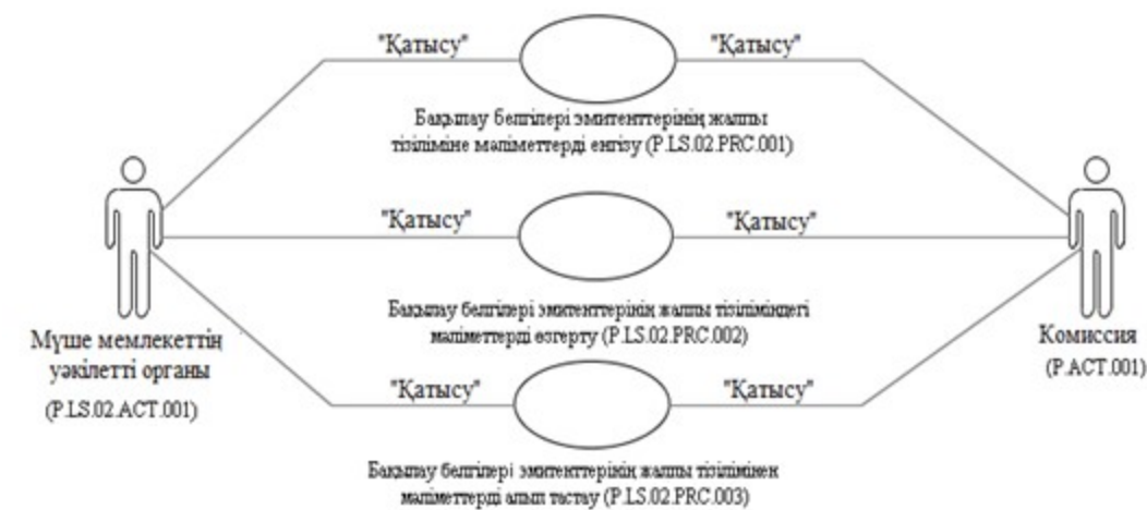
2-сурет. Бақылау белгілері эмитенттерінің жалпы тізілімін қалыптастыру және жүргізу рәсімдері тобының жалпы схемасы
