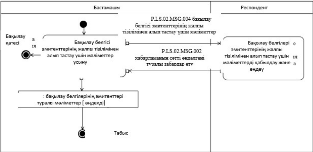
6-сурет. "Бақылау белгілері эмитенттері жалпы тізілімінен мәліметтерді алып тастау" жалпы процесс транзакциясын орындау схемасы (P.LS.02.TRN.003)
