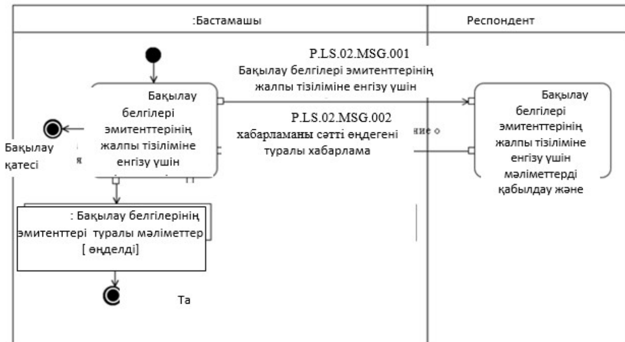
4-сурет. "Бақылау белгілері эмитенттерінің жалпы тізіліміне мәліметтер енгізу" ( P.LS.02.TRN.001) жалпы процесінің транзакциясын орындау схемасы 5-кесте
