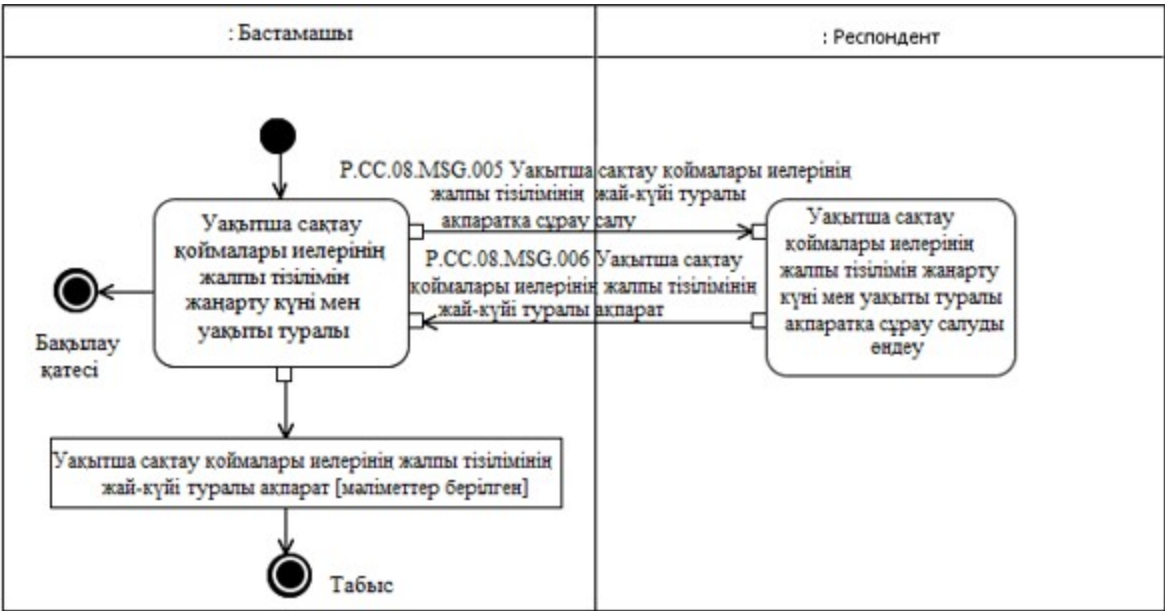
7-сурет. "Уақытша сақтау қоймалары иелерінің жалпы тізілімін жаңарту күні мен уақыты туралы ақпарат алу" (P.CC.08.TRN.004) жалпы процесс транзакциясының орындалу схемасы 8-кесте
